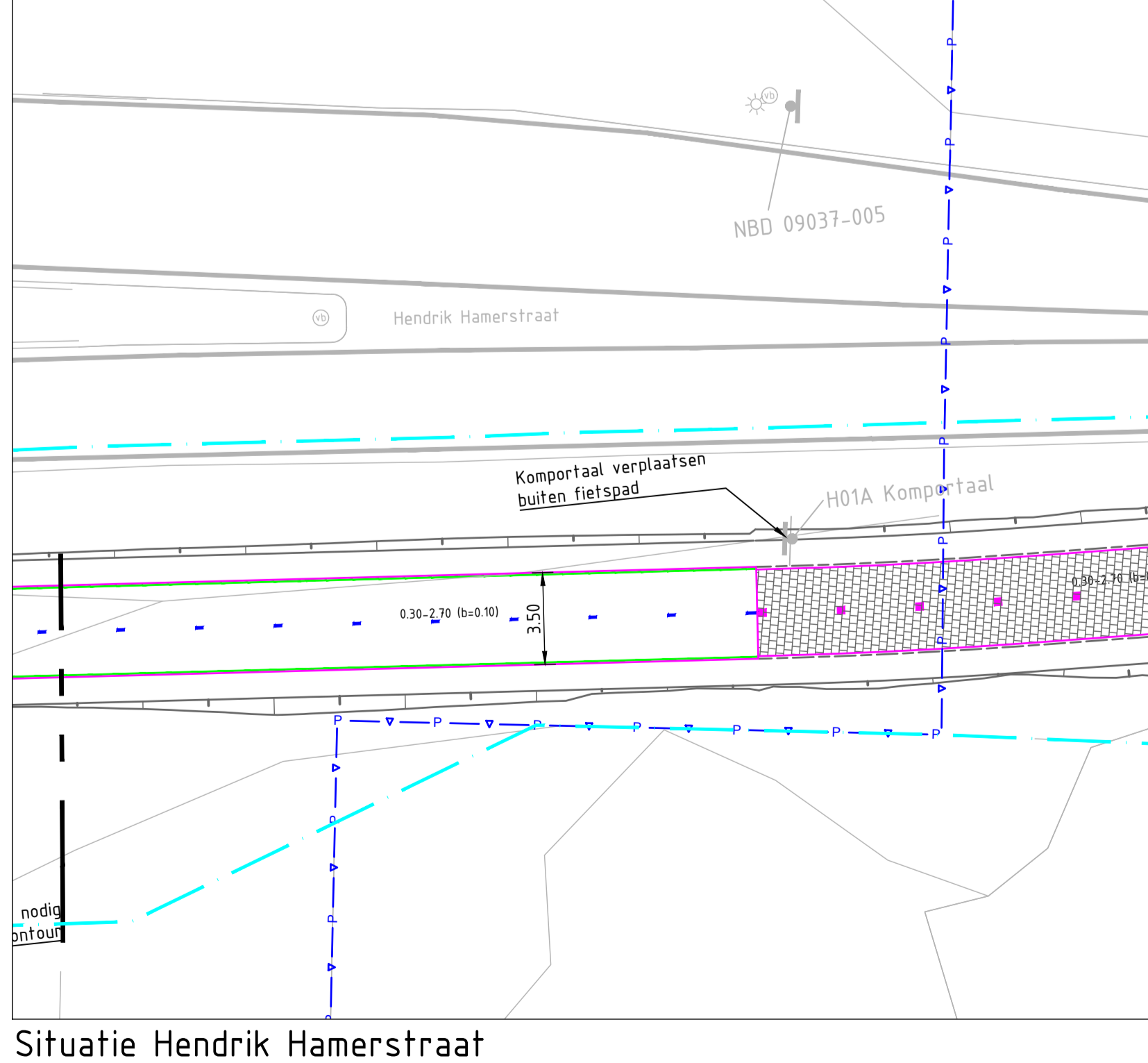
Situatie Hendrik Hamerstraat SCHAAL 1: 200
