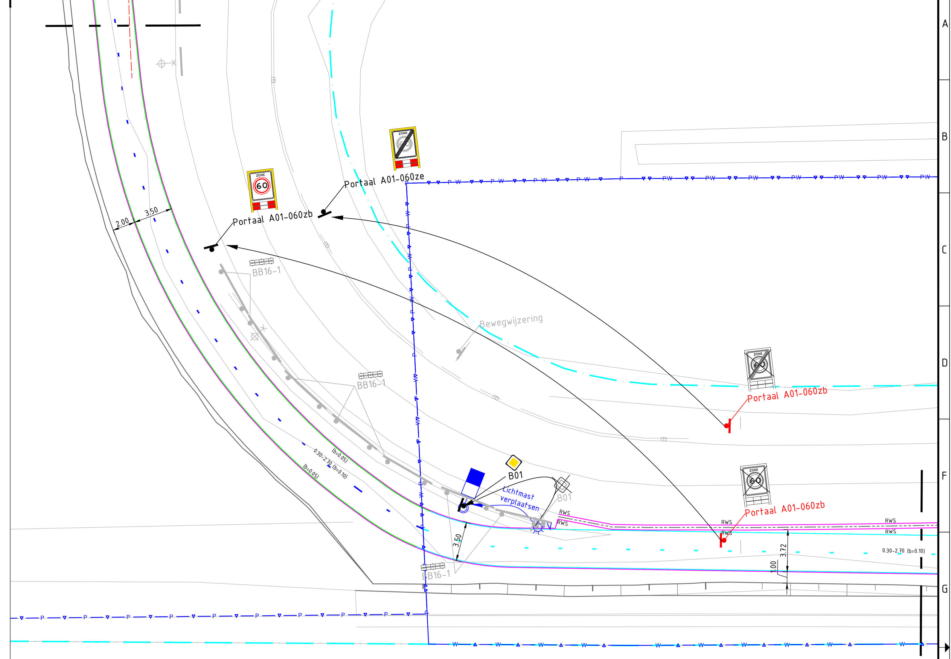
Situatie Havelaar SCHAAL 1: 200
