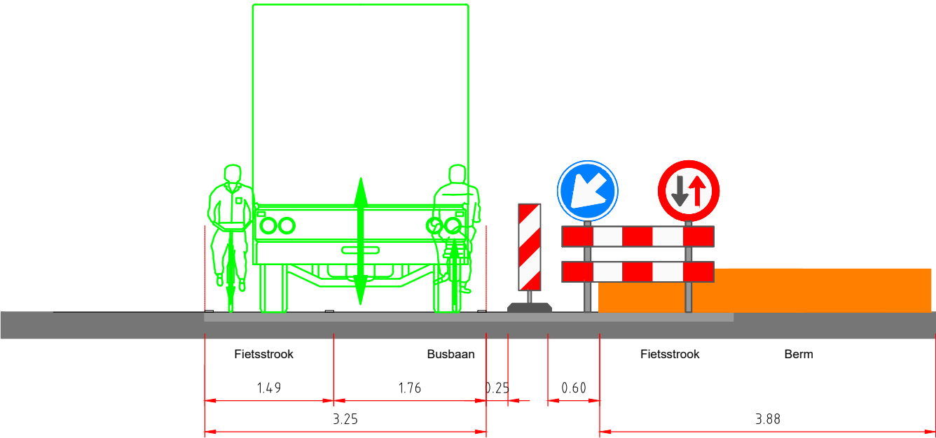
Dwarsprofiel A-A CROW 96b - tabel 2 Verkeersruimte bij twee rijstroken met verkeer in twee richtingen met fietsers
