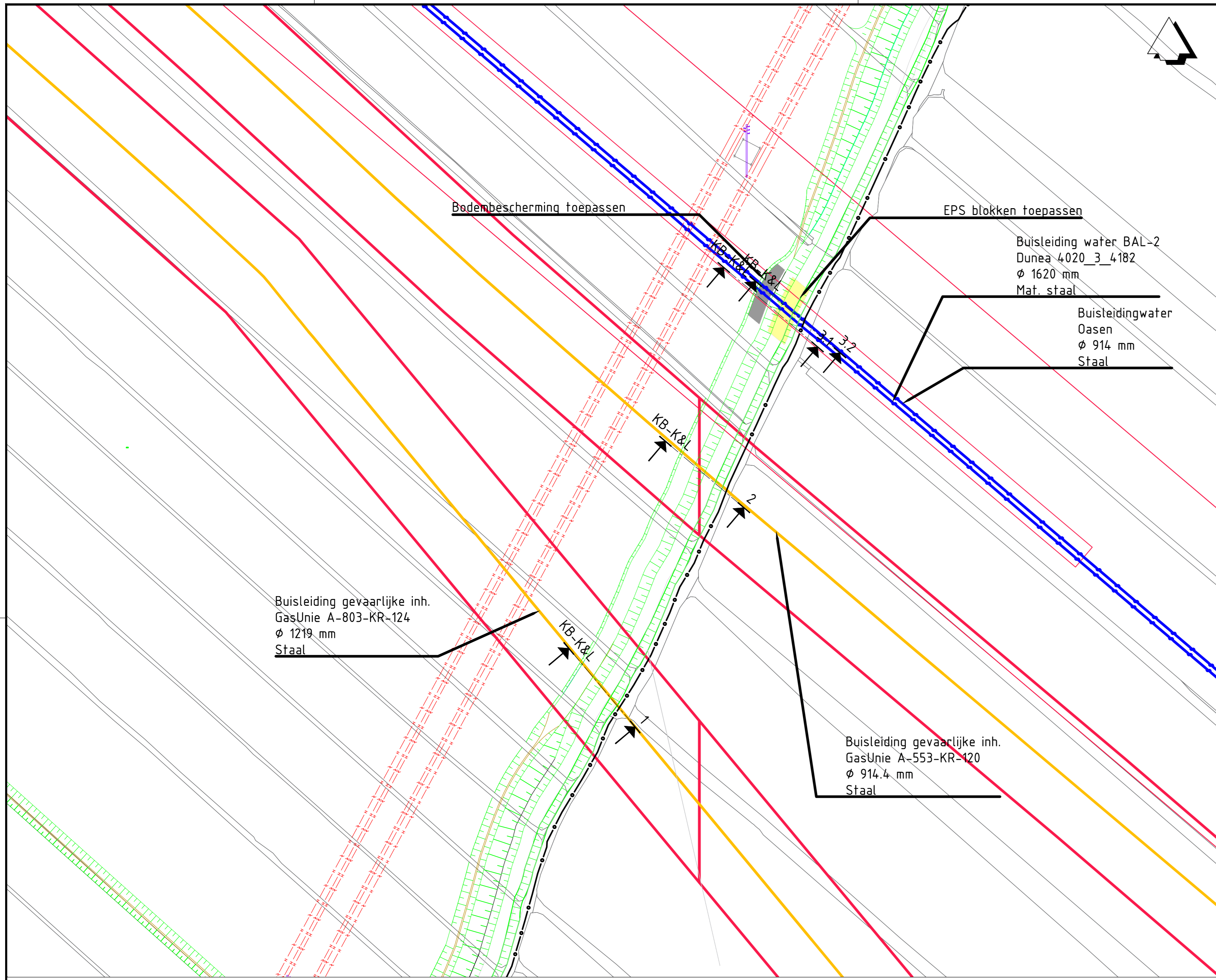
Locaties dwarsprofielen 1 SCHAAL 1:1000
