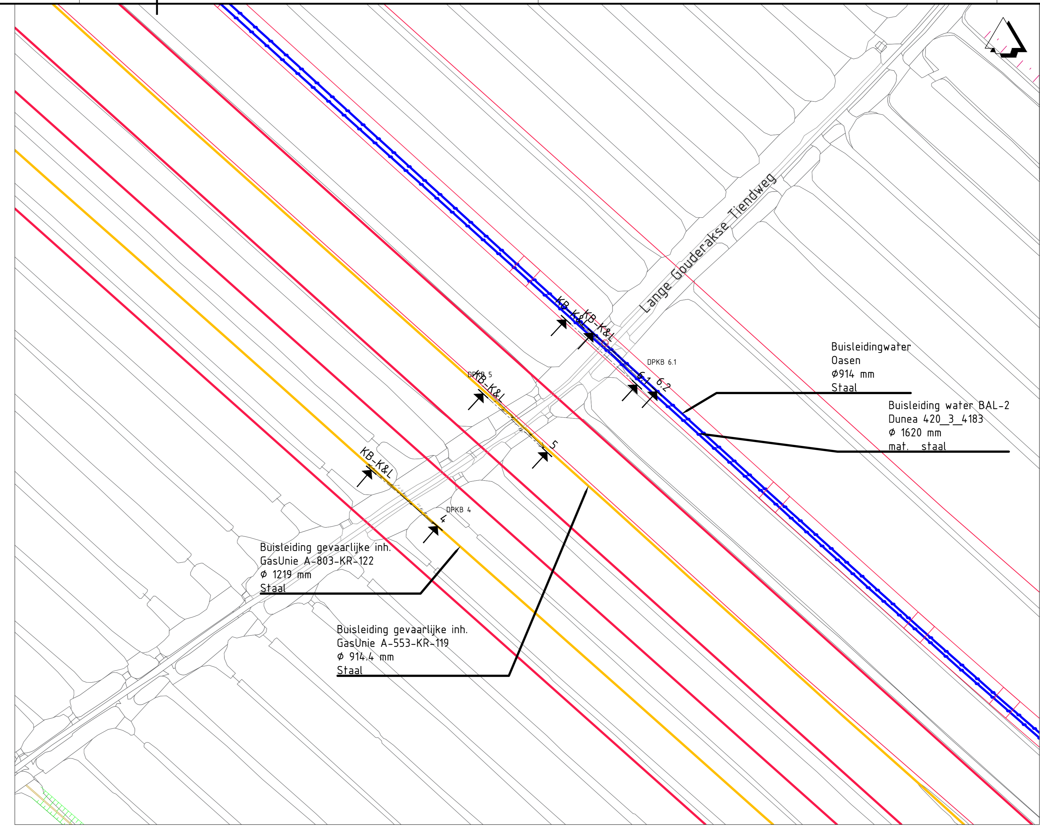
Locaties dwarsprofielen 2 SCHAAL 1:1000
