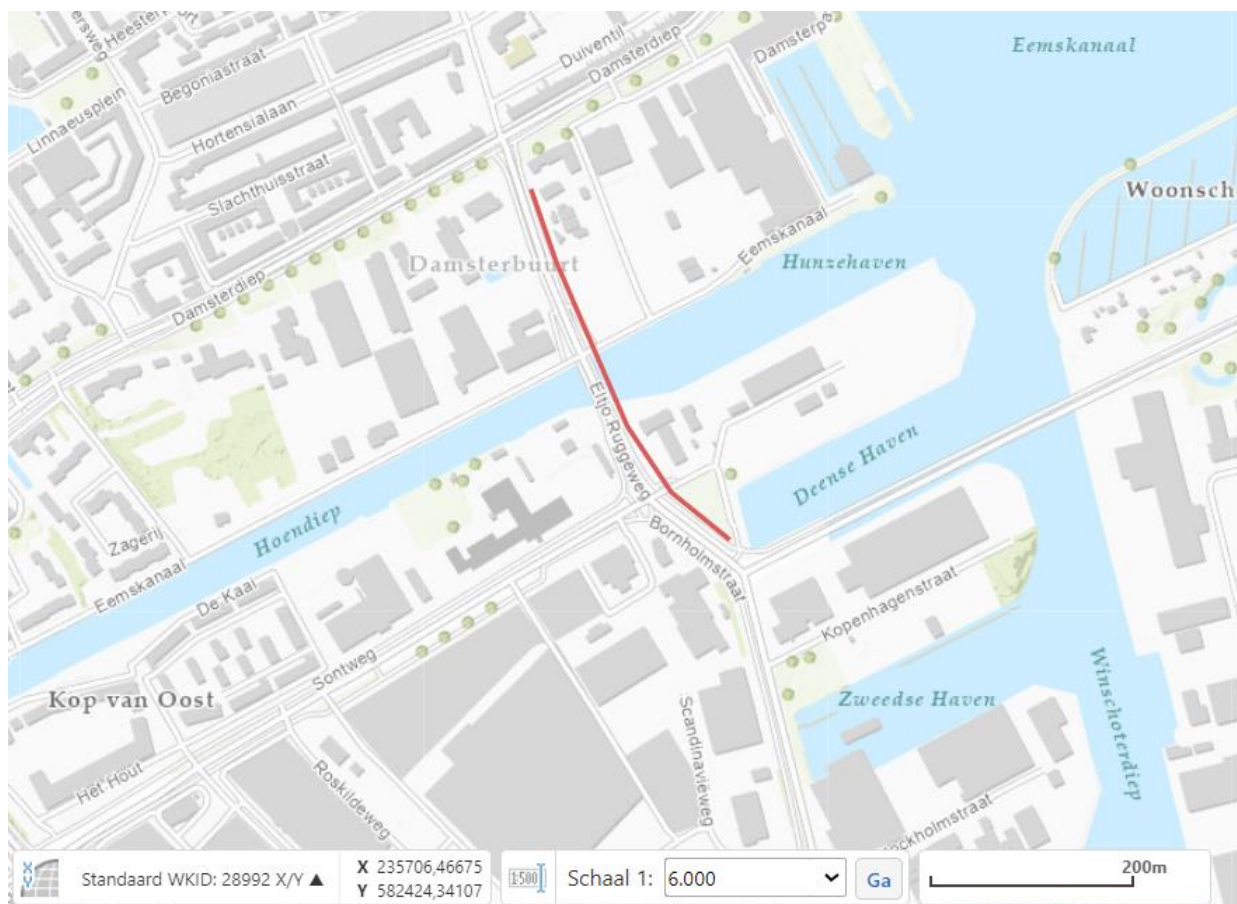
Figuur 1: De rode lijn geeft globaal de locatie weer van de aan te leggen leiding en de te maken gestuurde boring.
