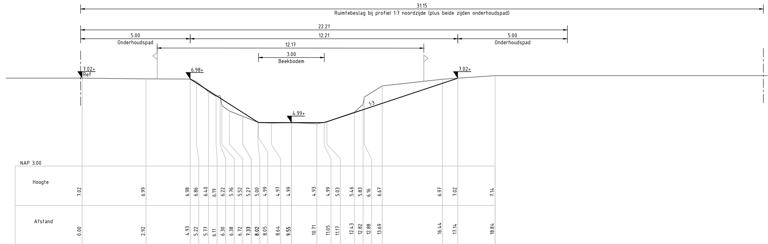
Principe profiel Biezenloop Schaal 1:100
