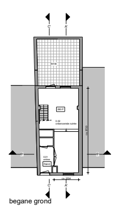
begane grond
