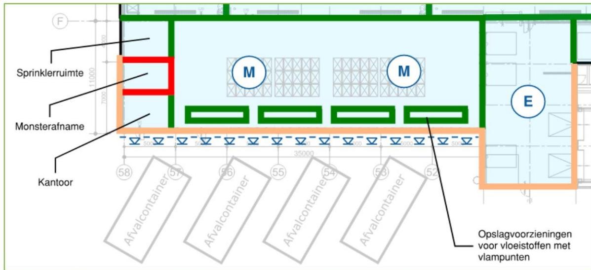
Figuur 1 Brandwerende maatregelen Hal M (groen= 60 min. | rood= 120 min. | oranje= niet brandbaar)
