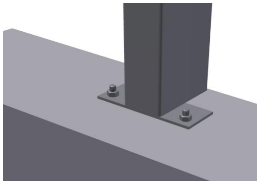
Afbeelding 5 Detail voetplaat
