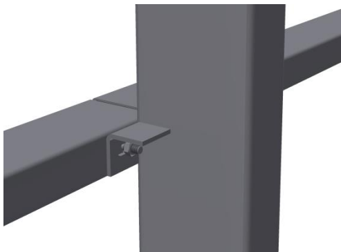
Afbeelding 4 Detail gording hoekje
