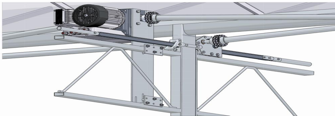
Afbeelding 10 Deatil overzicht luchtmechaniek
