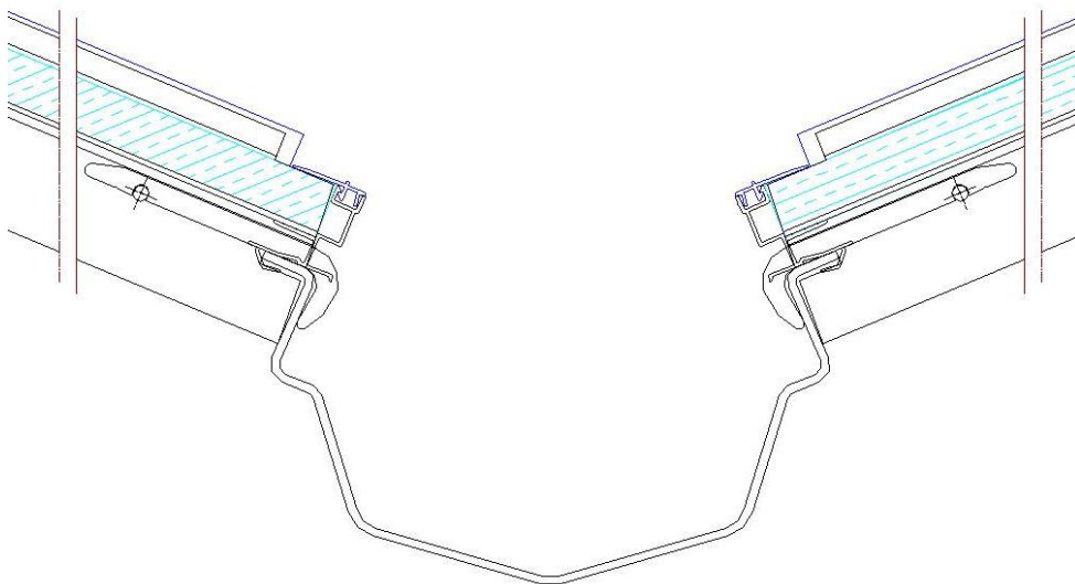
Afbeelding 7 stalen goot
