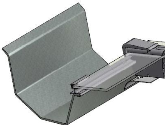
Afbeelding 6 stalen goot
