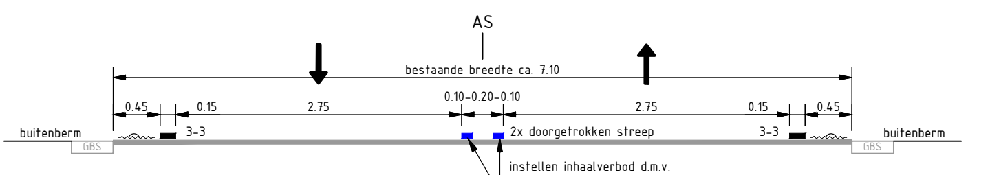
Principedoorsnede GOW (1x2) schaal 1:50
