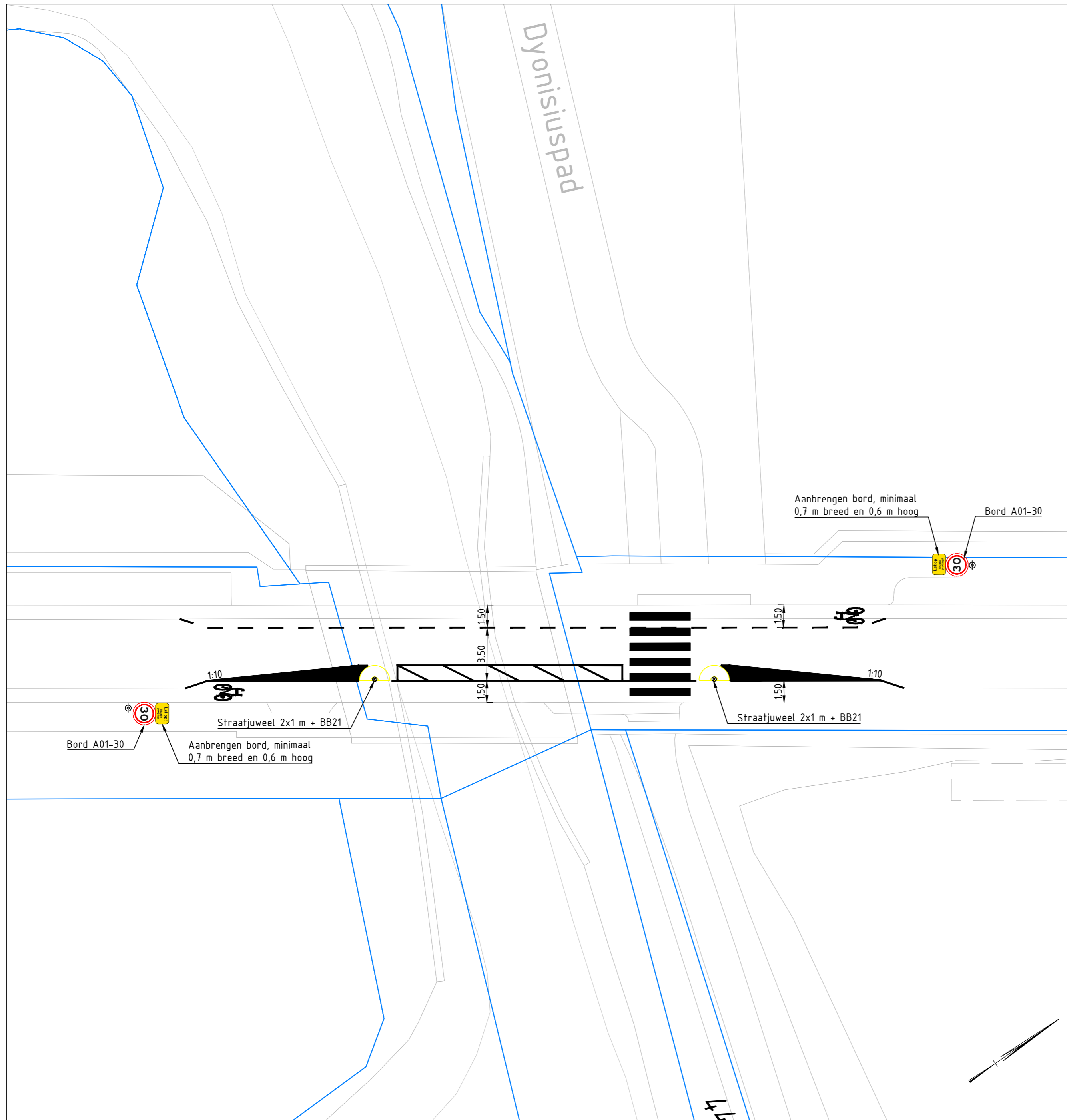
Situatie Schaal 1 : 200
