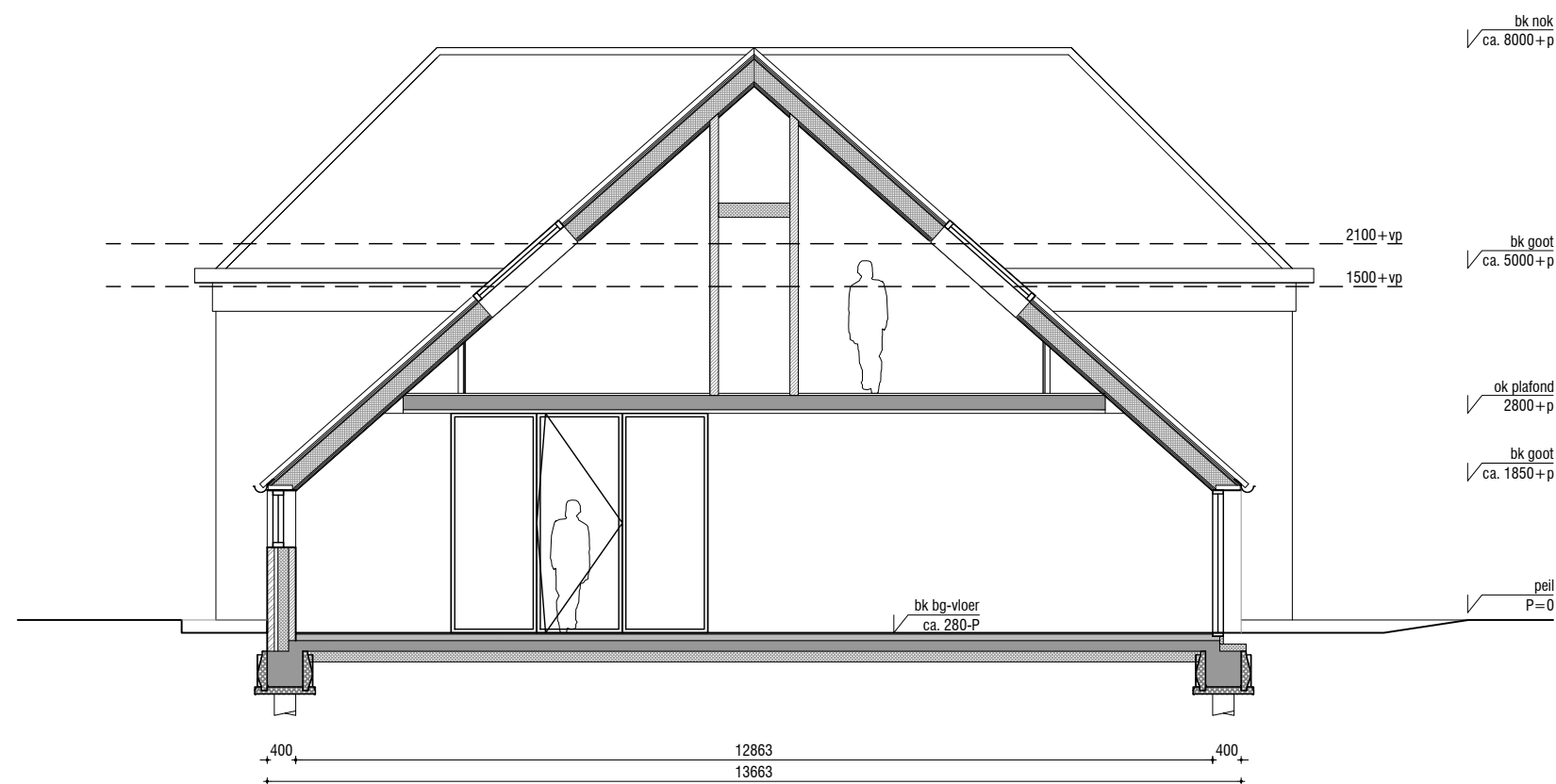
dwarsdoorsnede
