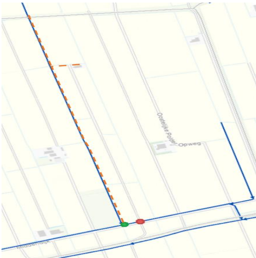
Figuur 1: De groene cirkel geeft globaal de locatie weer van de aan te leggen dam met duiker, de rode cirkel de te verwijderen brug, de nieuwe positie van het kavelpad is weergegeven met de oranje stippellijn.
