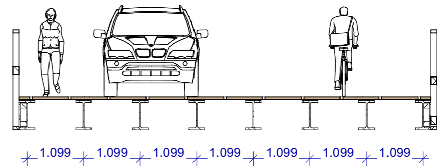
Doorsnede C-C
