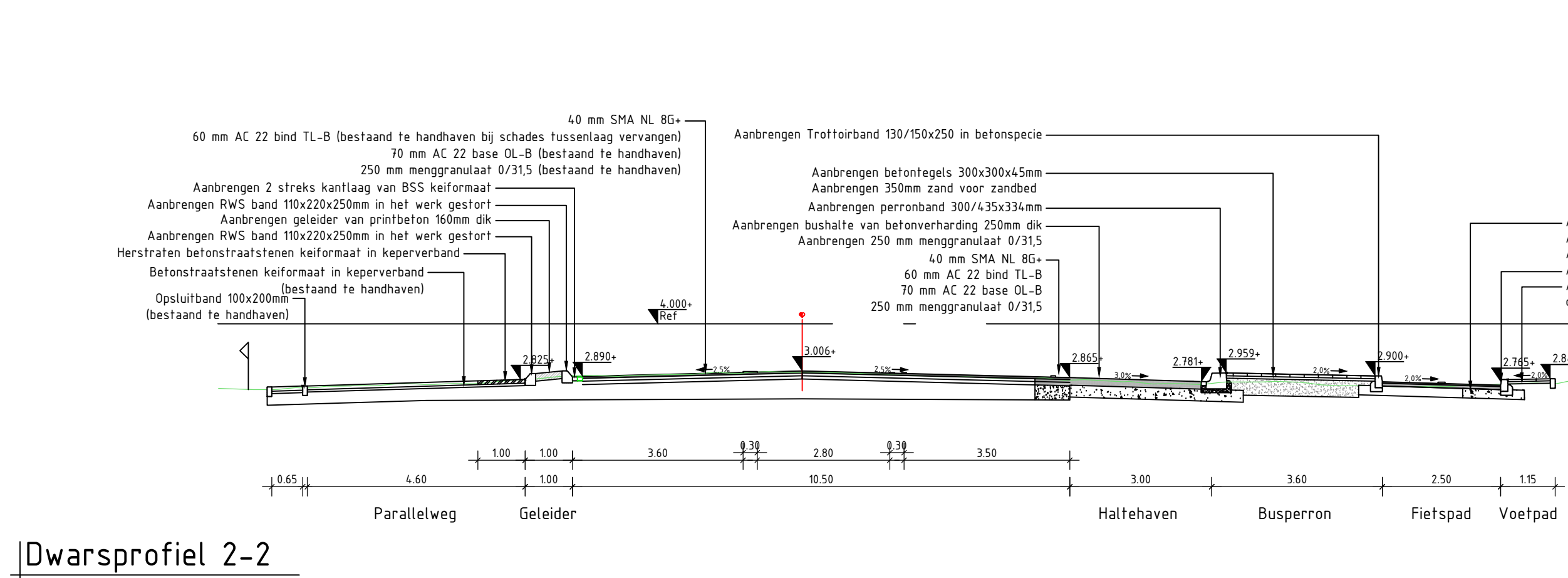
Dwarsprofiel 2-2 [Schaal 1:100 (rijrichting west)]
