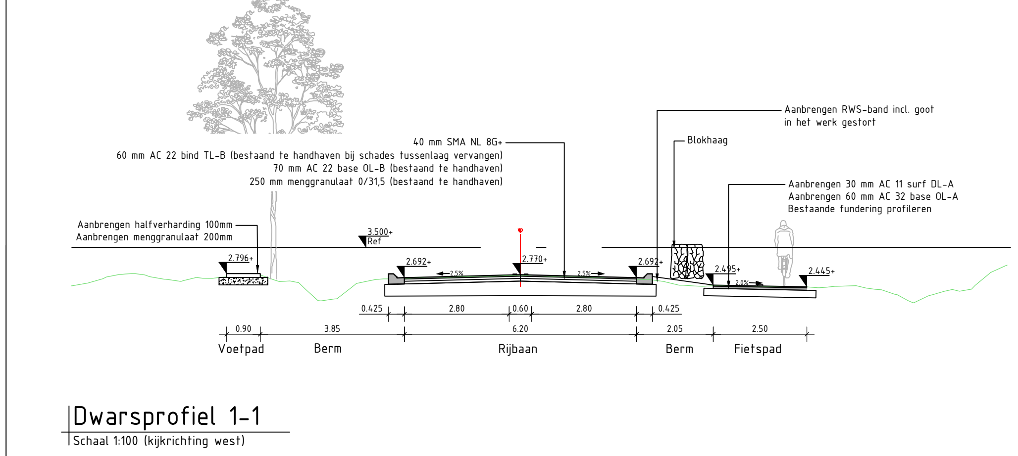
Dwarsprofiel 1-1 [Schaal 1:100 (rijrichting west)]
