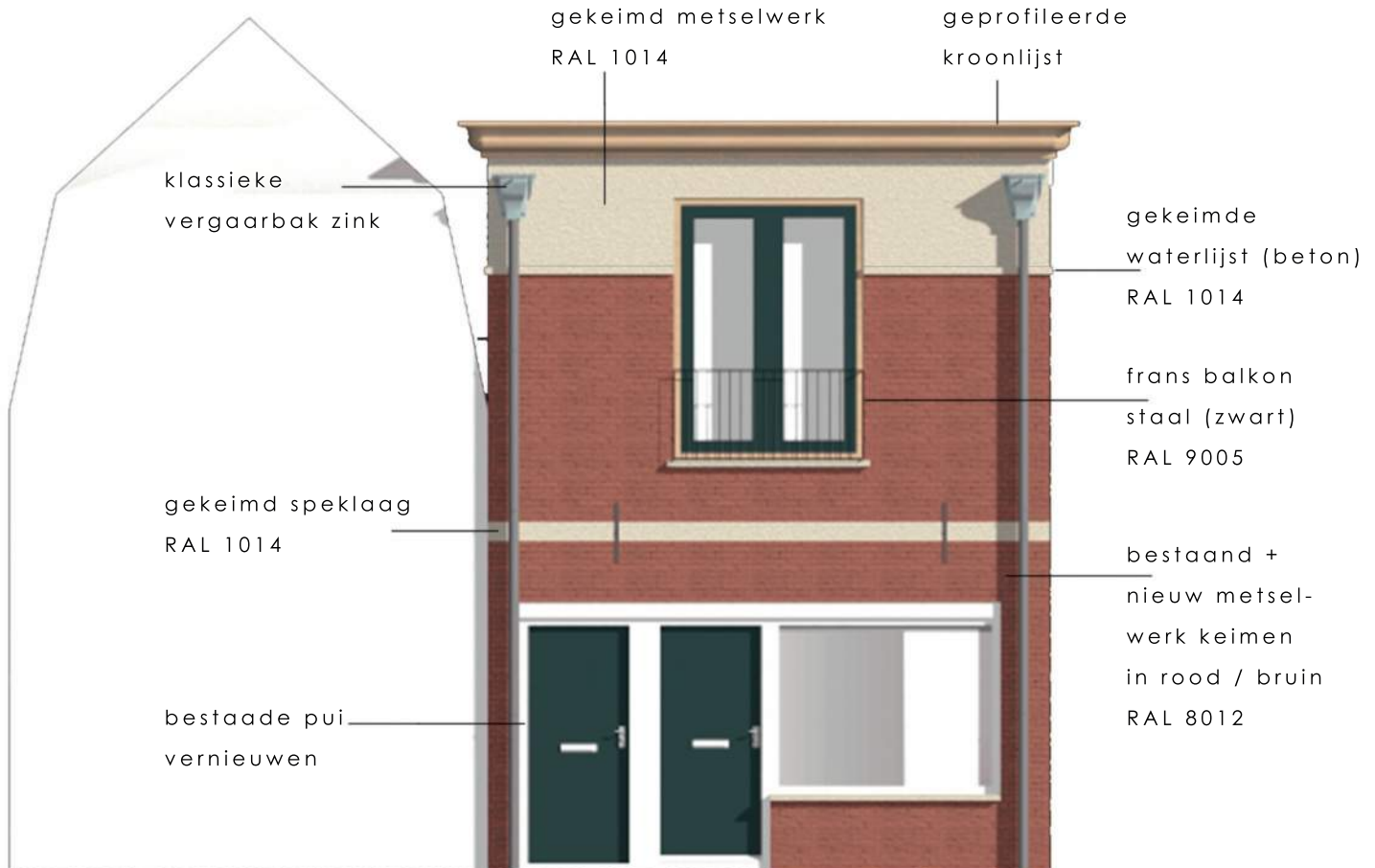
voorgevel nieuwe toestand
