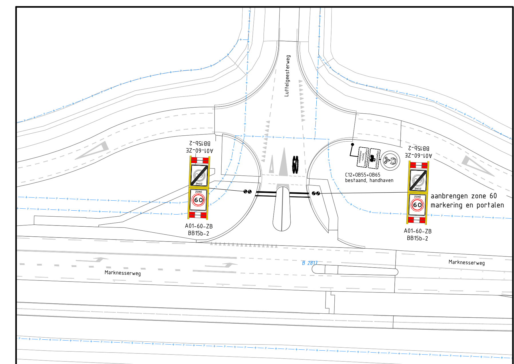
Detail C schaal 1500
