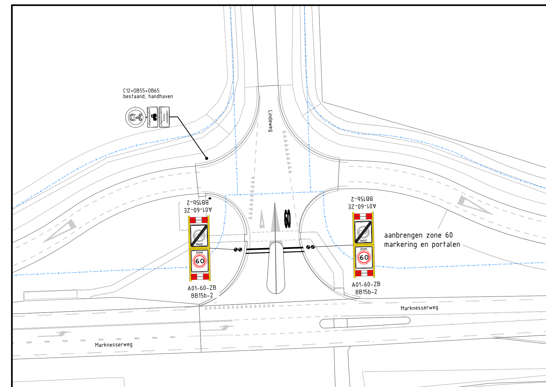
Detail B schaal 1500
