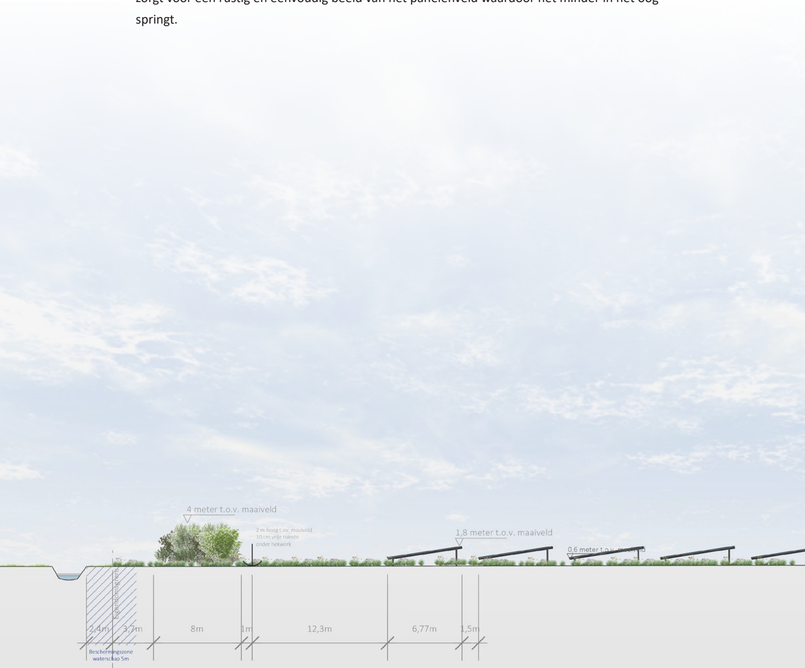
Afbeelding 12. Doorsnede D van zonneveld Kanaaldijk-Zuid met links de nieuwe landschappelijke haag en rechts het bestaande struweel met bomenrij.
