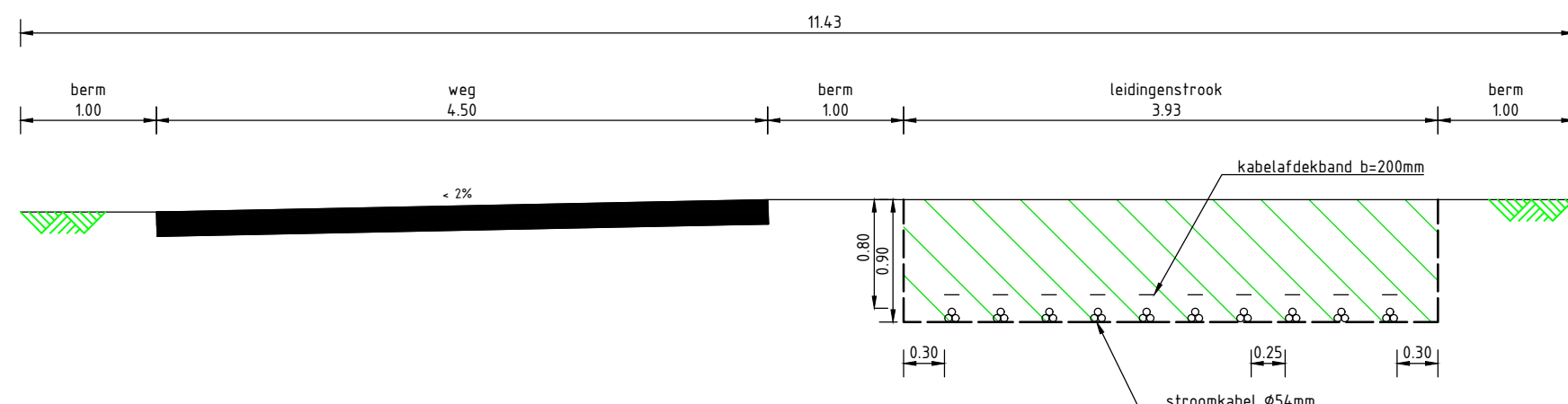
Detail B-B - Kabel- en leidingentracé Enexis
