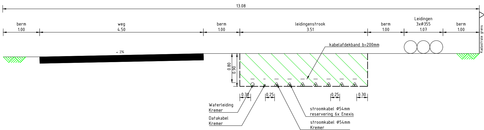
Detail A-A - Kabel- en leidingentracé Kremer en Enexis
