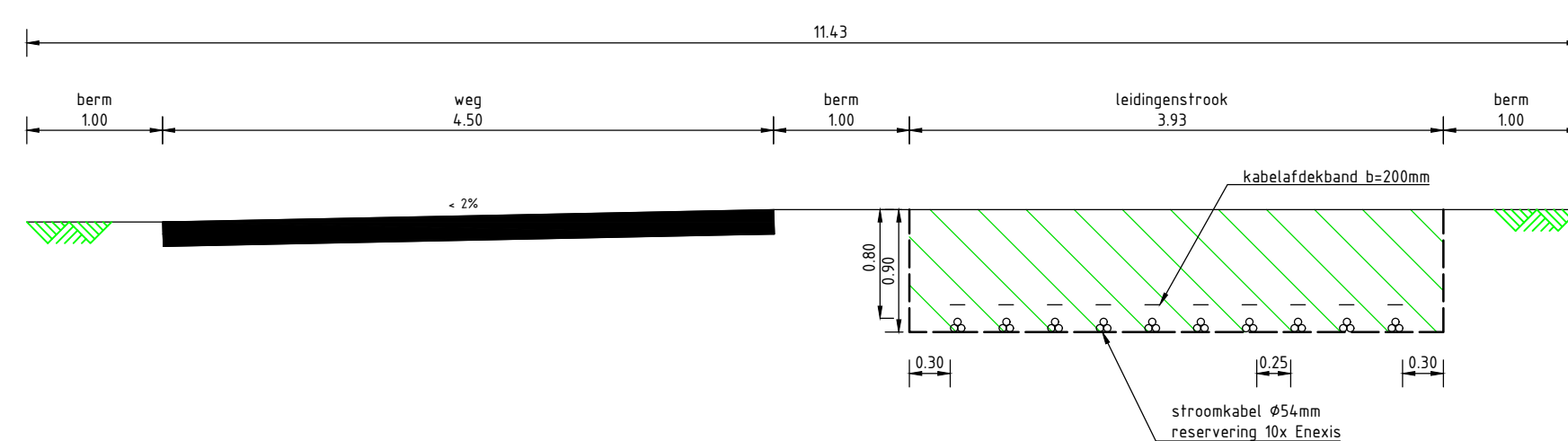
Detail B-B - Kabel- en leidingentracé Enexis
