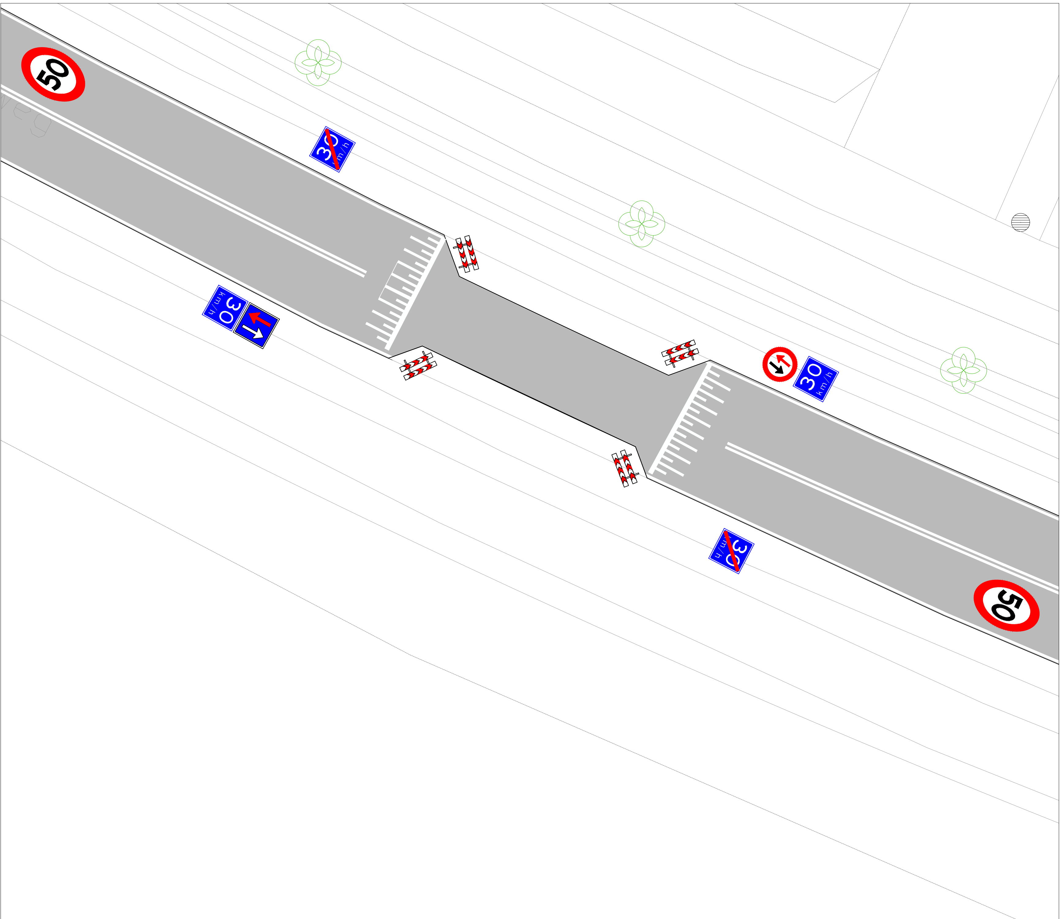
DETAIL D Schaal 1:100
