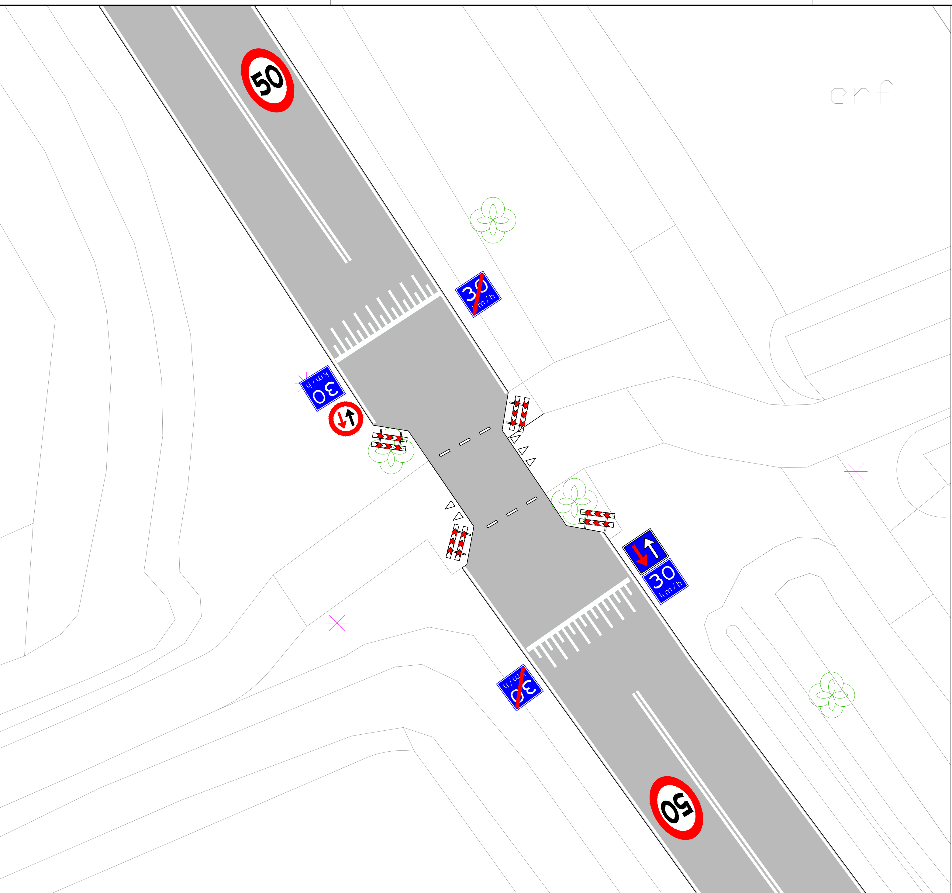
DETAIL B Schaal 1:100
