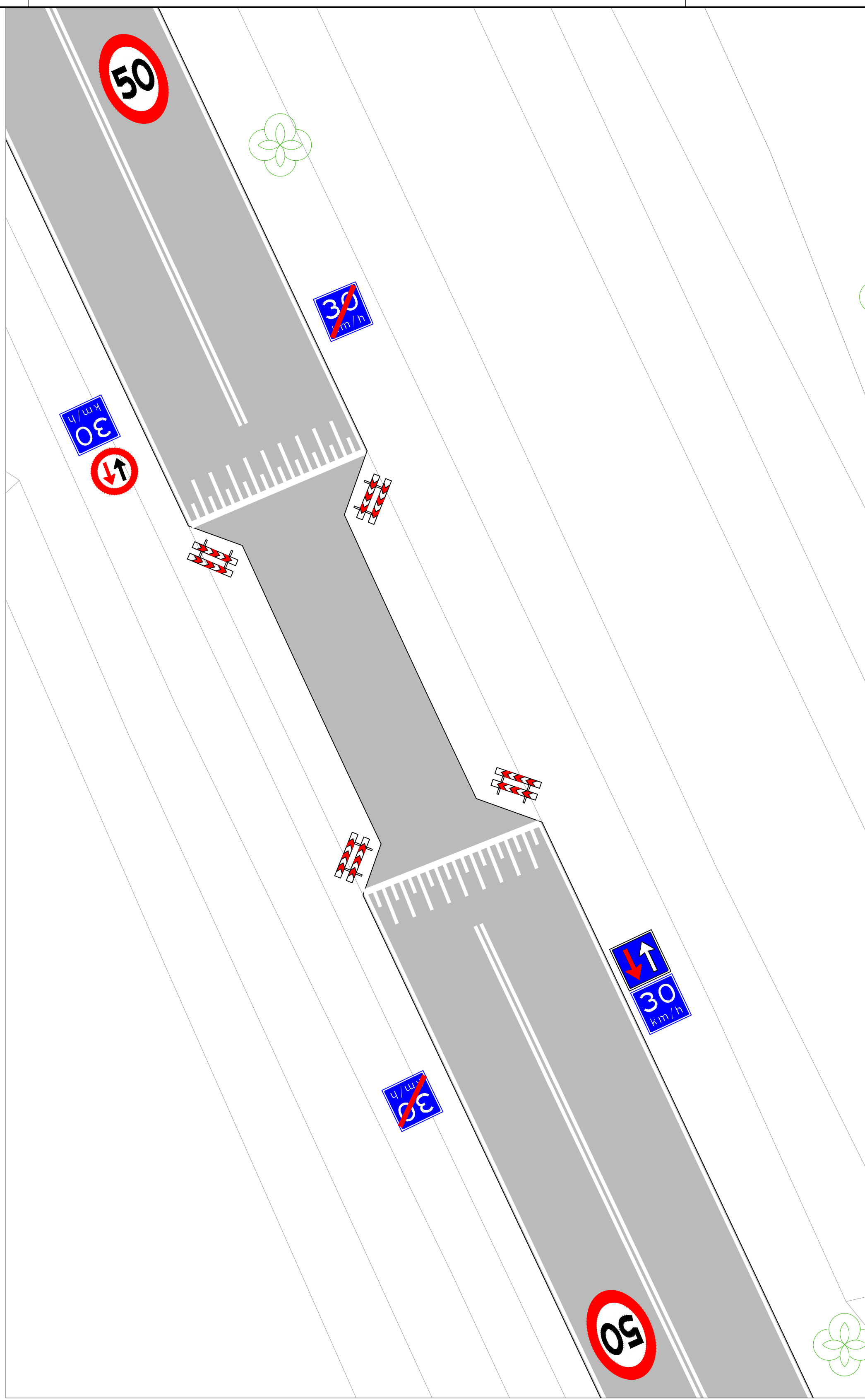
DETAIL A Schaal 1:100
