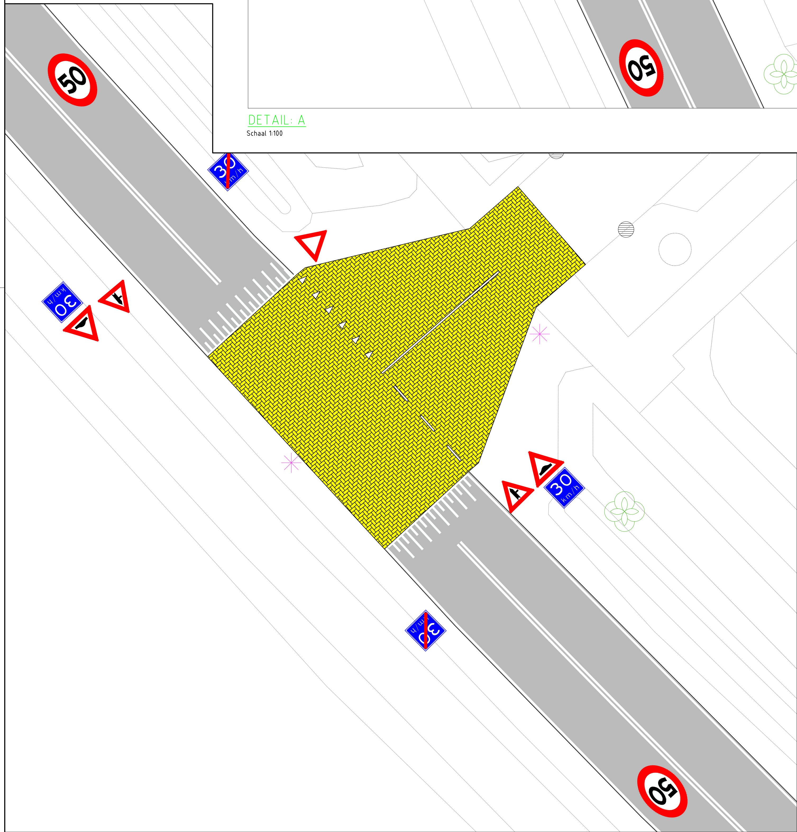
DETAIL C Schaal 1:100
