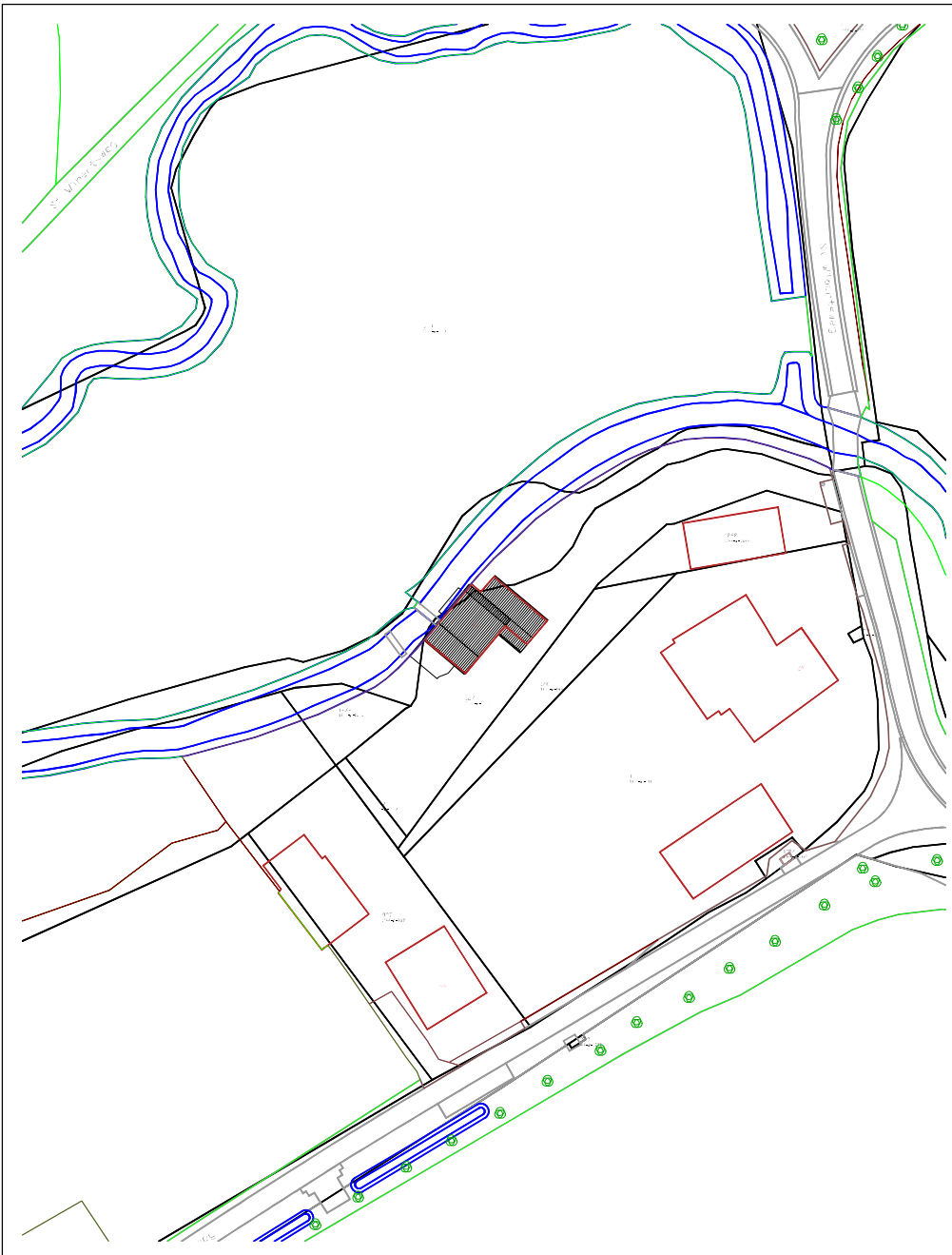
SITUATIE BESTAAND
