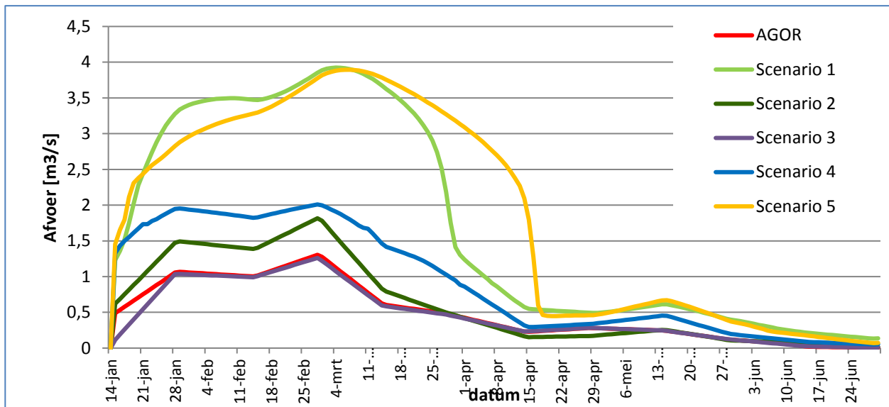
Figuur 9: Verandering afvoerloosheid ten gevolge van de scenario's (bovenstrooms van Medler).
