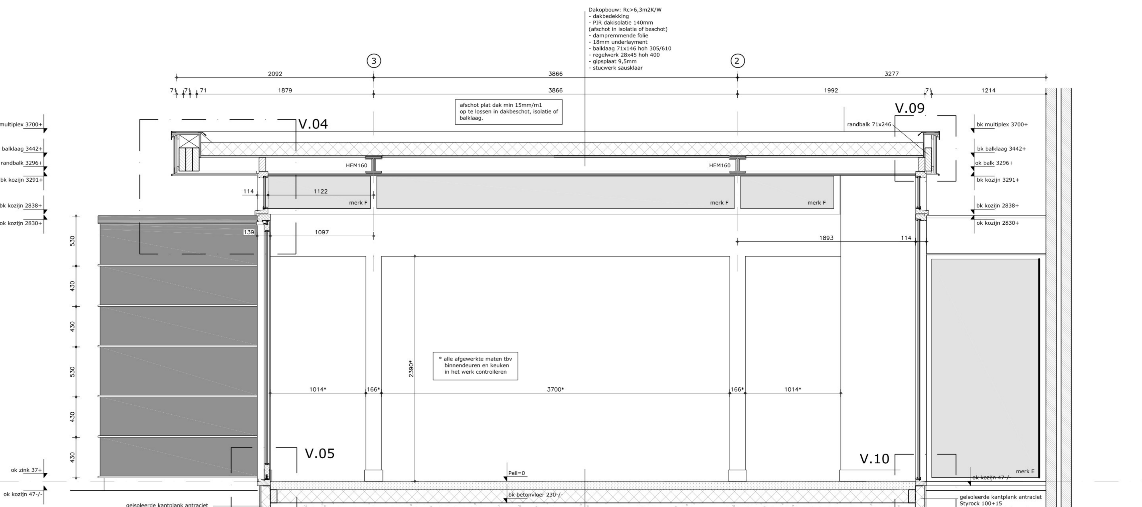
Doorsnede D-D
