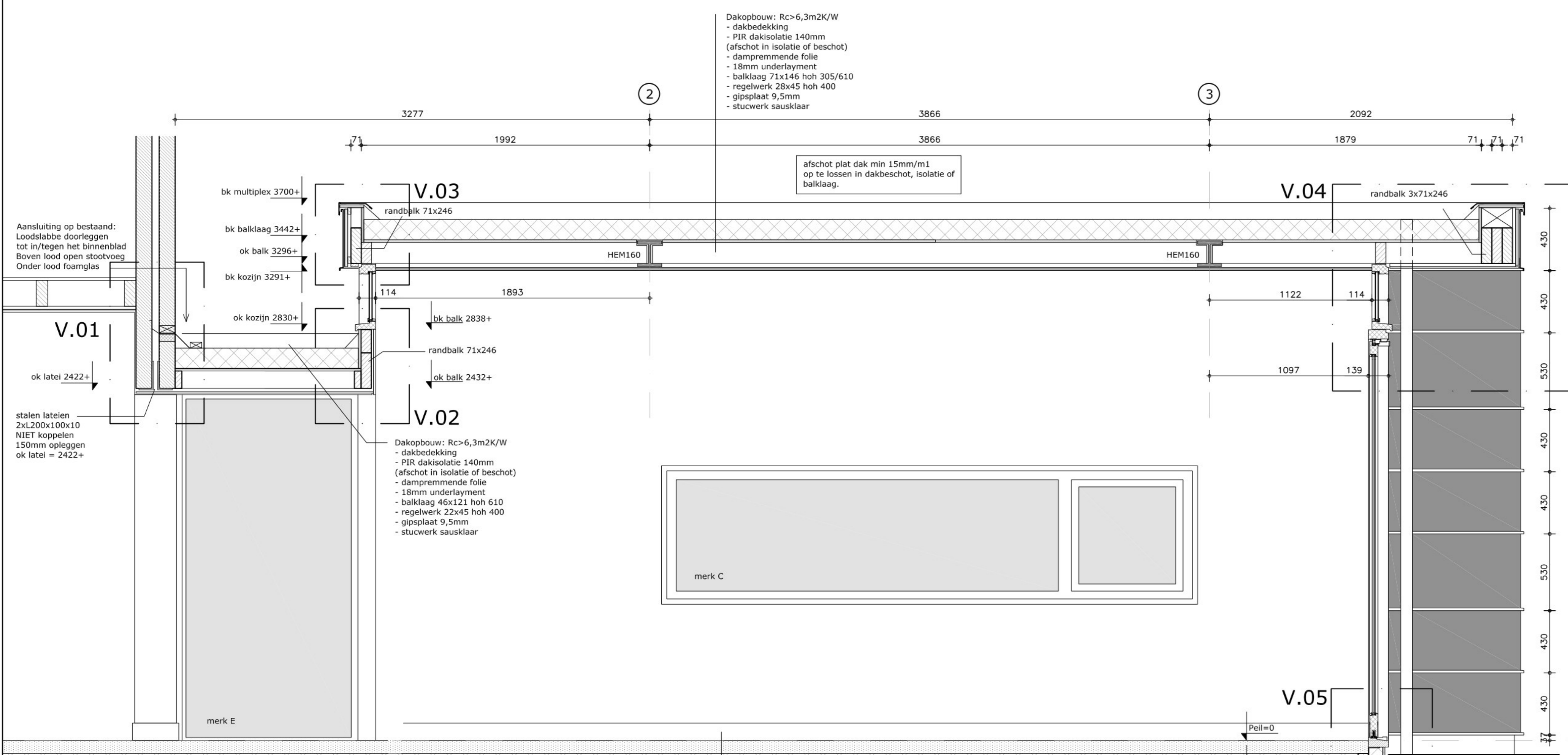
Doorsnede A-A
