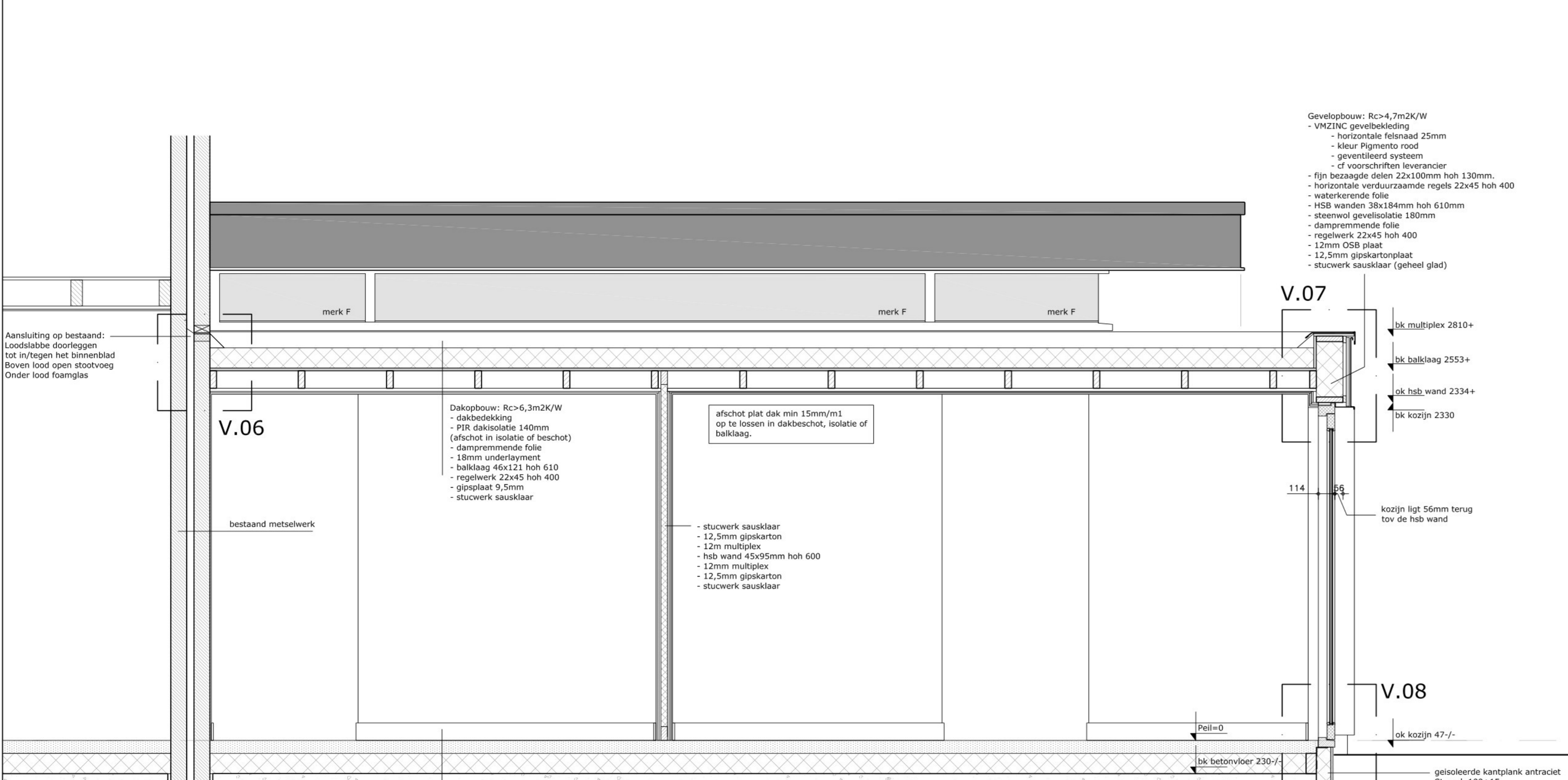
Doorsnede C-C
