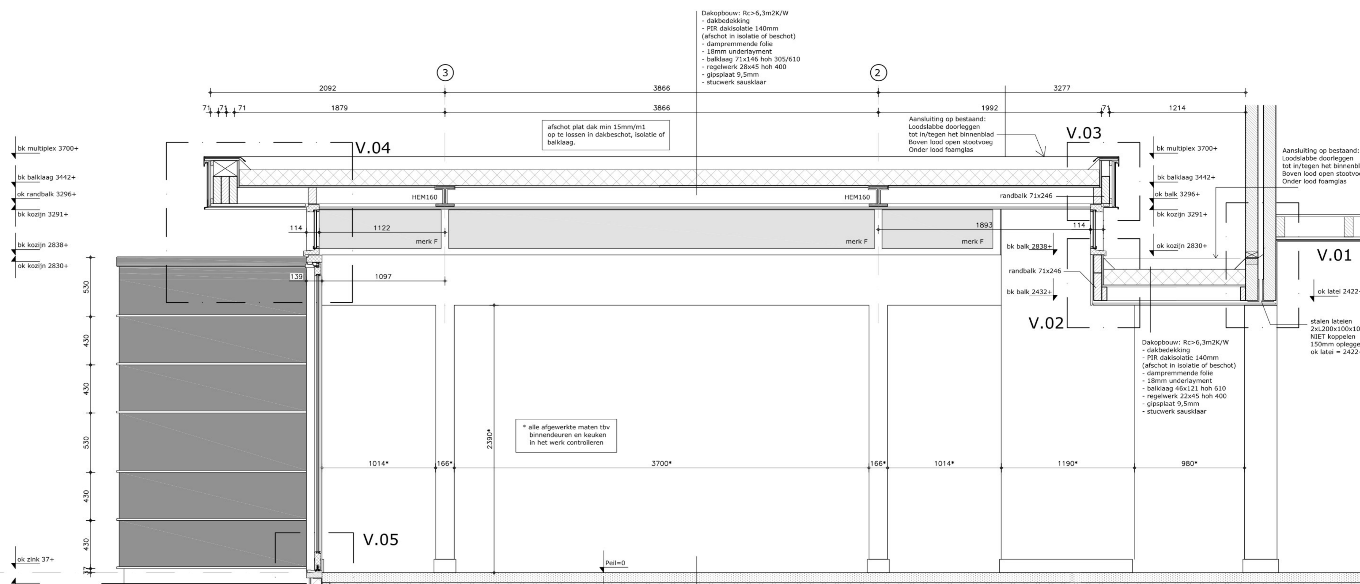
Doorsnede B-B
