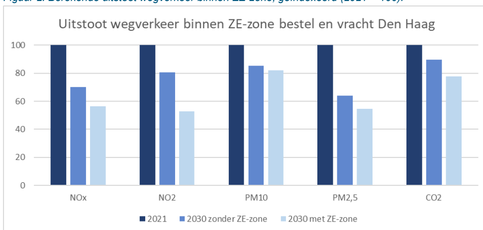
Figuur 2. Berekende uitstoot wegverkeer binnen ZE-zone, geïndexeerd (2021 = 100).
