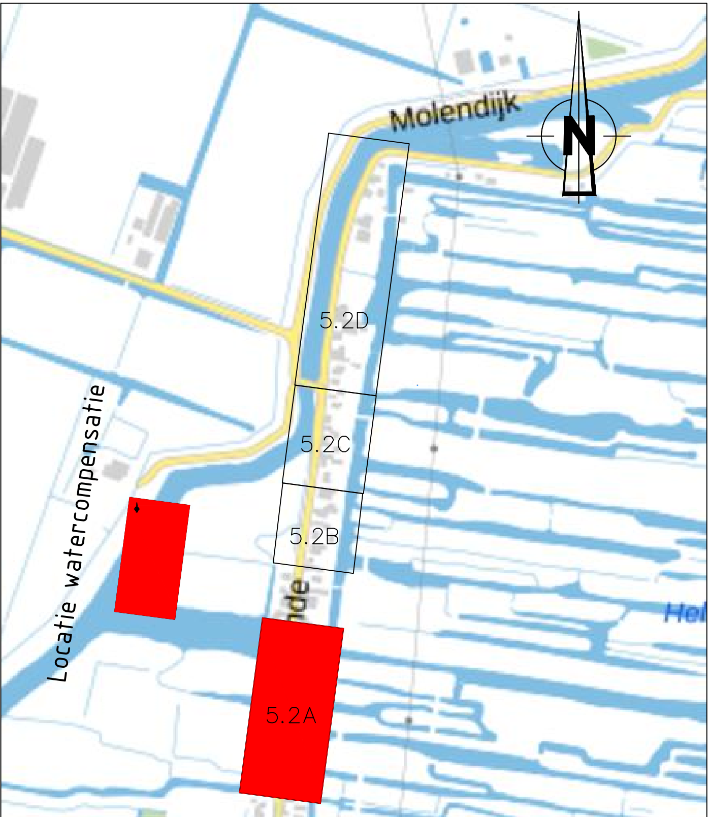
Situatie Eilandspolder Schaal 1:500
