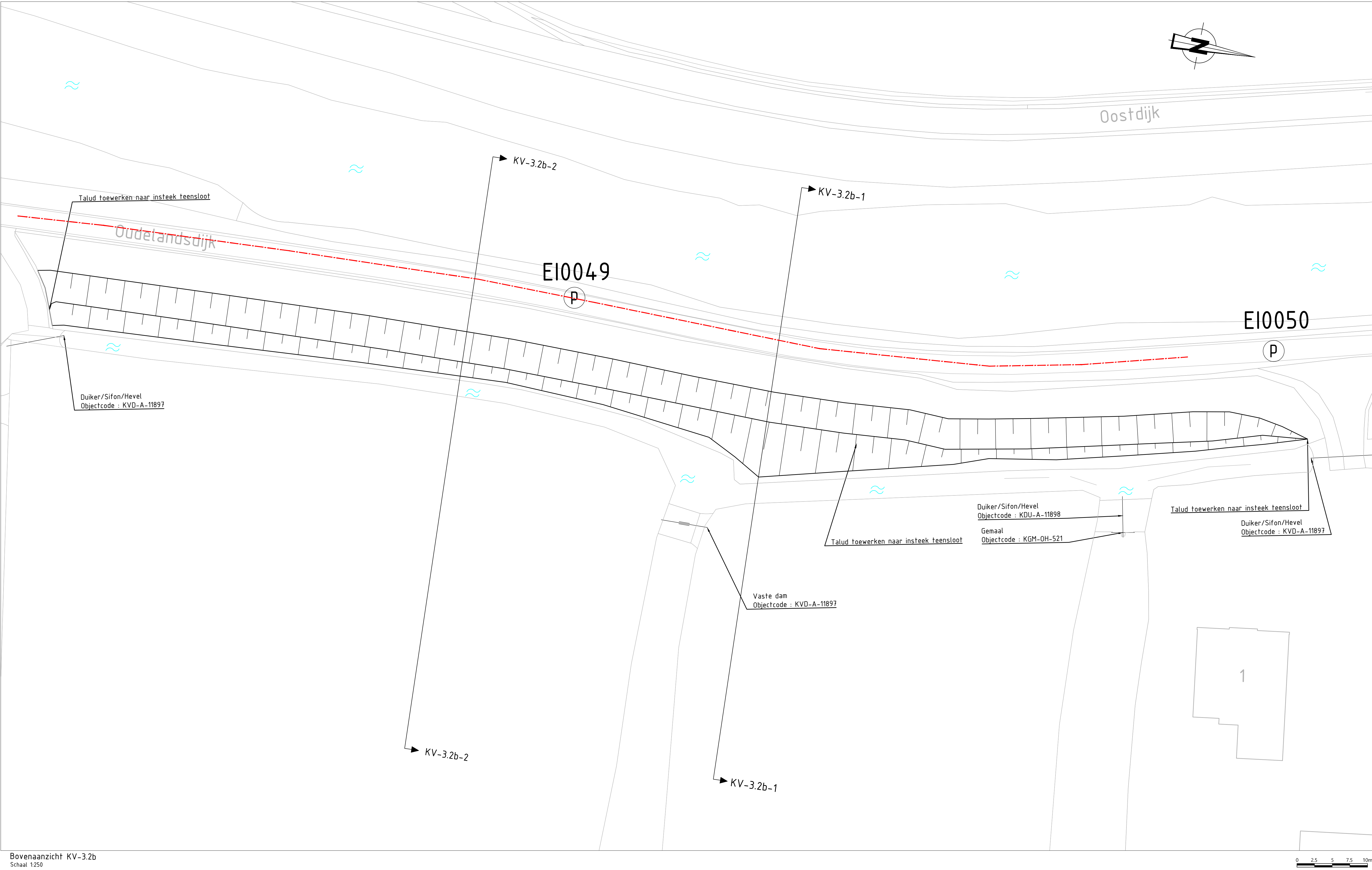
Bovenaanzicht KV-3.2b Schaal 1:250
