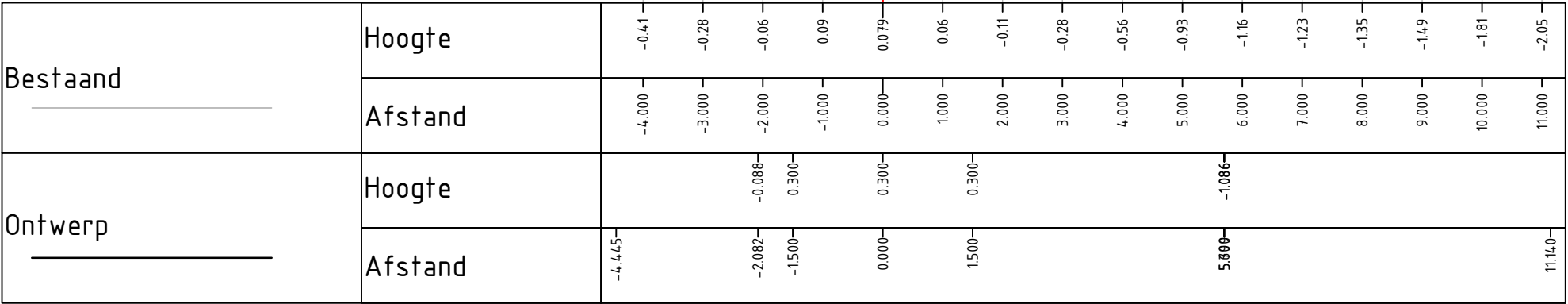
Dwarsprofiel KV-9.2b-1 t.o.v. as ALM KV-9.2b bij metrereng 25470.001 Schaal 1:100
