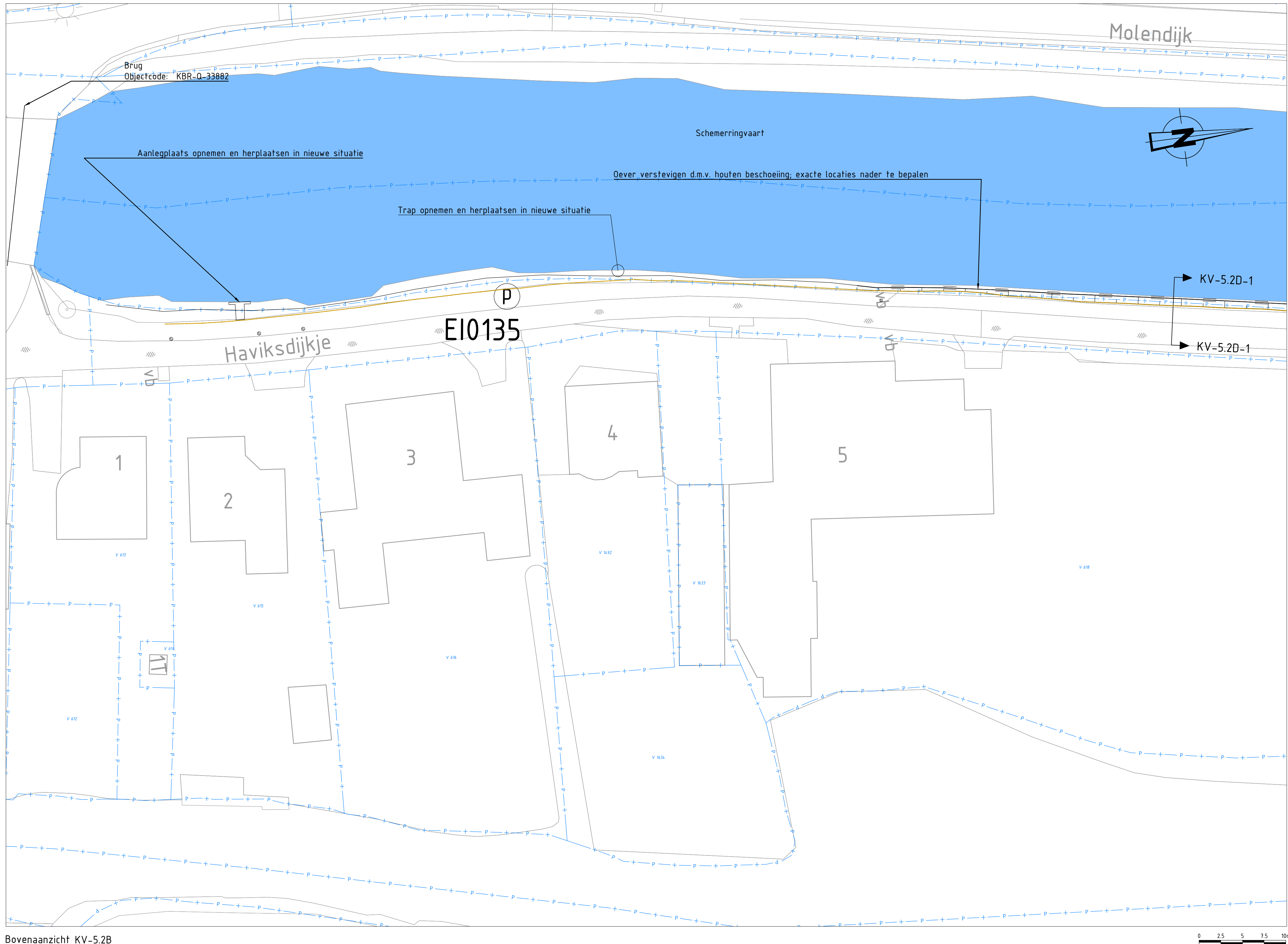
Bovenaanzicht KV-5.2B Schaal 1:250
