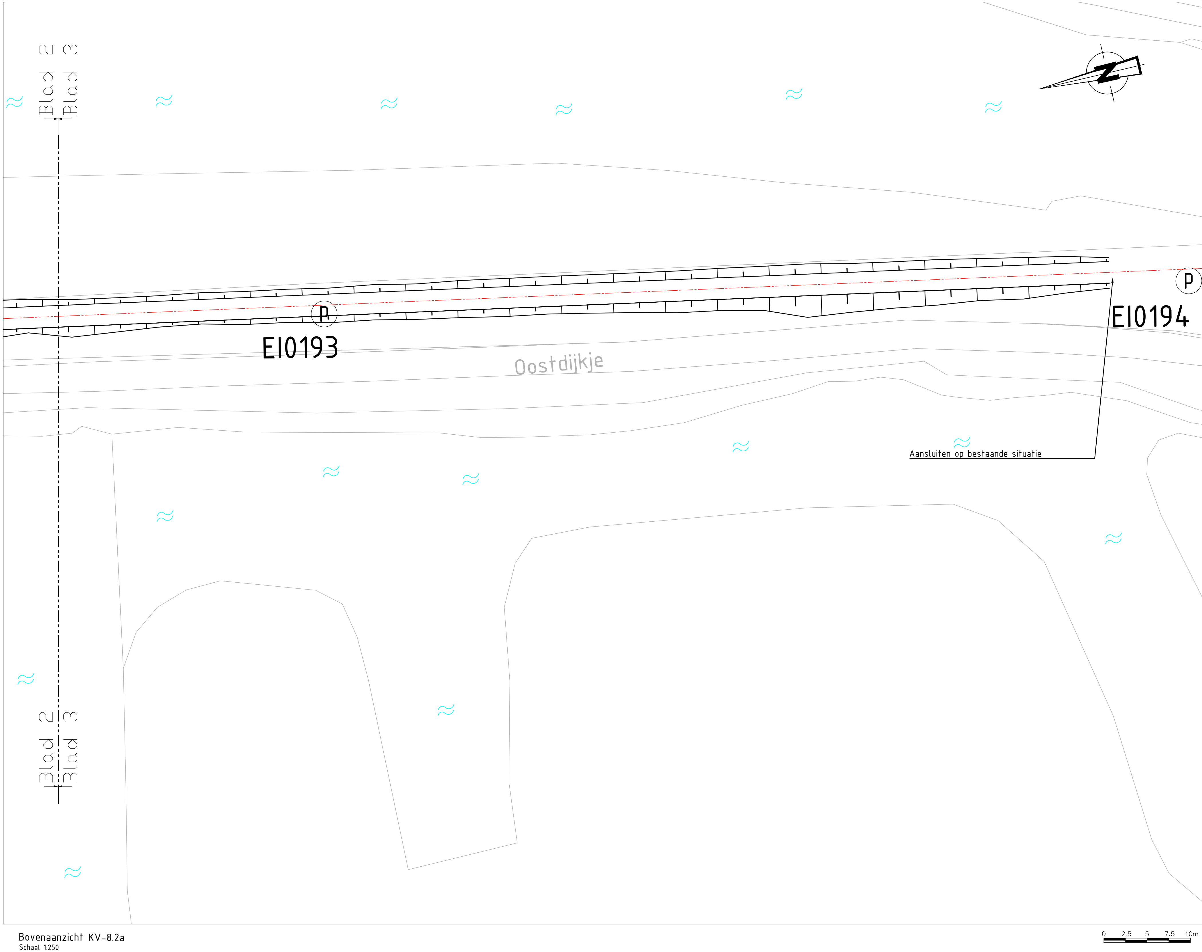
Bovenaanzicht KV-8.2a Schaal 1:250
