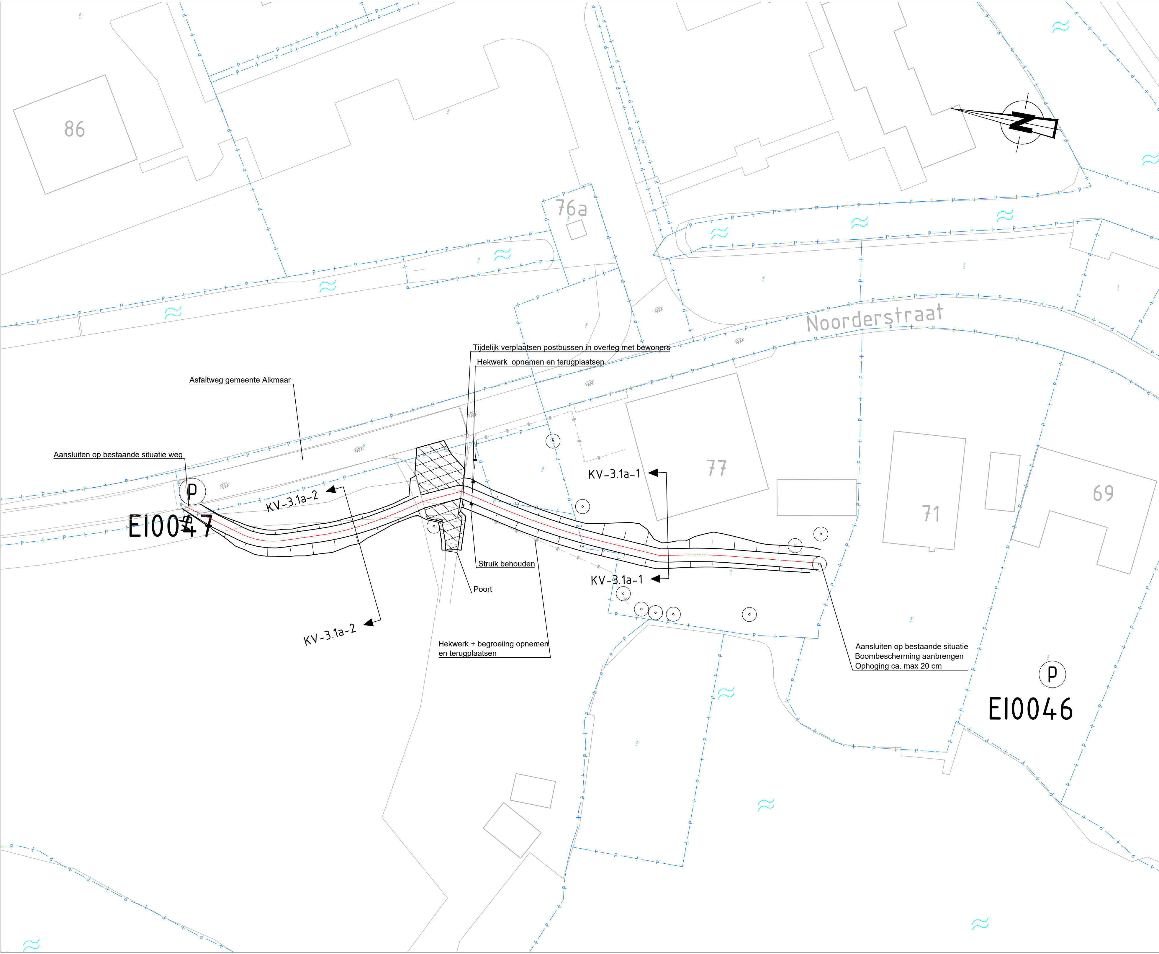
Bovenaanzicht KV-3.1a Schaal 1:250
