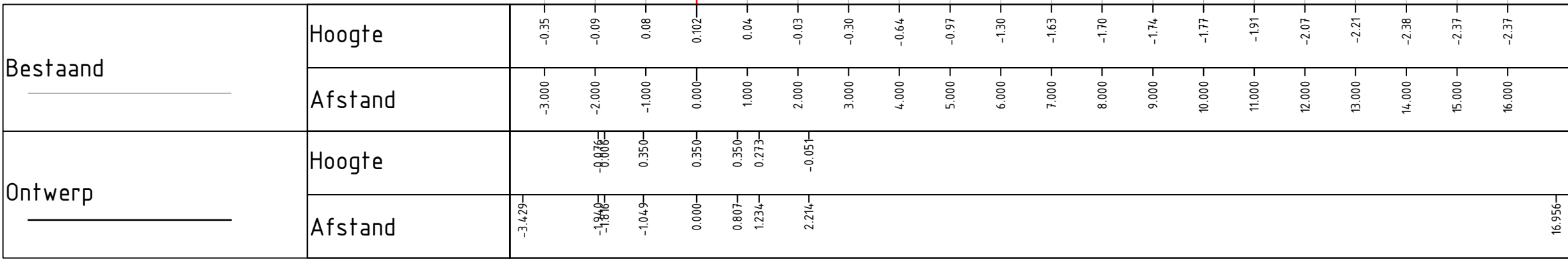
Dwarsprofiel DP-09 t.o.v. as As-kruin bij metreering 566.807 Schaal 1:100
