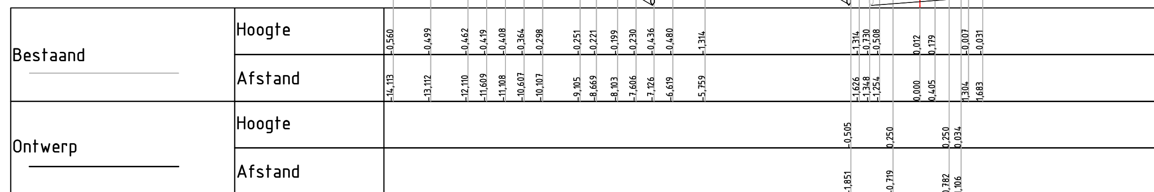
Dwarsprofiel KV-5.2A-2 t.o.v. as ALM - 5.2A bij meirering 79.438 Schaal 1:100
