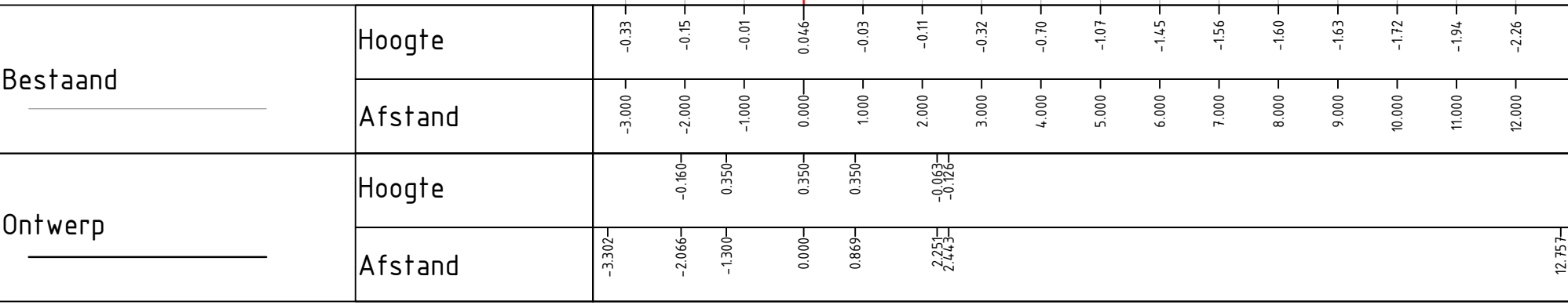
Dwarsprofiel DP-15 t.o.v. as As-kruin bij metreering 1219.131 Schaal 1:100
