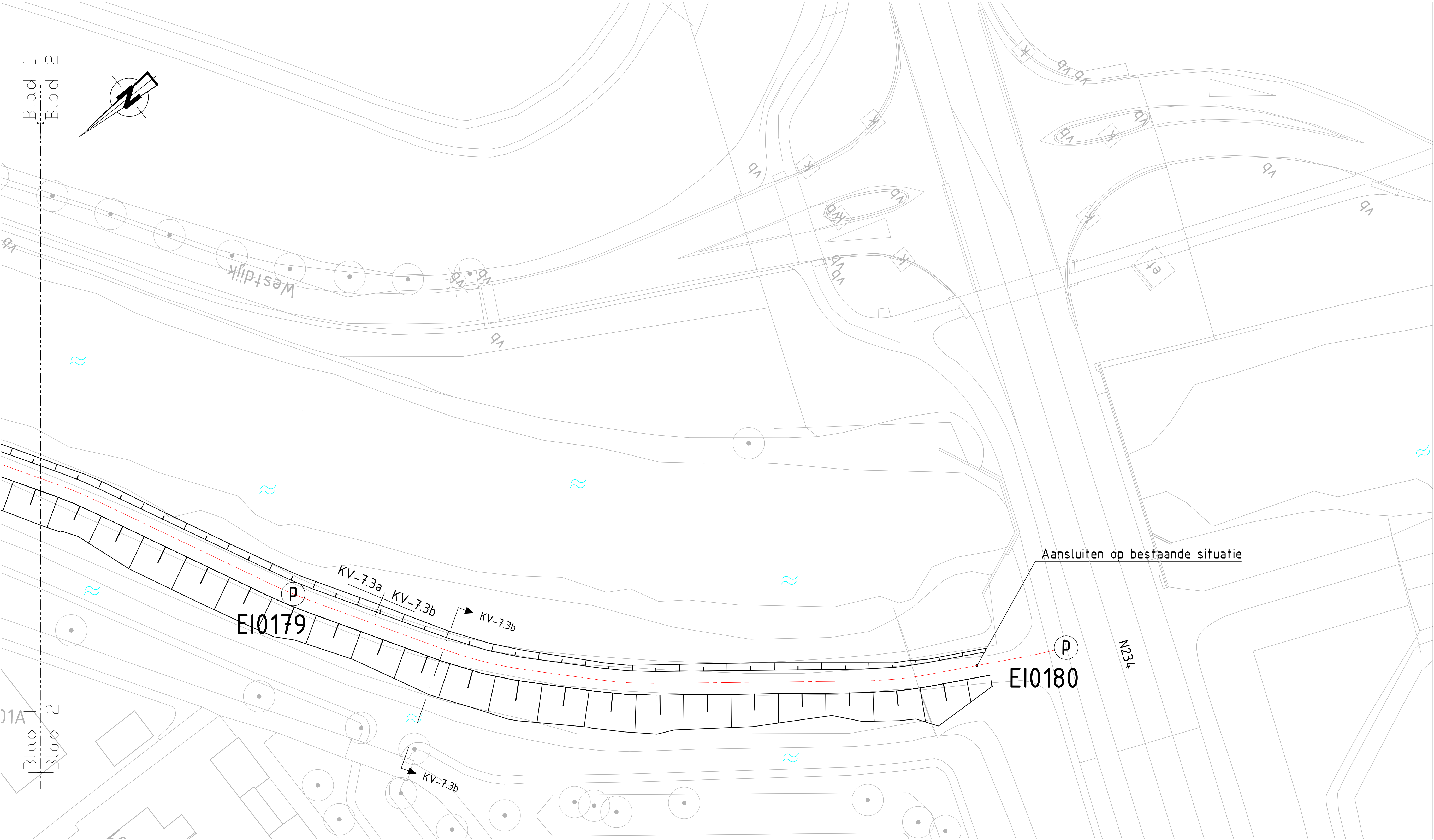
Bovenaanzicht KV-7.3a Schaal: 1:250
