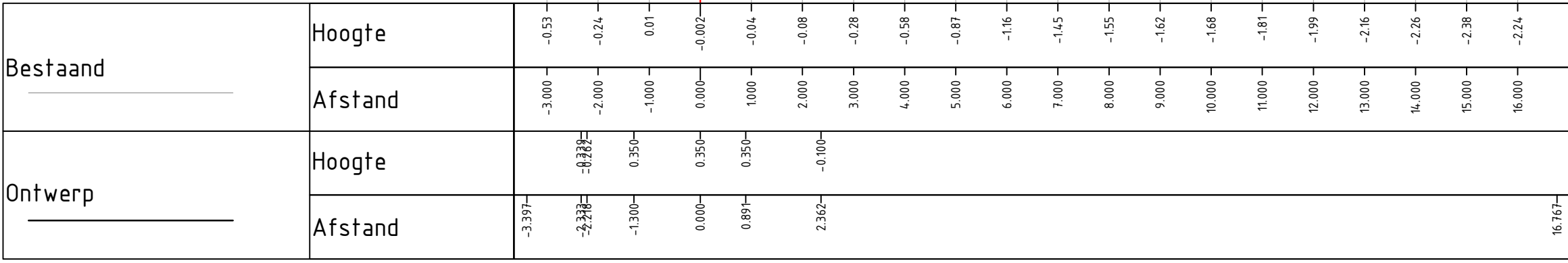
Dwarsprofiel DP-12 t.o.v. as As-kruin bij metreering 814.109 Schaal 1:100
