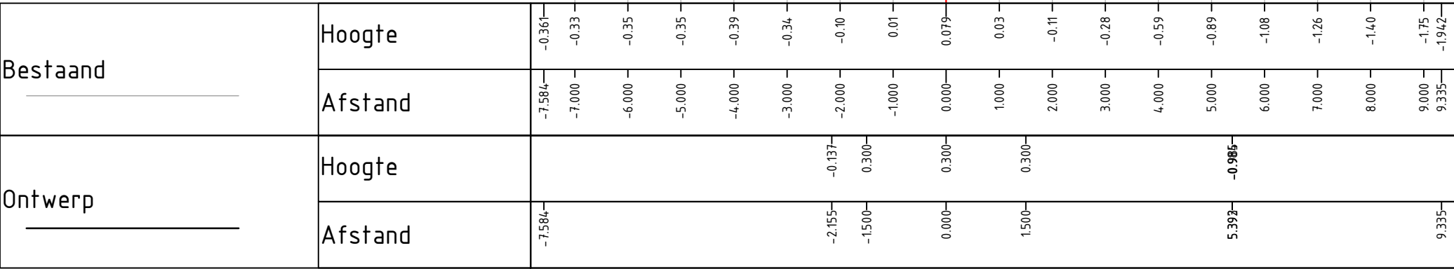
Dwarsprofiel KV-9.2d-1 t.o.v. as ALM KV-9.2d bij metrereng 26230.001 Schaal 1:100
