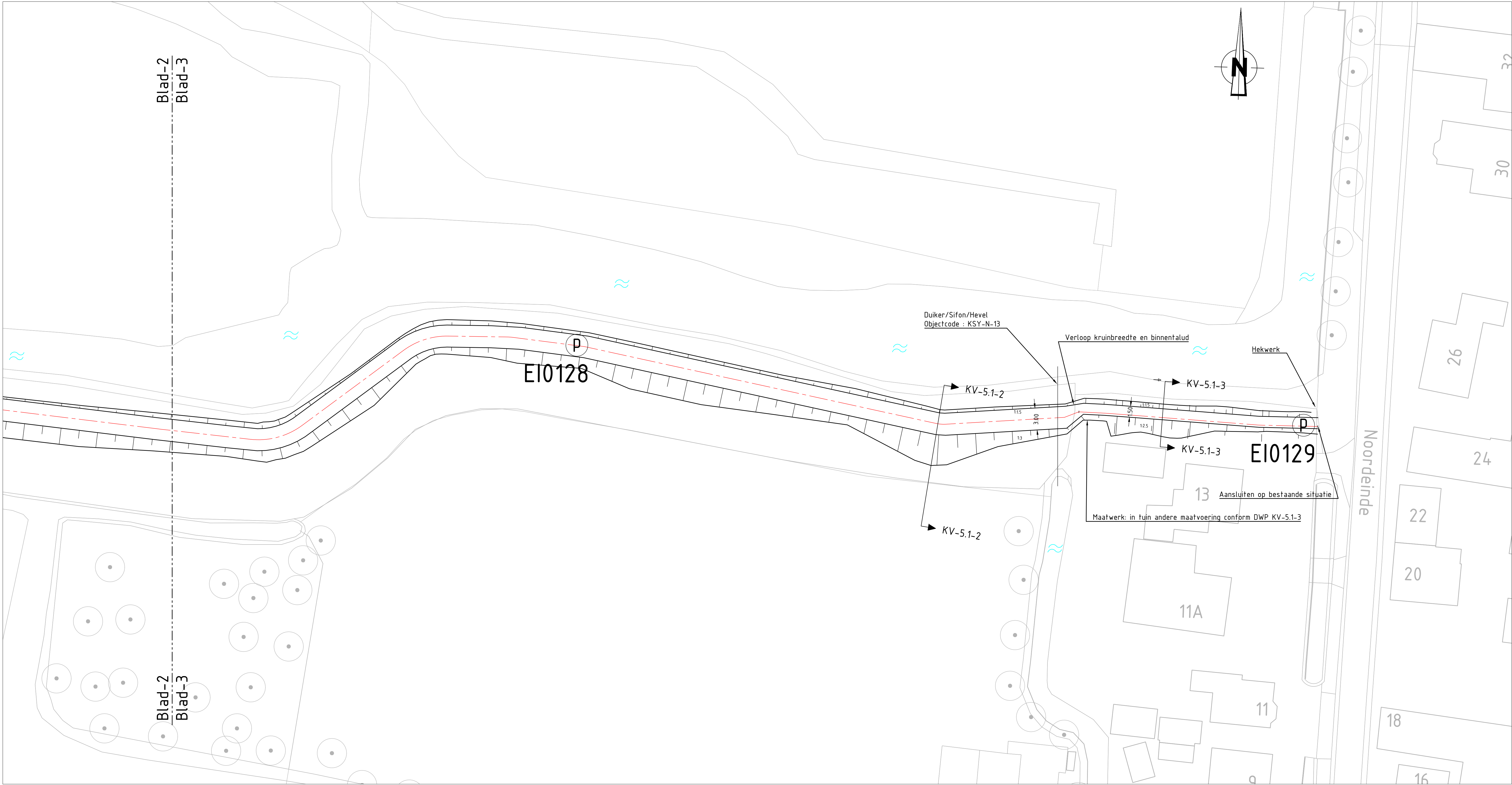
Bovenaanzicht KV-5.1 Schaal 1:250
