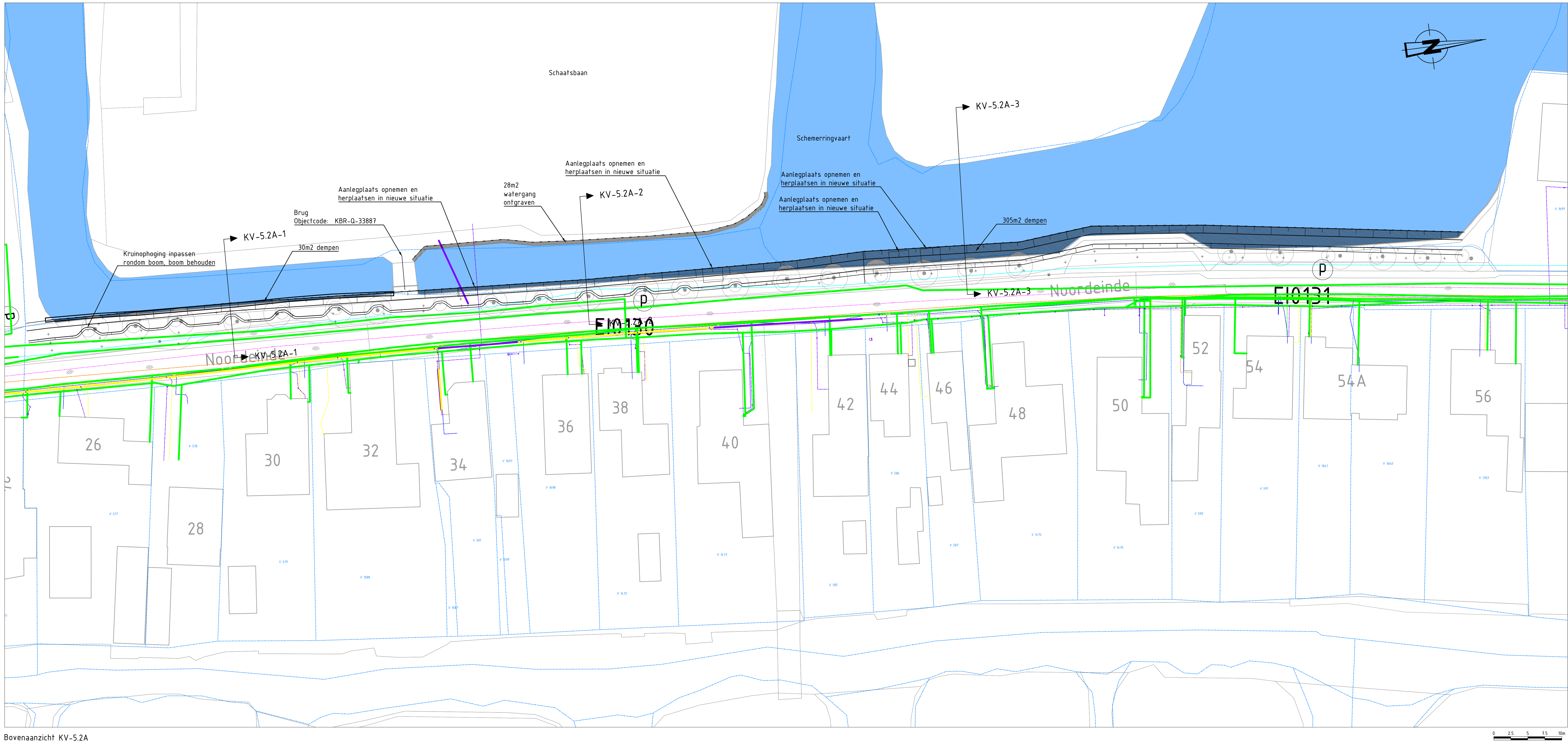
Bovenaanzicht KV-5.2A Schaal 1:250
