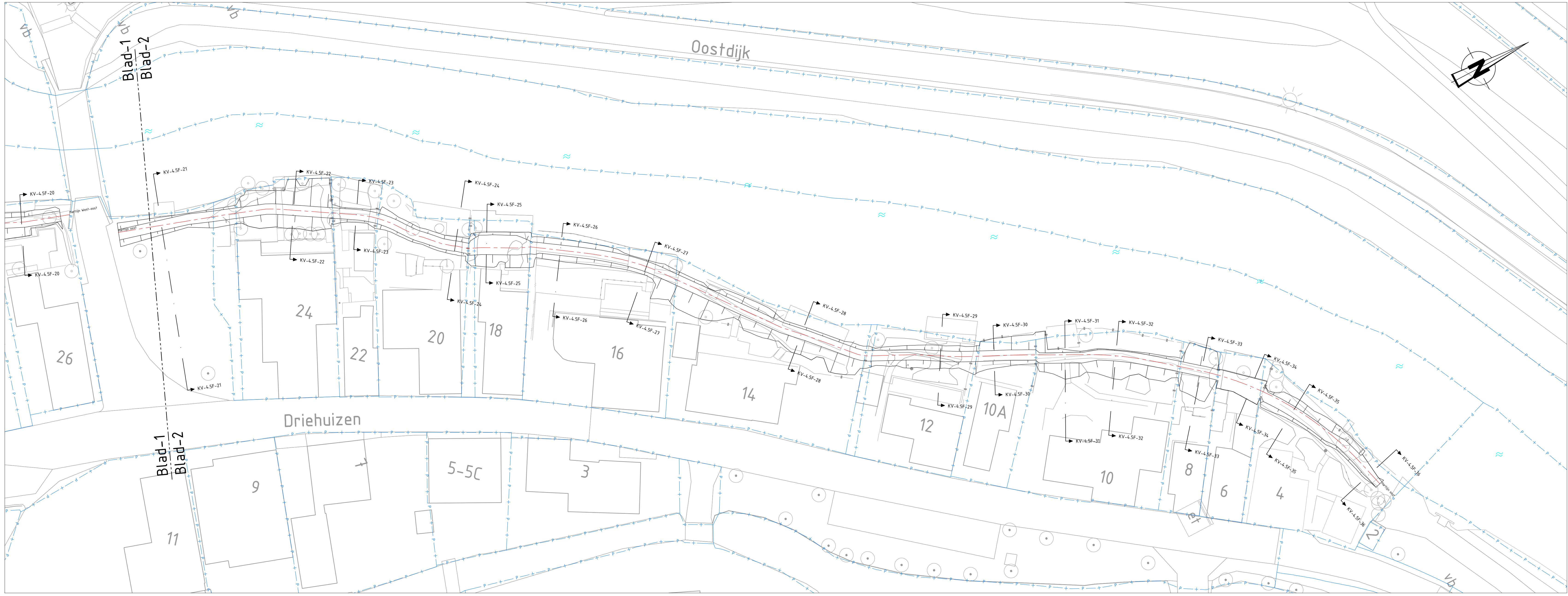
Bovenaanzicht KV-4.5F: 2 Schaal 1:250
