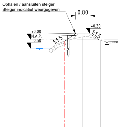
Dwarsprofiel KV-2.4-3 t.o.v. as ALM – Kant stortsteen bij metreering 187.777 Schaal 1:100
