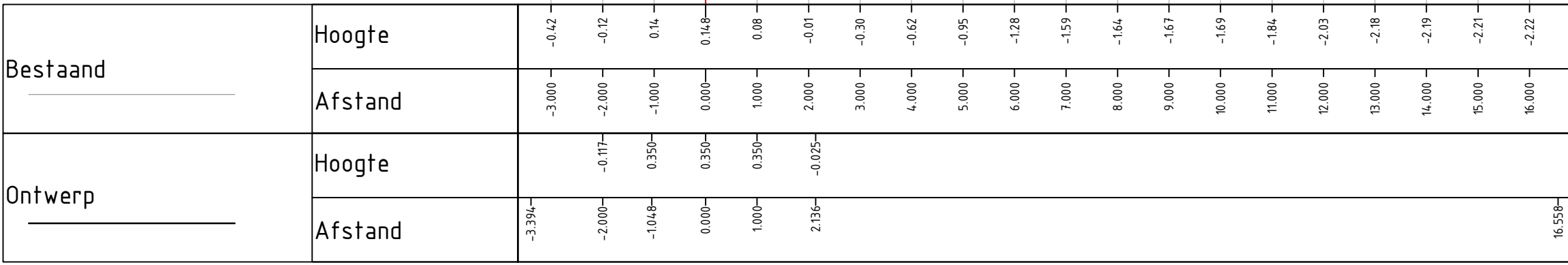
Dwarsprofiel DP-11 t.o.v. as As-kruin bij metreering 725.806 Schaal 1:100
