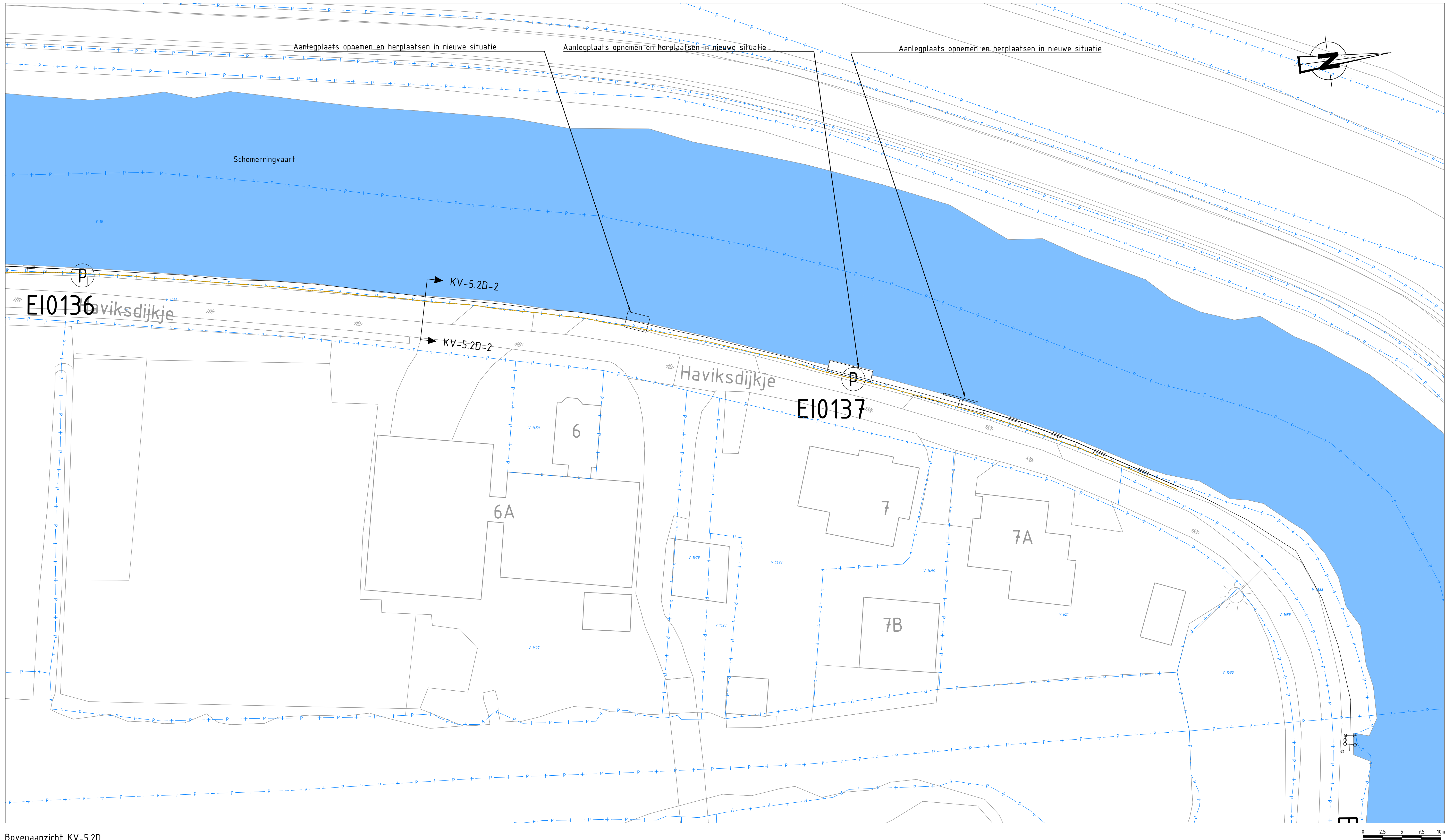
Bovenaanzicht KV-5.2D Schaal 1:250
