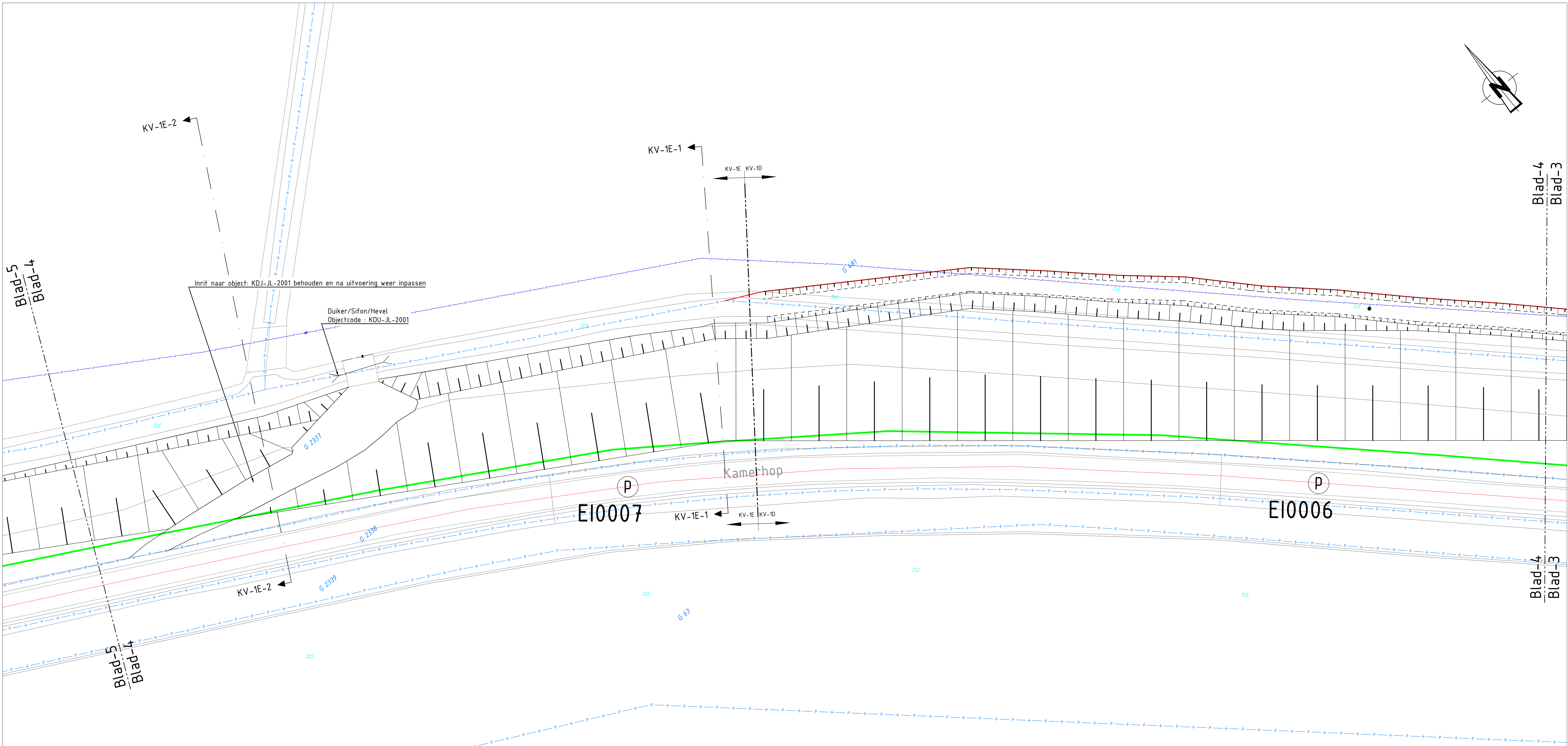
Bovenaanzicht KV-1 Schaal 1:250
