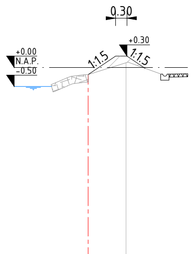
Dwarsprofiel KV-2.4-2 t.o.v. as ALM – Kant stortsteen bij metreering 141.849 Schaal 1:100
