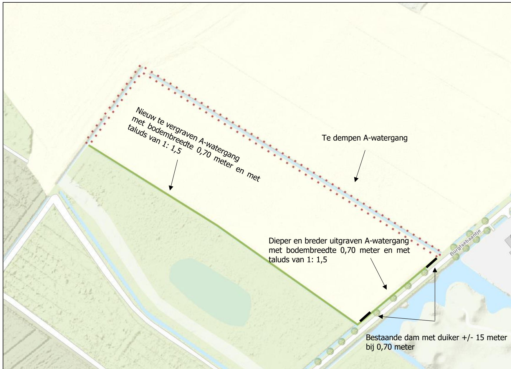
Situatietekening dempen en graven watergangen nabij Burgtsebaantje te Molenschot
