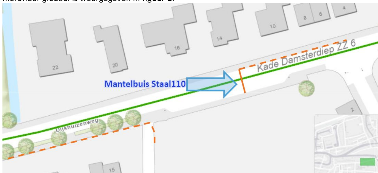
Figuur 1: Weergave werkzaamheden (oranje lijn) in en nabij de regionale waterkering.
