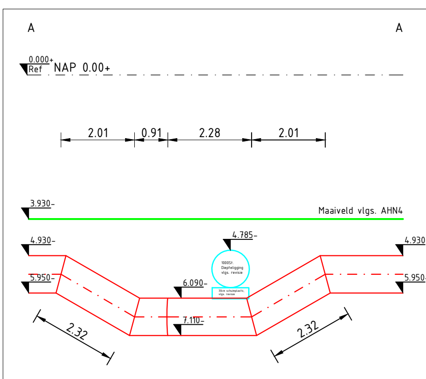
Dwarsdoorsnede A-A
