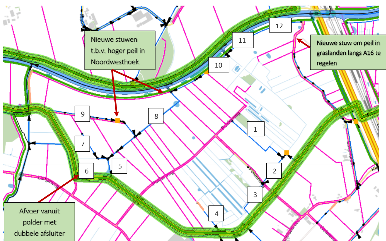
Figuur 14: Aanpassingen A watergangen en stuwen in Weimeren.
