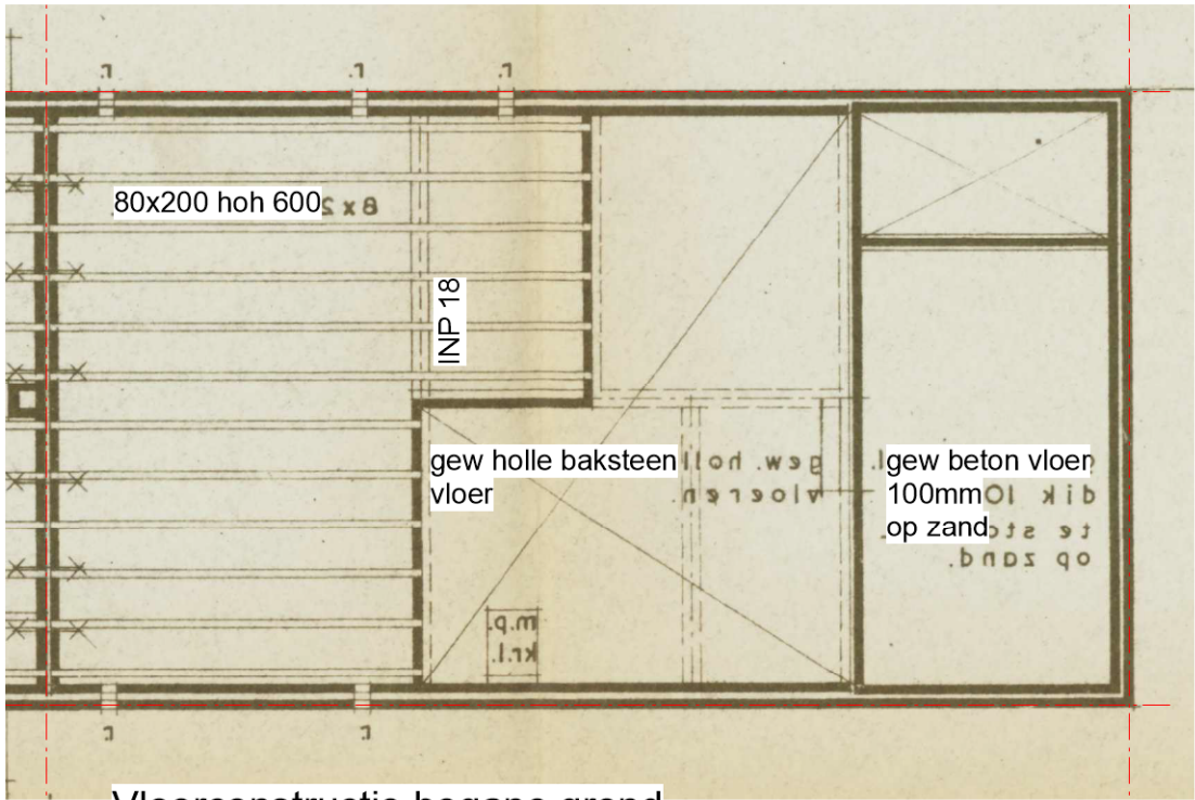
Vloerconstructie begane grond
