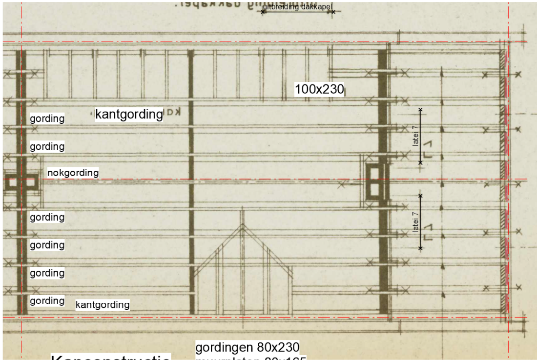
Kapconstructie
