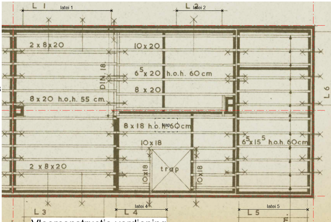
Vloerconstructie verdieping
