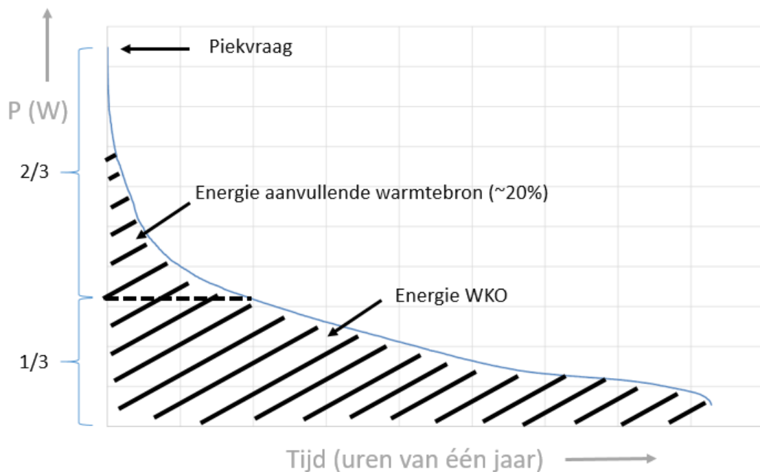
Figuur Fout! Geen tekst met de opgegeven stijl in het document.-5 Jaarbelastingduurkromme bivalent systeem [11]. Indicatief, als \frac{1}{3} van het vermogen uit de ondergrond gehaald wordt, kan daarmee 80% van de energie worden voorzien. Exacte percentages kunnen per gebouw en/of systeem verschillen.
