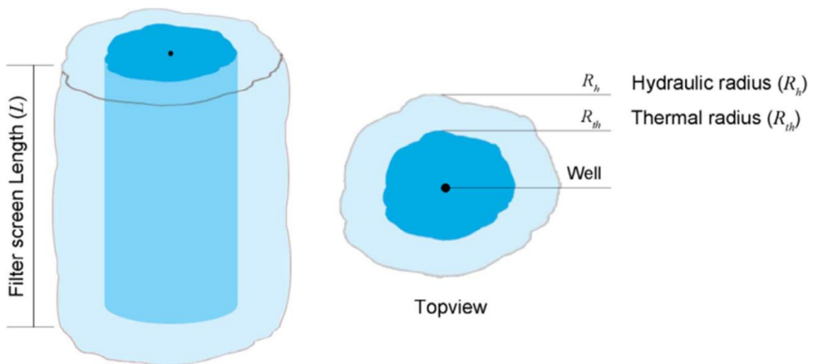
Figuur Fout! Geen tekst met de opgegeven stijl in het document.-4 Filterlengte en thermische en hydraulische straal [2].
