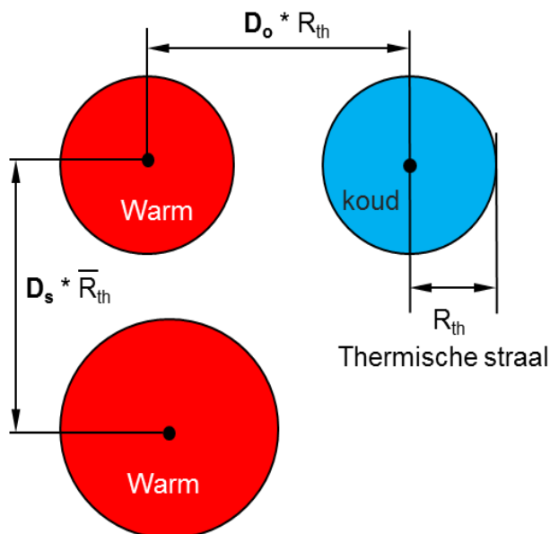
Figuur Fout! Geen tekst met de opgegeven stijl in het document.-3 De principe van bronnenafstand
