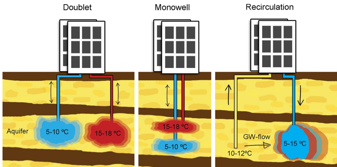
Figuur Fout! Geen tekst met de opgegeven stijl in het document.-2 Schematische weergave van doublet, monobron en recirculatie OBES [2].
