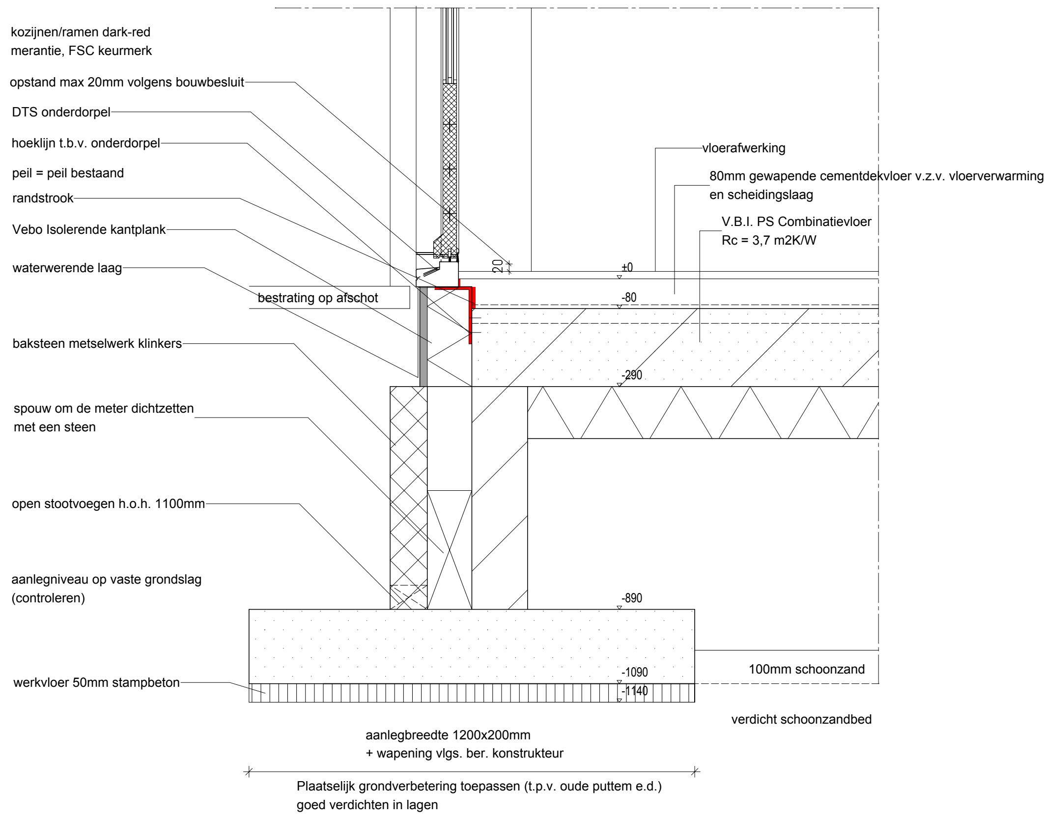
Detail 1 (onderdorpeldetail voordeur)
