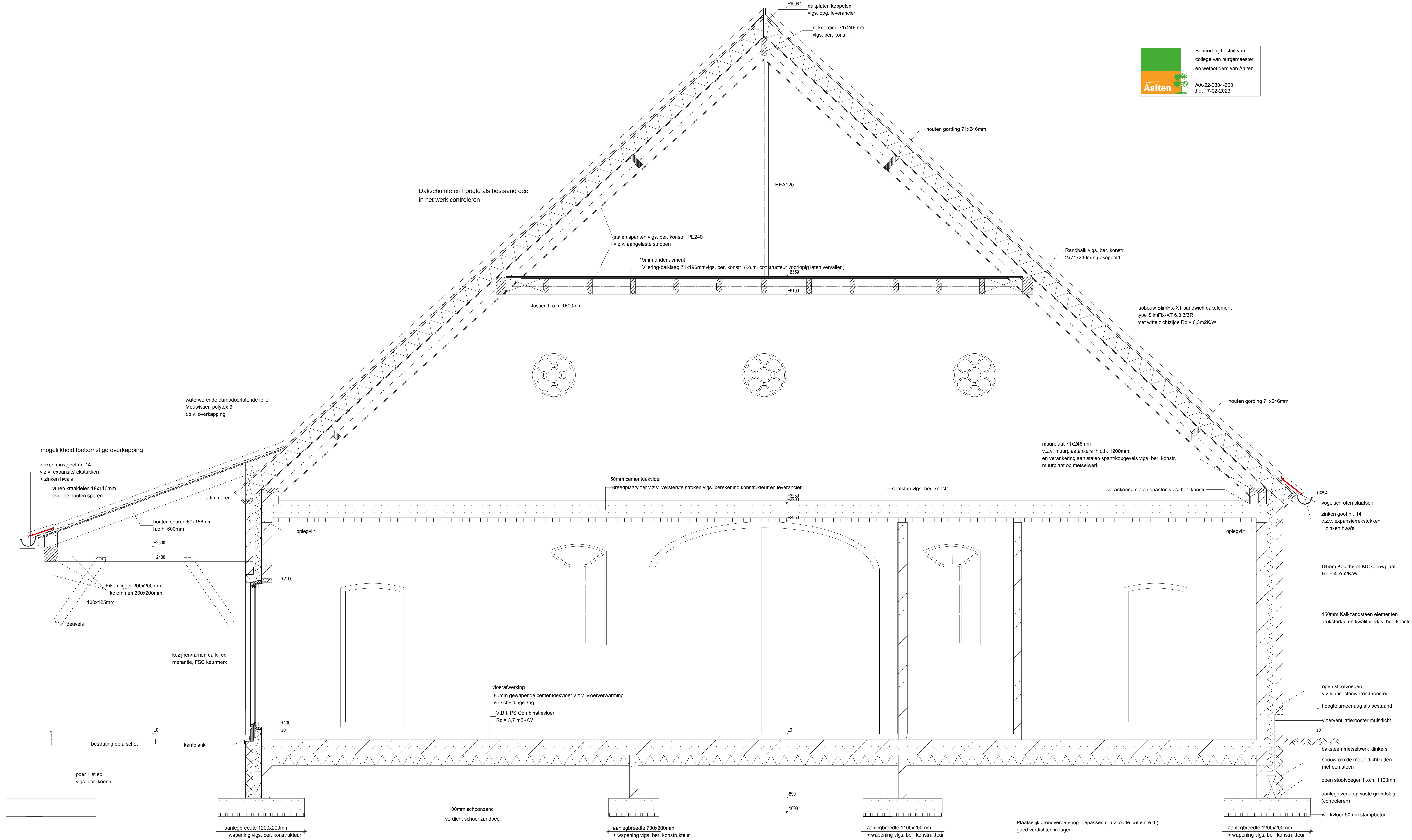
Doorsnede A-A.
