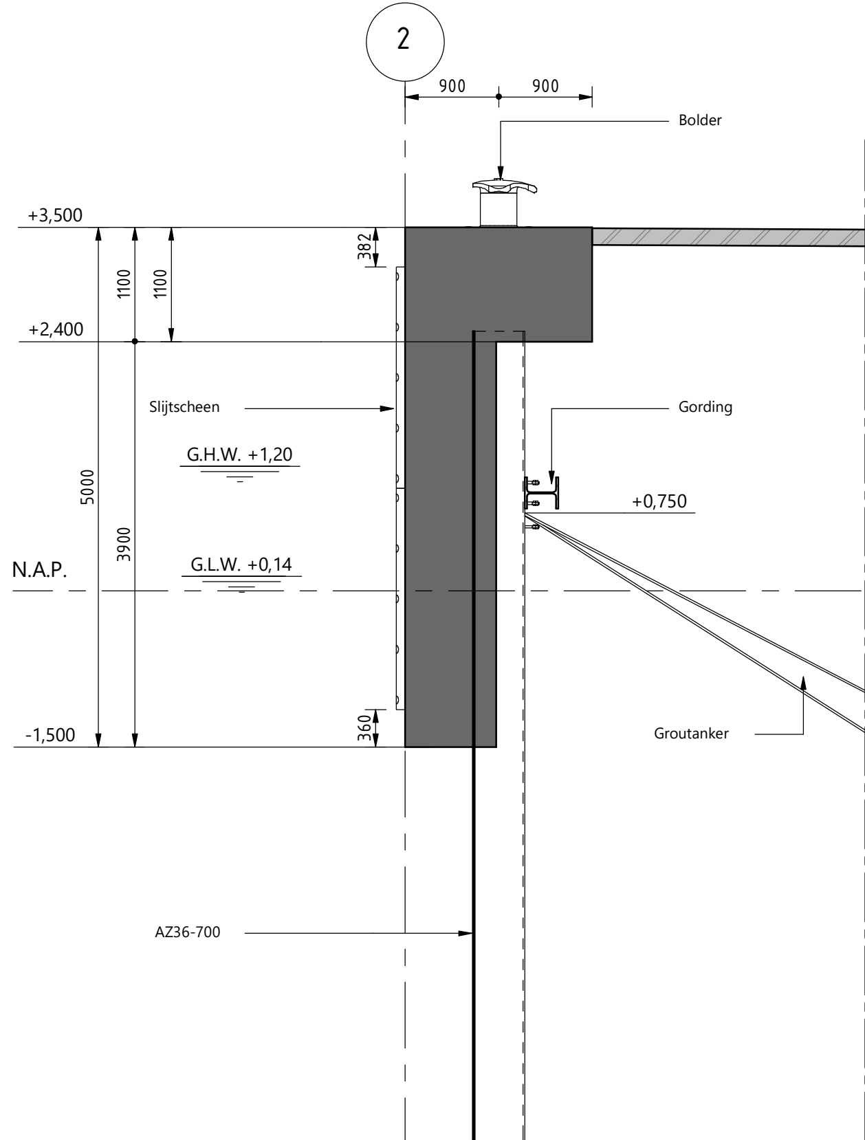
PRINCIPE DWARSDOORSNEDE DEKSLOOF
