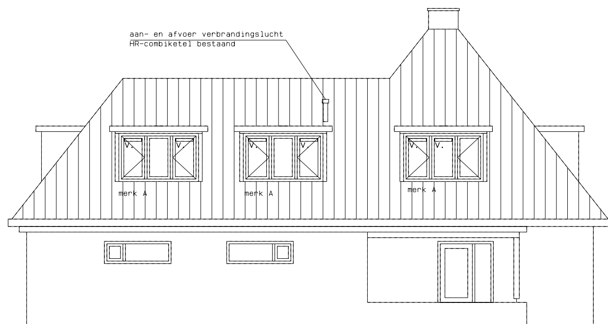
Achtergevel (gewijzigd)
