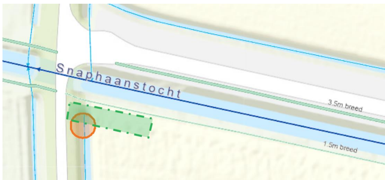
Figuur 1: Gewenste damverbreding weergegeven met oranje cirkel, gewenste stelconplaten binnen de beschermingszone van de hoofdwatergang weergegeven met groene vlak.
