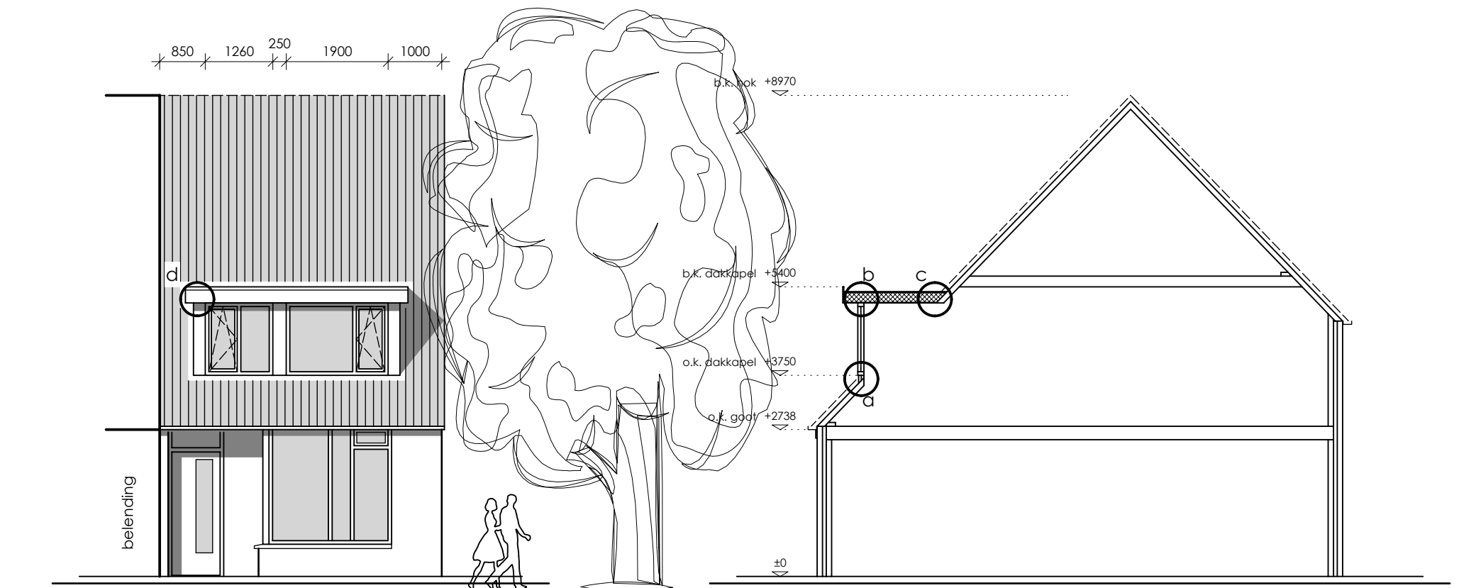
Voorgevel huidig
