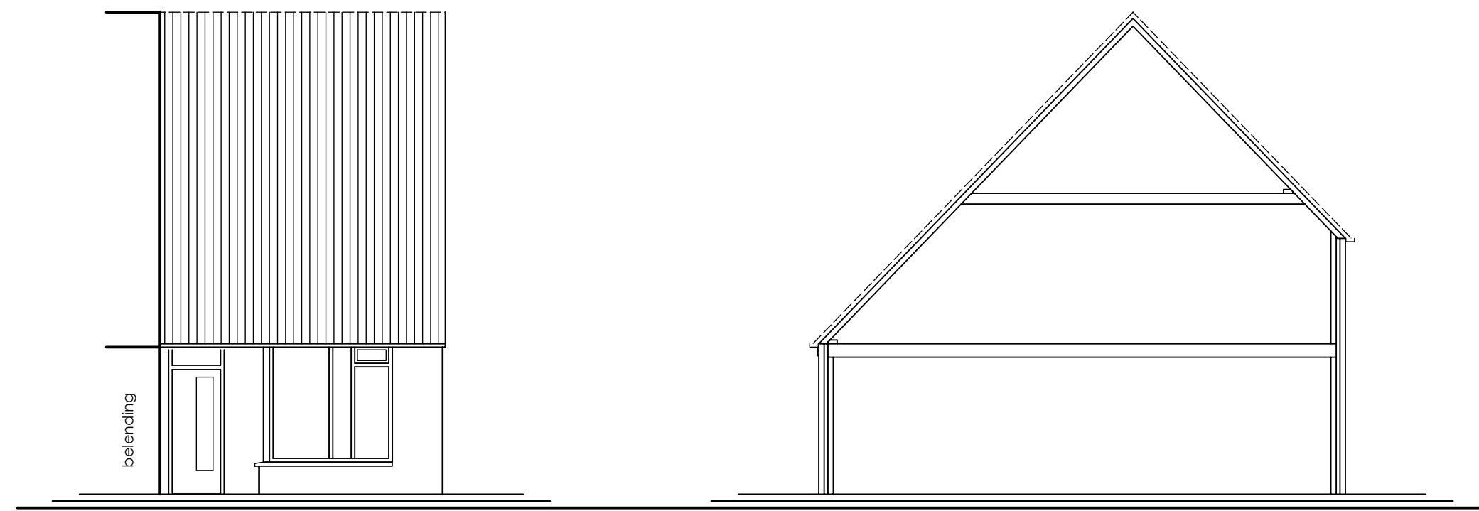
Voorgevel huidig
