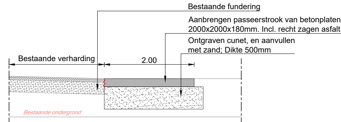
Principe doorsnede passer-/ pechstrook Schaal 1:50
