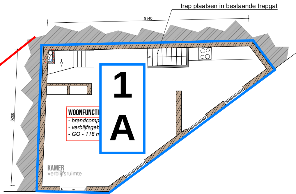
TWEDE VERDIEPING NIEUWE SITUATIE
