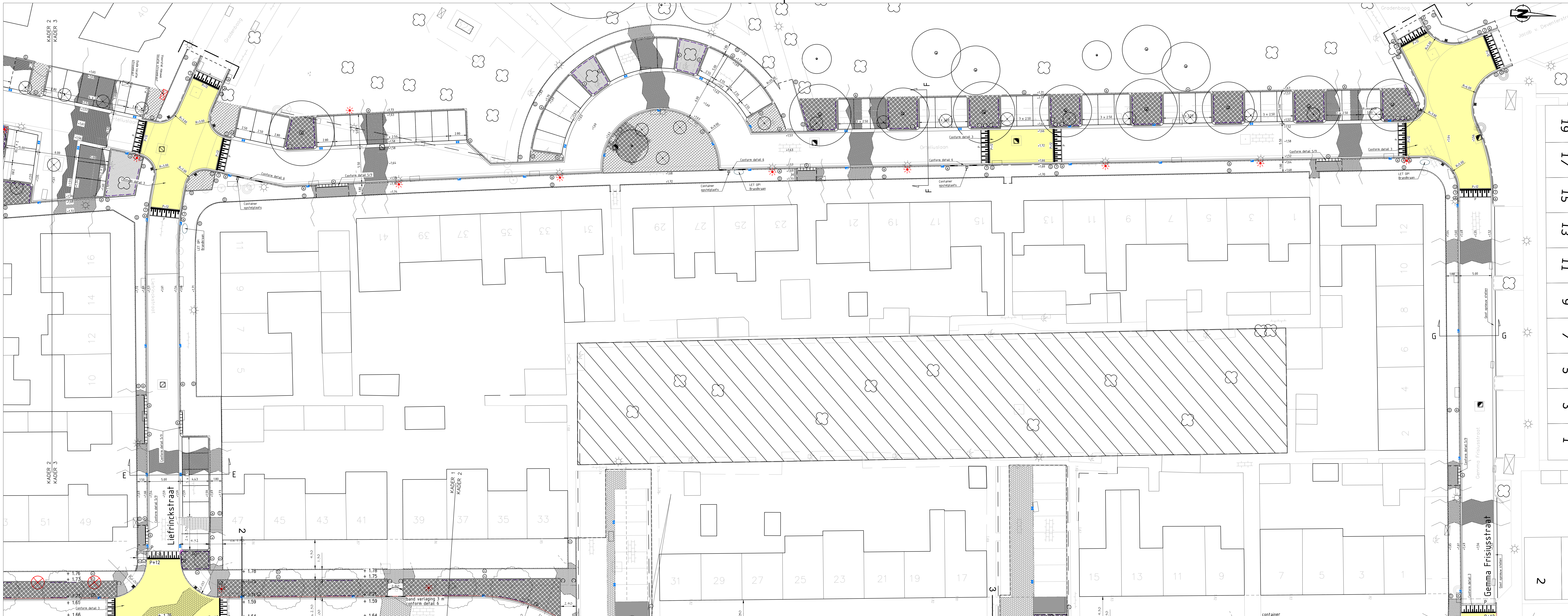
KADER 3 SCHAAL 1 : 200
