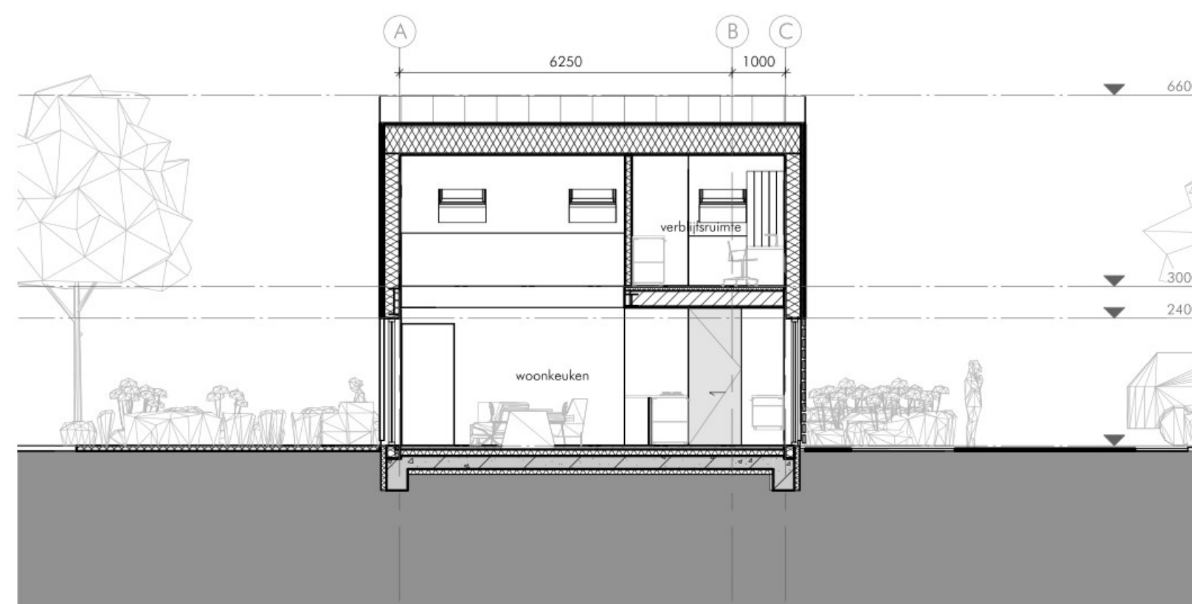
doorsnede C
