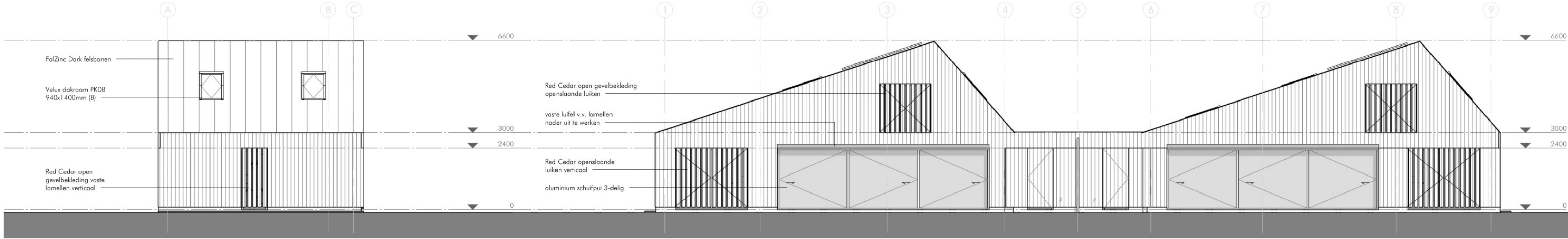
linker zijgevel (oost)
