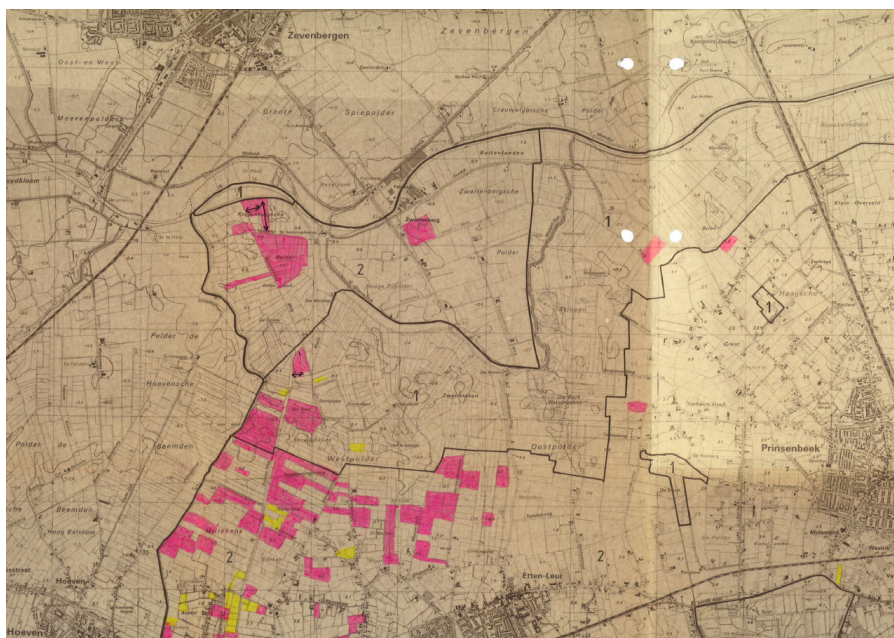
Figuur 5-14 Drainagekaart waterschap Mark&Weerijns (1995-2003). Roze kleur geeft aan dat drainage aanwezig is.
