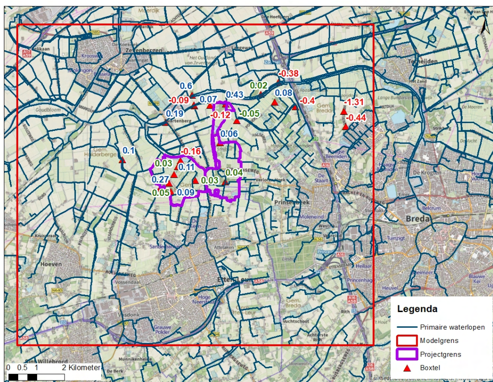
Figuur 5-18 Afwijkingen (m) in het 1ste watervoerende pakket van het gekalibreerde model ten opzichte van metingen (model-meting). Blauwe cijfers betekent dat het model te hoge stijghoogten berekent, rood te lage stijghoogten en groen zit tussen de +0.05 en -0.05 cm verschil.
