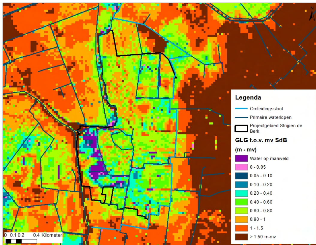
Figuur 9-19 GLG ten opzichte van maaiveld voor het extra scenario aanpassing infiltratie Strijpen de Berk.
