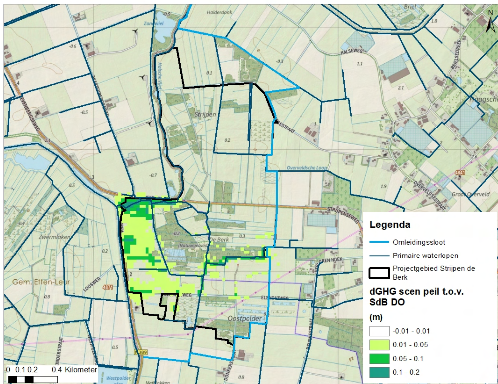
Figuur 9-22 Verschil in GHG tussen het extra scenario aanpassing peilen Strijpen de Berk en DO inrichtingsplan 2022.
