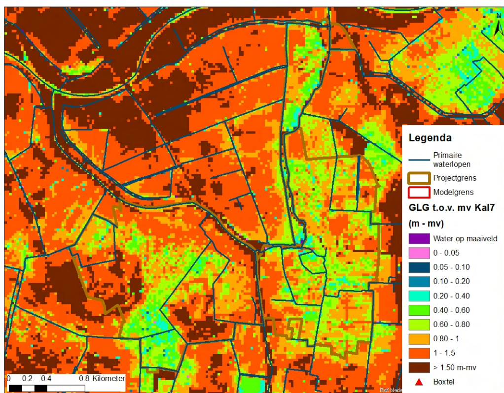
Figuur 5-26 GLG ten opzichte van maaiveld voor het gekalibreerde model.
