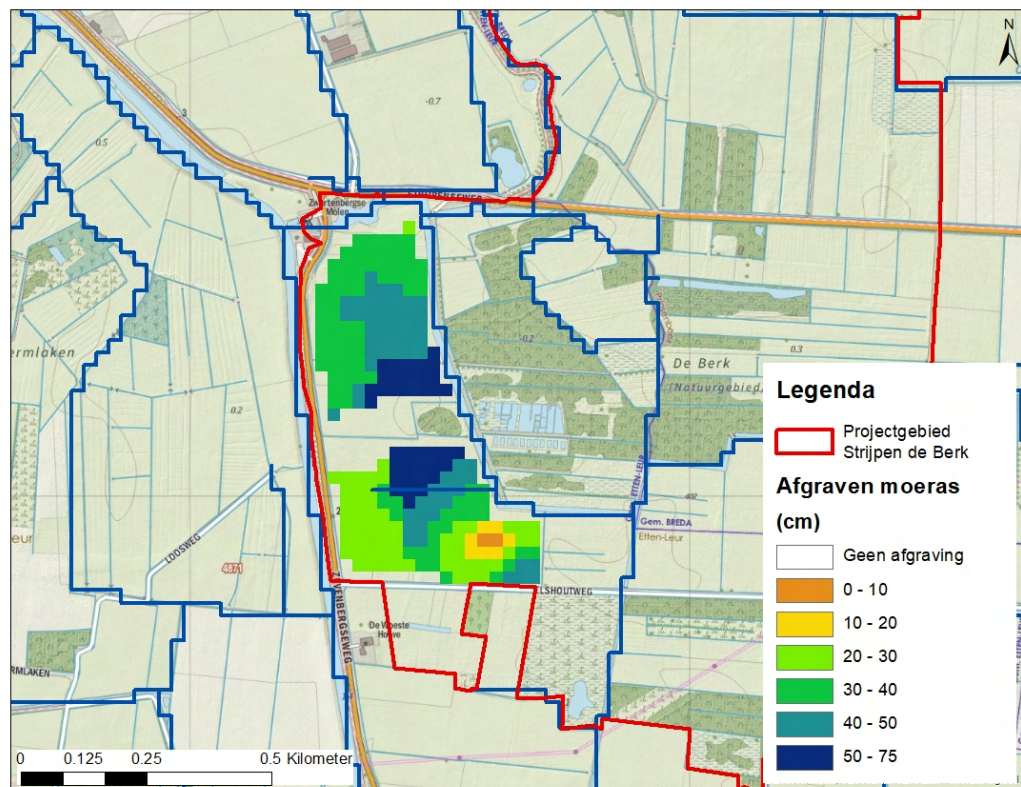
Figuur 9-5 Afgraving ten behoeve van aanleg moerasgebied.
