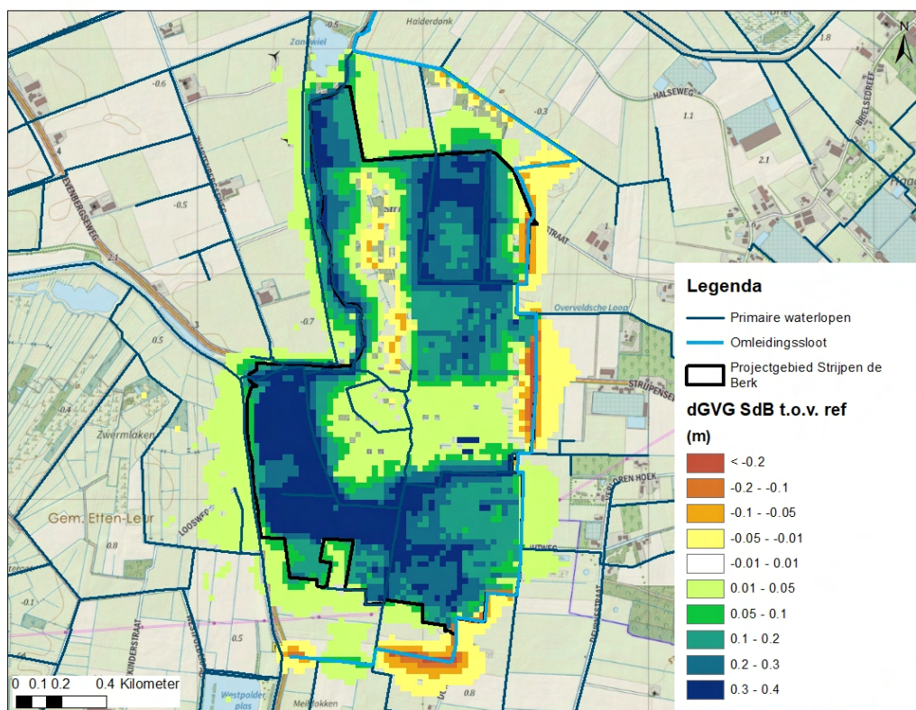
Figuur 9-8 Verschil in GVG tussen het scenario Strijpen de Berk en de referentiesituatie.
