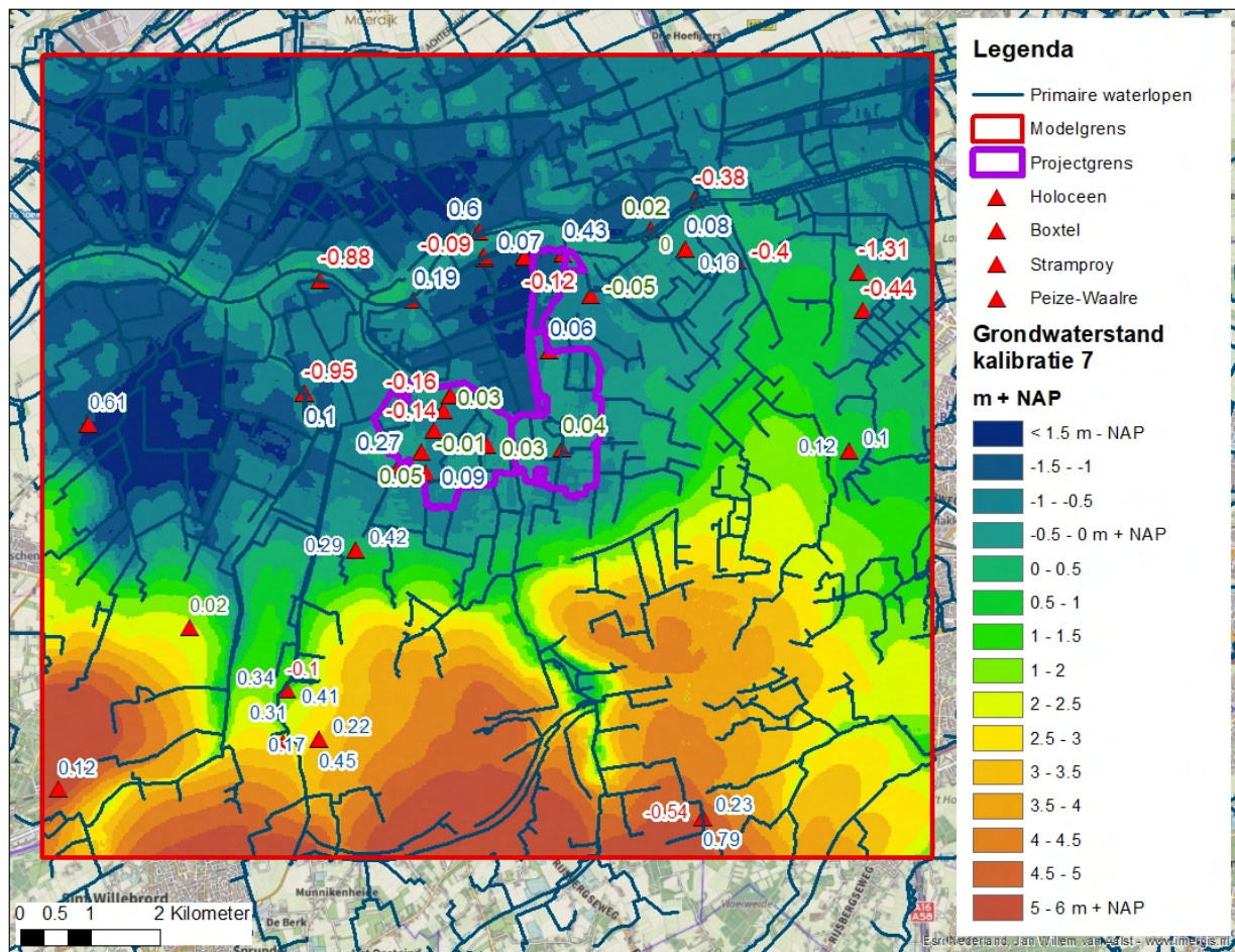
Figuur 5-17: Kalibratieresultaat hele modelgebied, peilbuizen met filter in formatie van Bostel, Stramproy of Peize Waalre. Blauwe cijfers betekend dat het model te hoge stijghoogten berekent, rood te lage stijghoogten en groen zit tussen de +0.05 en -0.05 cm verschil.
