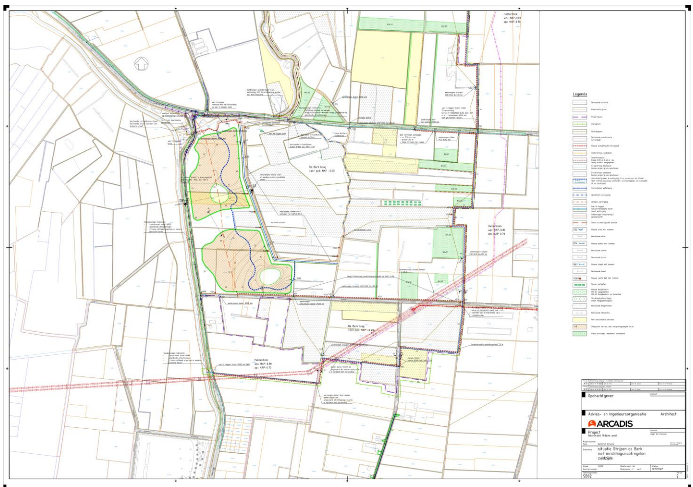
Figuur 4-18 Definitief Ontwerp, zuidelijk deel (De Berk)
