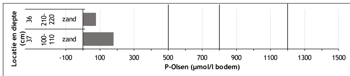
Figuur 31. De plantbeschikbare fosfaatconcentratie per bodemonster (in \mu\text{mol/l} bodem). De dikke verticale lijnen geven de randvoorwaarden van 500, 800 en 1200 \mu\text{mol/l} weer (tabel 2).
