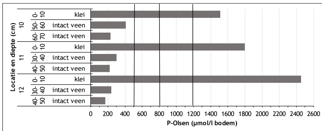
Figuur 21. De plantbeschikbare fosfaatconcentratie per bodemonster (in \mu\text{mol/l} bodem). De dikke verticale lijnen geven de randvoorwaardes van 500, 800 en 1200 \mu\text{mol/l} weer (tabel 2).
