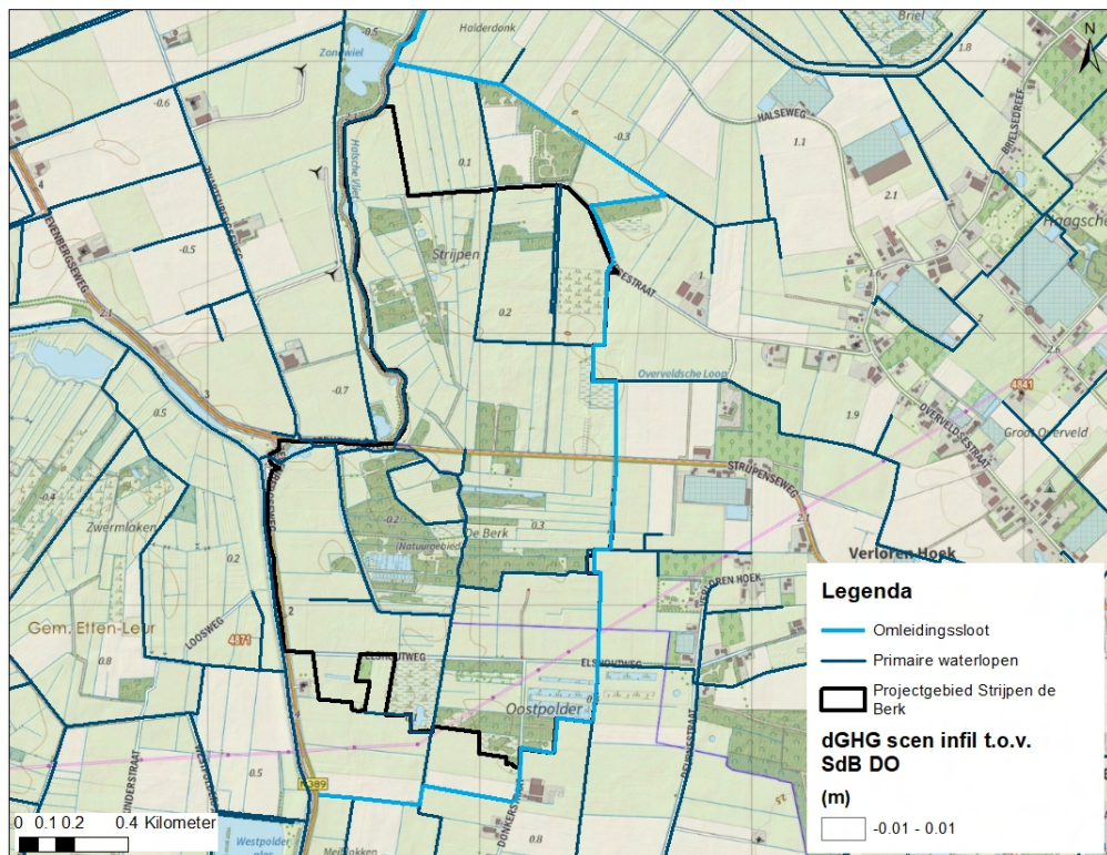
Figuur 9-14 Verschil in GHG tussen het extra scenario aanpassing infiltratie Strijpen de Berk en de DO inrichtingsplan 2022.
