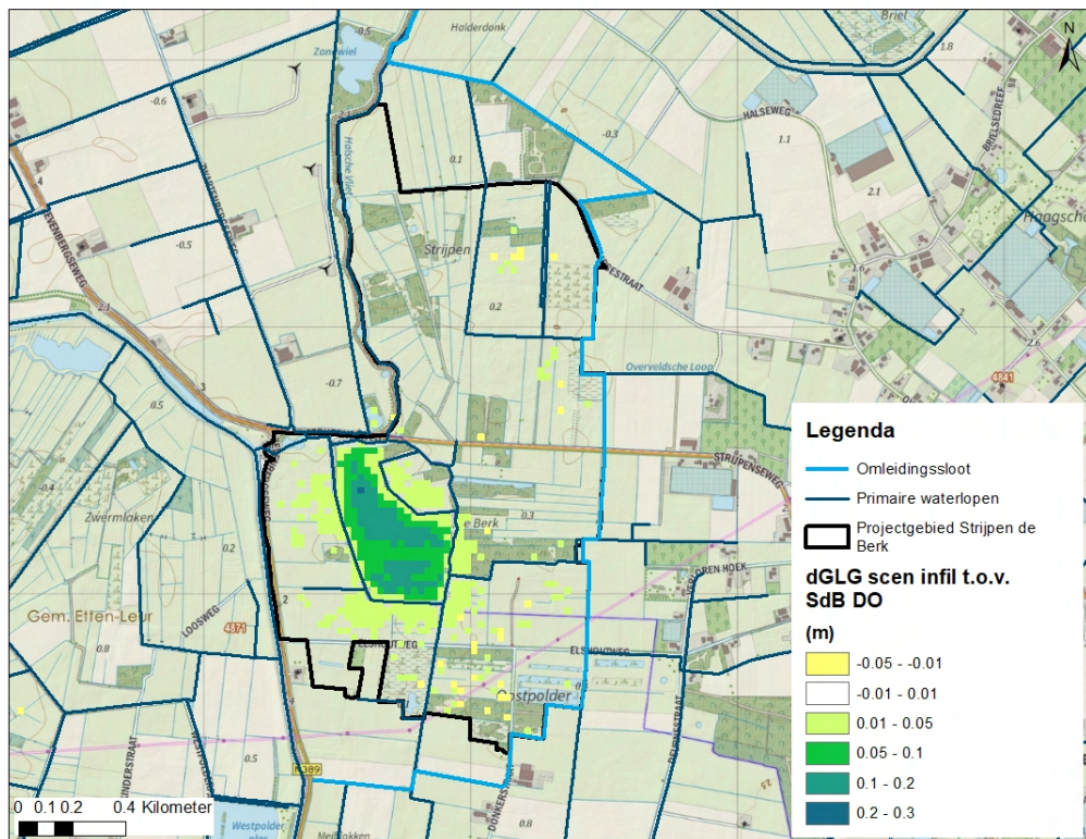
Figuur 9-18 Verschil in GLG tussen het extra scenario aanpassing infiltratie Strijpen de Berk en DO inrichtingsplan 2022.
