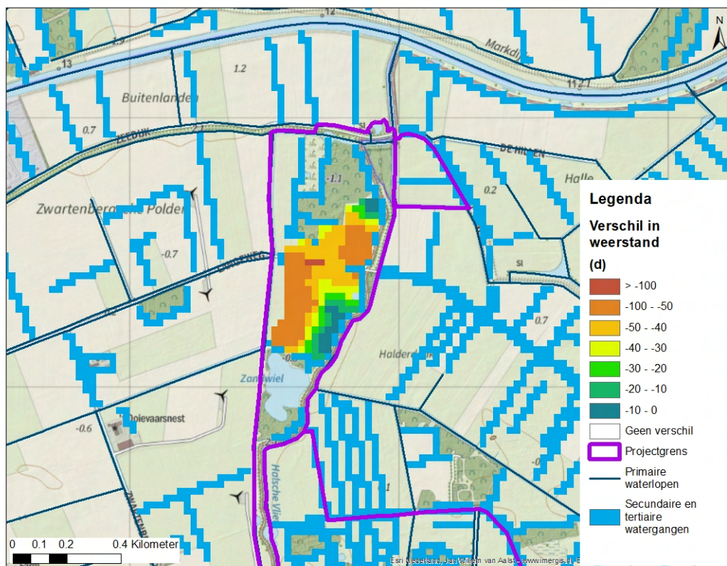
Figuur 7-4 Nieuwe deklaagweerstand in het afgegraven gebied in Zwartenbergse Polder.
