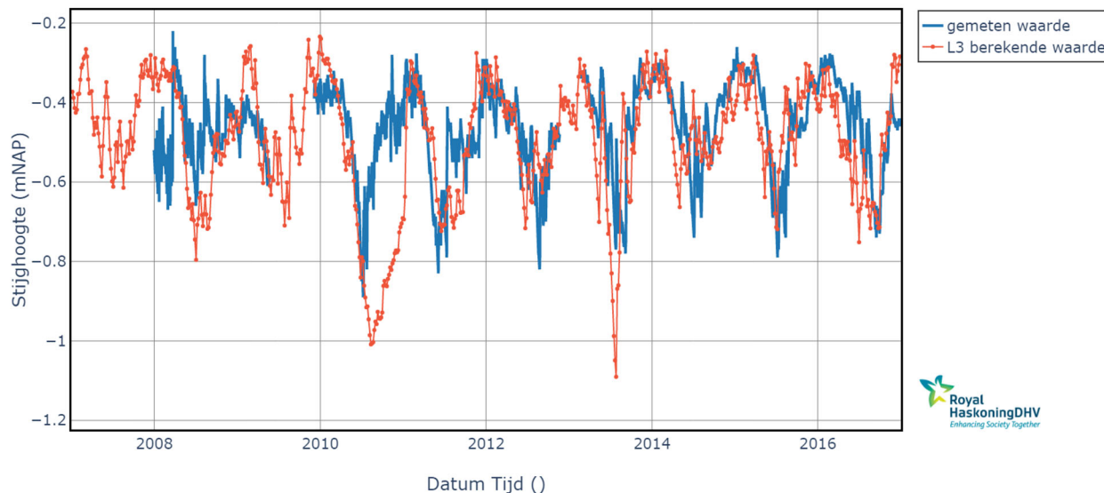
Figuur 5-21 Grafiek van model (rode lijn) en meting (blauwe lijn) voor peilbuis 1466 (zie Figuur 4-4 voor de locatie van deze peilbuis).
