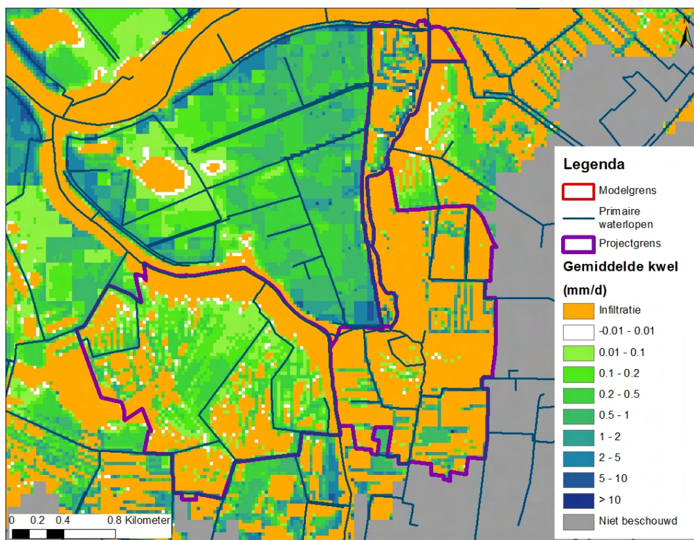
Figuur 5-27 Gemiddelde kwel in het gekalibreerde model.
