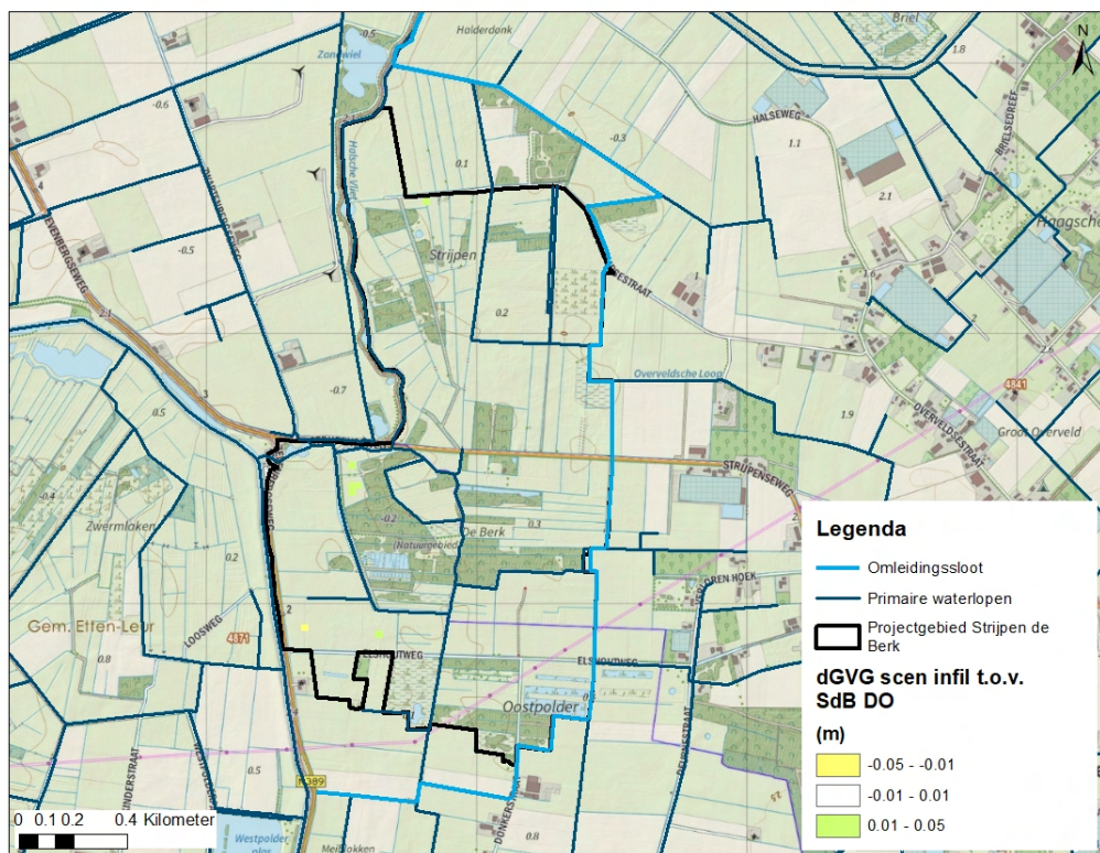
Figuur 9-16 Verskil in GVG tussen het extra scenario aanpassing infiltratie Strijpen de Berk en DO inrichtingsplan 2022.
