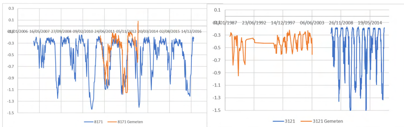
Figuur 9-36 Berekende en gemeten stijghoogte van links peilbuis 8171 en rechts peilbuis 3121. De locaties staan aangegeven in Figuur 9-35
