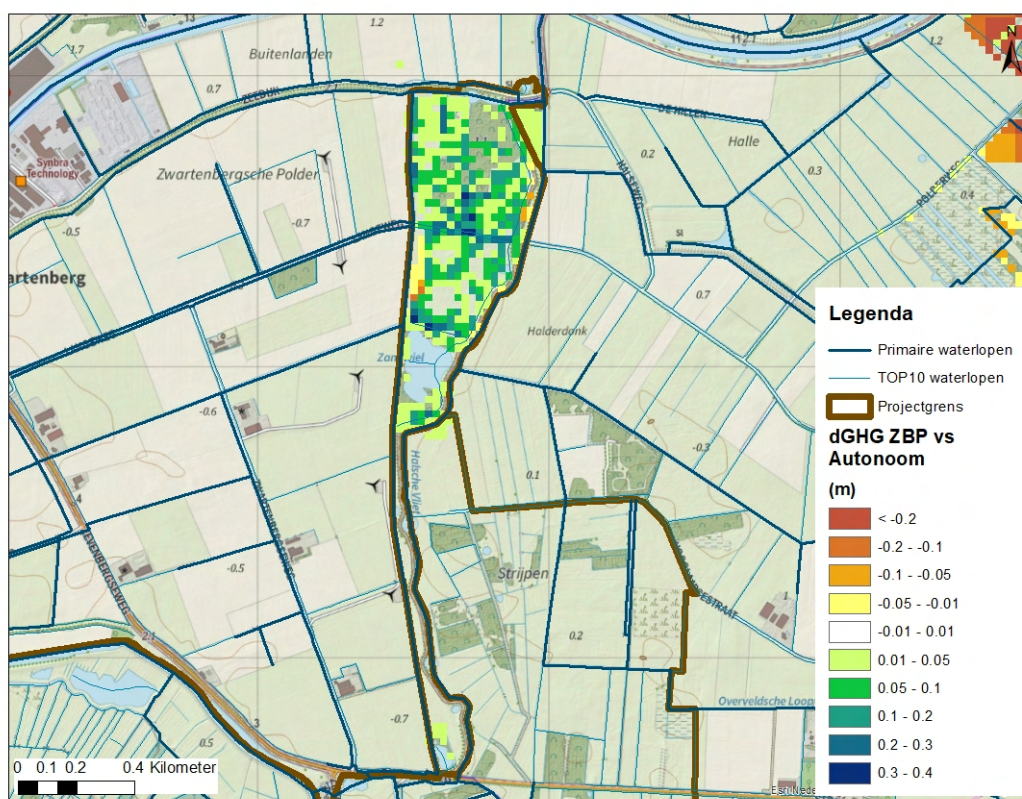
Figuur 7-5 Verschil in GHG tussen scenario Autonoom en scenario Zwartenbergse Polder.
