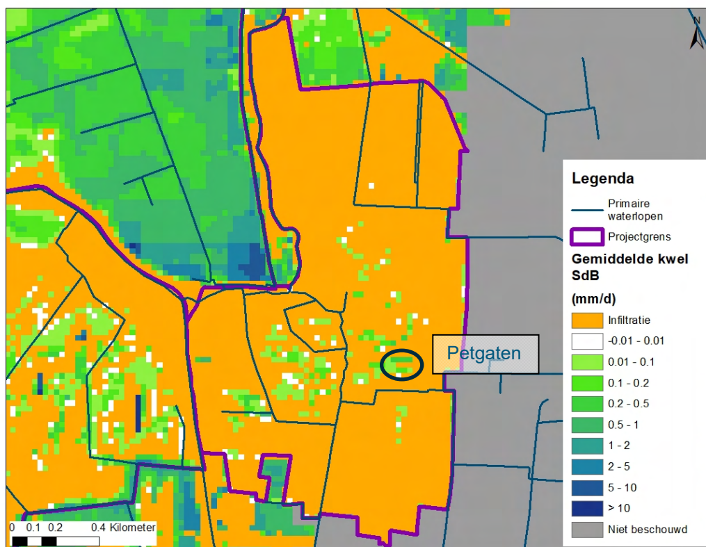
Figuur 9-12 Gemiddelde kwel in het scenario Strippen de Berk.
