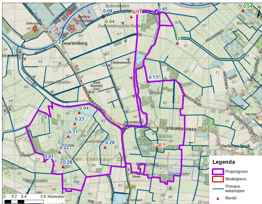
Figuur 5-2 Afwijkingen (m) van het basismodel in het 1 ste watervoerende pakket ten opzichte van metingen (model-meting). Blauwe cijfers betekent dat het model te hoge stijghoogten berekent, rood te lage stijghoogten en groen zit tussen de +0.05 en -0.05 cm verschil.
