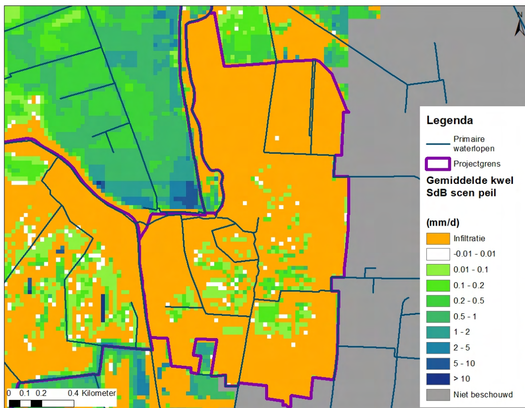
Figuur 9-28 Gemiddelde kwel in het extra scenario aanpassing peilen Stripen de Berk.
