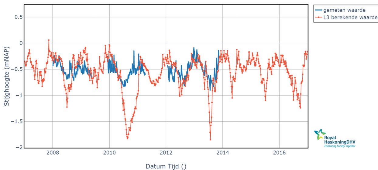
Figuur 5-3 Grafiek van model (rode lijn) en meting (blauwe lijn) voor peilbuis 6 (zie Figuur 4-4 voor de locatie van deze peilbuis).
