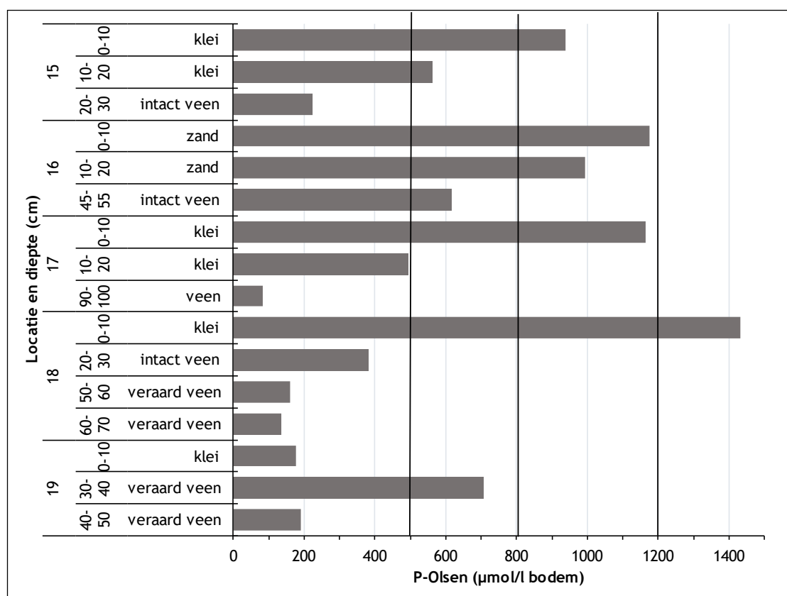
Figuur 24. De plantbeschikbare fosfaatconcentratie per bodemonster (in µmol/l bodem). De dikke verticale lijnen geven de randvoorwaarden van 500, 800 en 1200 µmol/l weer (tabel 2).
