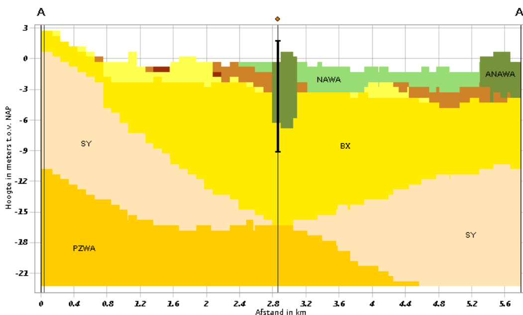
Figuur 2.3. Geo(hydro)logische doorsnede o.b.v. GEOTOP v1.4 ( www.dinoloket.nl ; mrt-2021) van Etten-Leur west via Kelsdok-Zwermlaken en de Zwartenbergese polder naar de Mark. PZWA = Peize&Waalre, SY= Stramproy, BX= Boxtel, NAWA = Naaldwijk-Walcheren, ANAW, Donkerbruin = Formatie van Nieuwkoop, Basisveen, Lichtbruin= Formatie van Nieuwkoop, Hollandveen.
