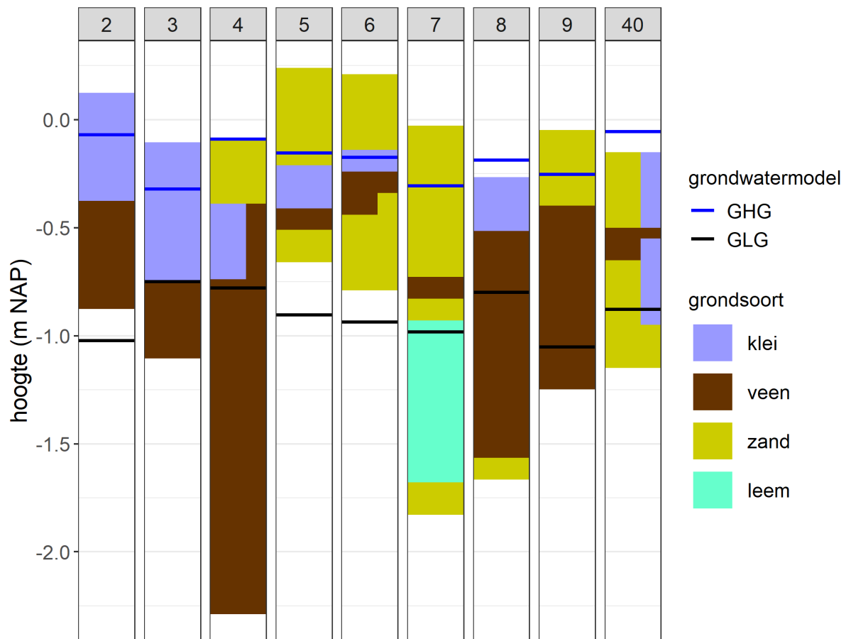
Figuur 14. Bodemprofielen van de onderzochte locaties. Maaiveldhoogte in meter +NAP.
