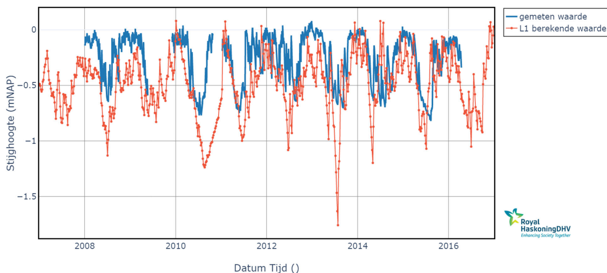
Figuur 5-23 Grafiek van model (rode lijn) en meting (blauwe lijn) voor peilbuis 1 (zie Figuur 4-4 voor de locatie van deze peilbuis).
