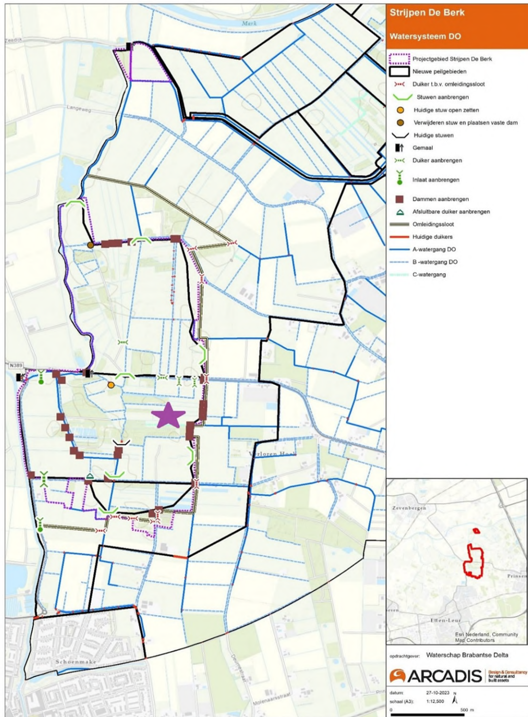
Figuur 7.6 Veranderingen ten gevolge van afgraving: bruine lijn is definitieve ligging omleidingssloot, deels in de vorm van een natuurvriendelijke oever. Verder wordt op één perceel een nieuw petgatcomplex aangelegd (paarse arcering) Bron: Arcadis, 2023, aangepast door TAUW
