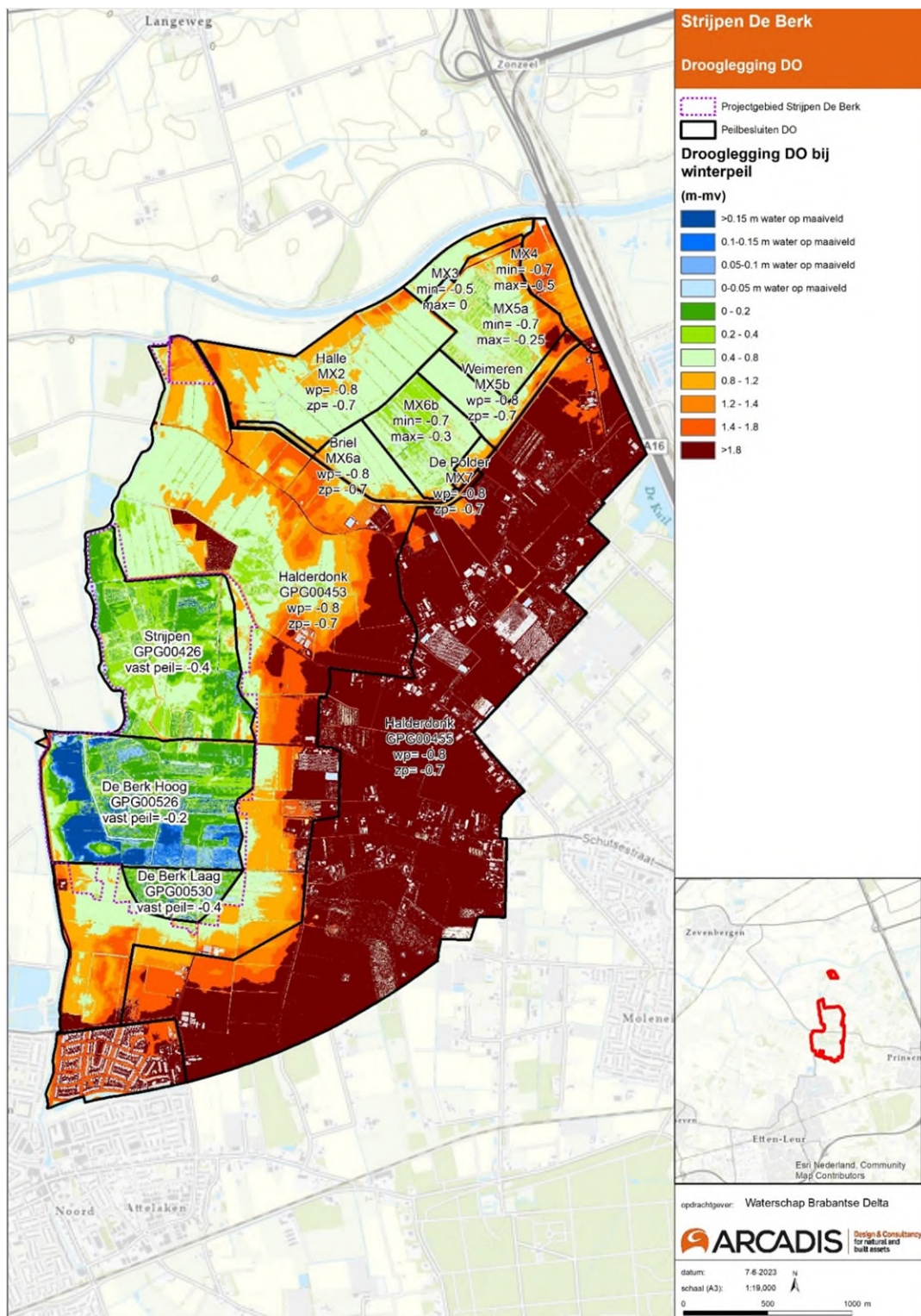
Figuur 7.12 Toekomstige drooglegging, bij vast/winterpeil in het gebied
