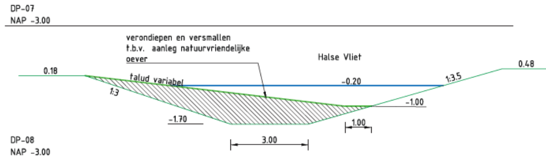
Figuur 4.3: ter illustratie het beoogde dwarsprofiel van de natuurvriendelijke oever bij de Halsche Vliet, incl. de verondieping van dit gedeelte van deze watergang. De natuurvriendelijke oever bij de Hooglaarsestraat heeft een ander profiel.
