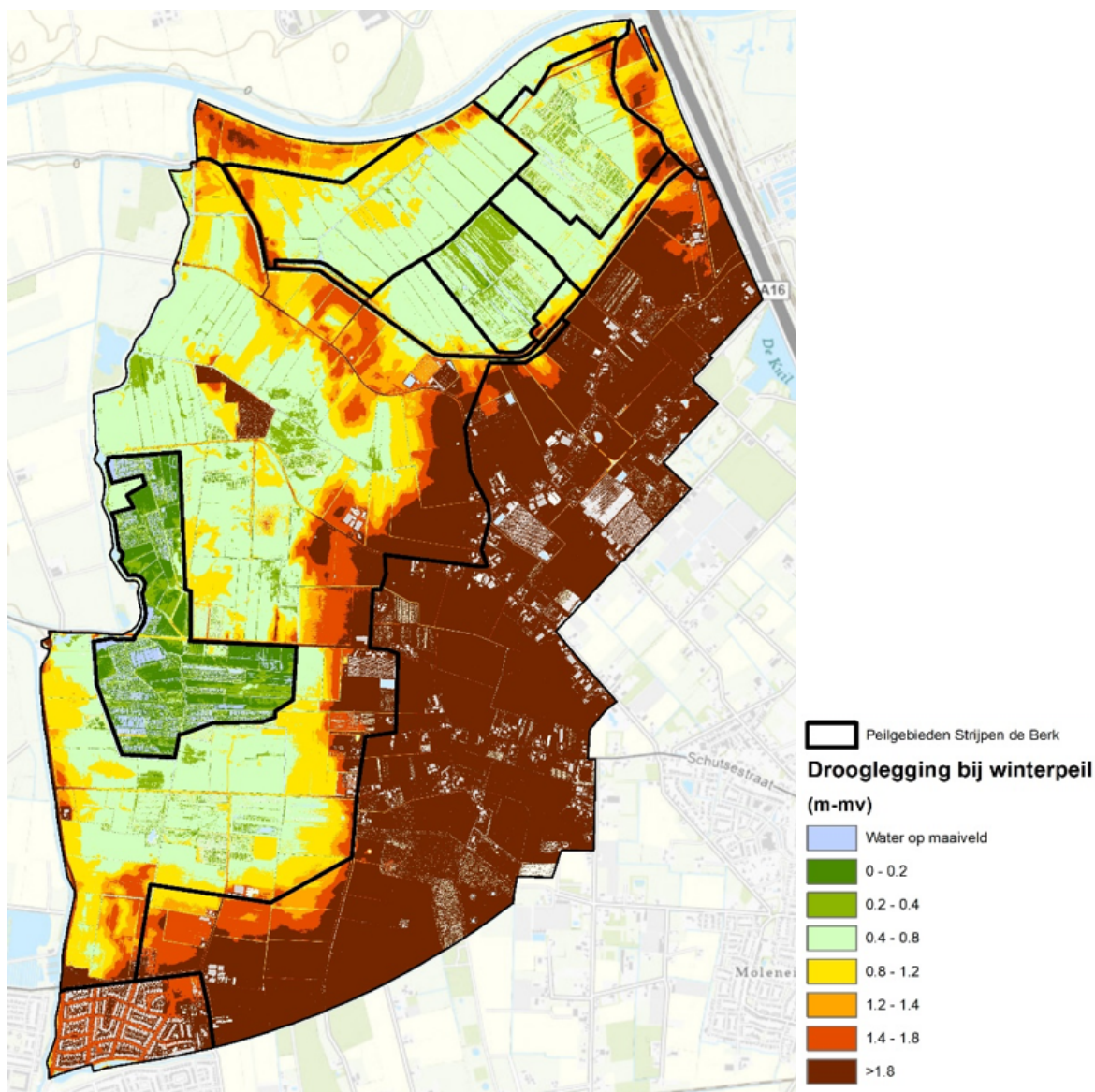
Figuur 7.3 Drooglegging bij de huidige praktijksituatie in plangebied Strijpen - de Berk en omgeving (bij winterpeil). Voor het peilgebied Strijpen- de Berk is uitgegaan van een max peil in de winter van -0,2 m NAP. (bron: Arcadis Onderbouwing Ontwerp integrale rapportage)
