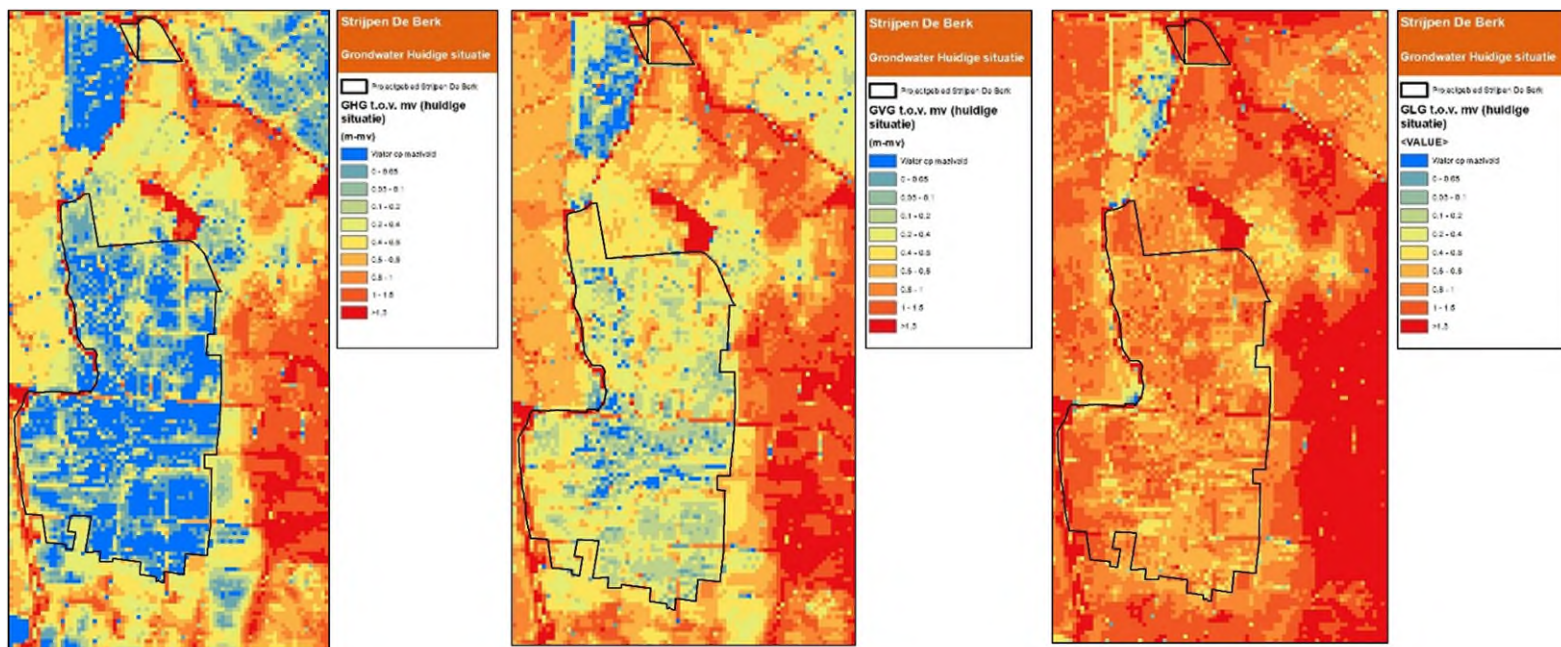
Figuur 7.10 Van links naar rechts: de verandering GHG, GVG en GLG door inrichtingsmaatregelen en peilaanpassingen (N.B. de effecten van peilopzet en verbetering infiltratie zijn afzonderlijk gemodelleerd en voor deze figuren samengenomen door ze op te tellen)
