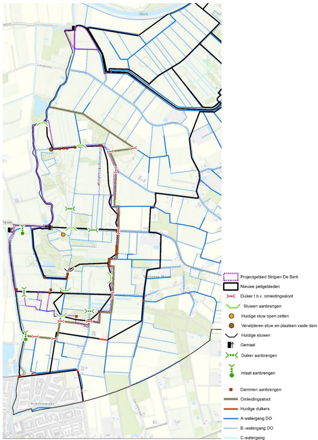
Figuur 4.2 Overzicht van het voorgestelde, nieuwe watersysteem in en rondom plangebied Strijpen/De Berk (Bron: Arcadis, Integrale rapportage)
