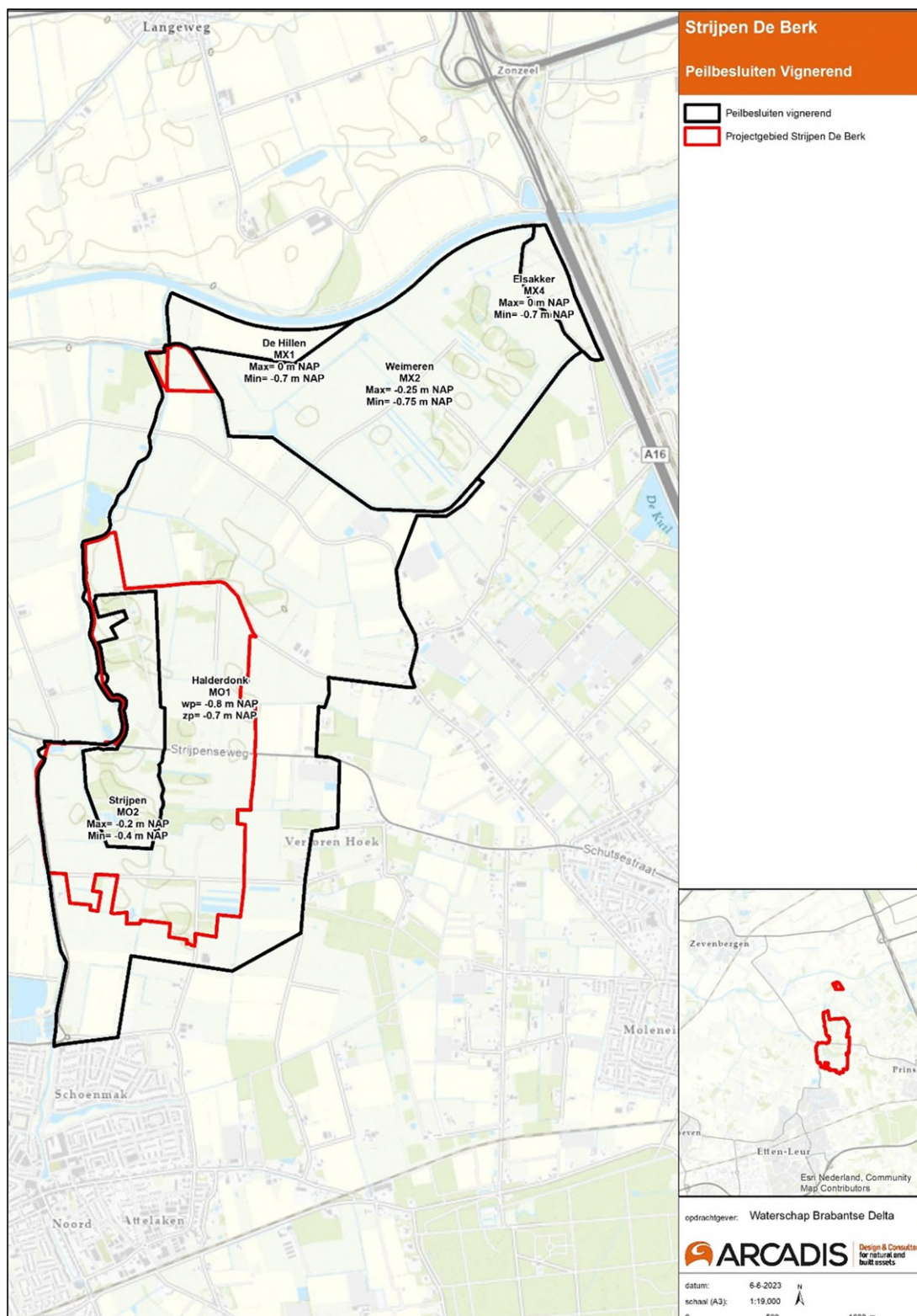
Figuur 7.2 Peilgebieden, ligging en peilen van peilgebied Strijpen/De Berk en omgeving. In rood het plangebied (geen peilgebied) (bron: Peilenplan Strijpen De Berk 2023)
