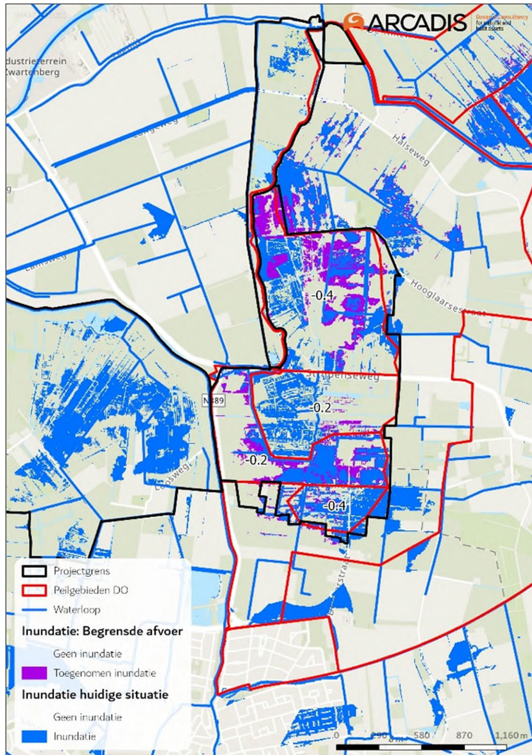
Figuur 7.9 Gevolgen van het plan op inundaties in en rond het plangebied
