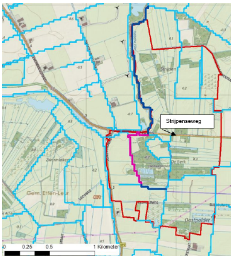
Figuur 7.8 Aanpassing peil Halse Vliet donkerblauwe en paarse lijntracé, paarse lijn geeft het gedeelte weer waar een kleilaag wordt aangebracht
