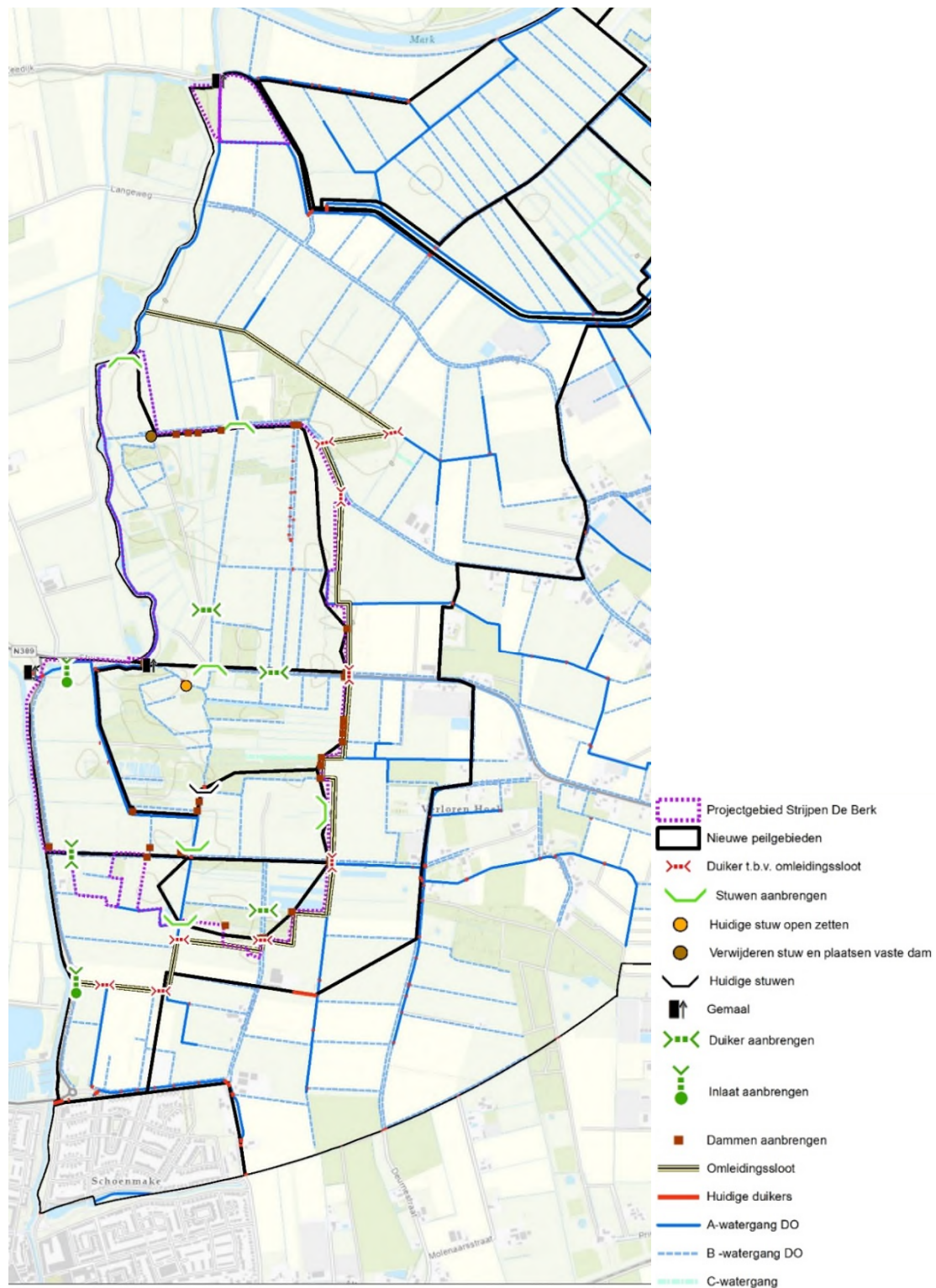
Figuur 0.5 Overzicht van het voorgestelde, nieuwe watersysteem in en rondom plangebied Strijpen/De Berk (Bron: Arcadis, Integrale rapportage)
