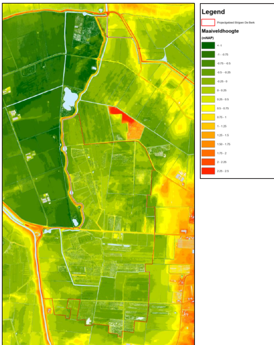
Figuur 2.1 Maaiveldhoogte in het projectgebied Strijpen/De Berk en omgeving (Bron: Projectplan Waterwet)
