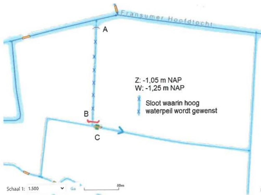
Figuur 1: Locatie van werkzaamheden. A: Vervangen stuw & locatie van de pomp op zonne-energie. B: Plaatsen keerwand. C: Bestaande dam voorzien van een duiker.
