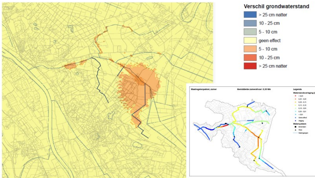
Figuur 3-2. Effecten tijdens een zomersituatie (inzet: effect oppervlaktewater). Geel: minder dan 5 cm verlaging, licht oranje: 5-10 cm verlaging en donkeroranje: 10-25 cm verlaging.
