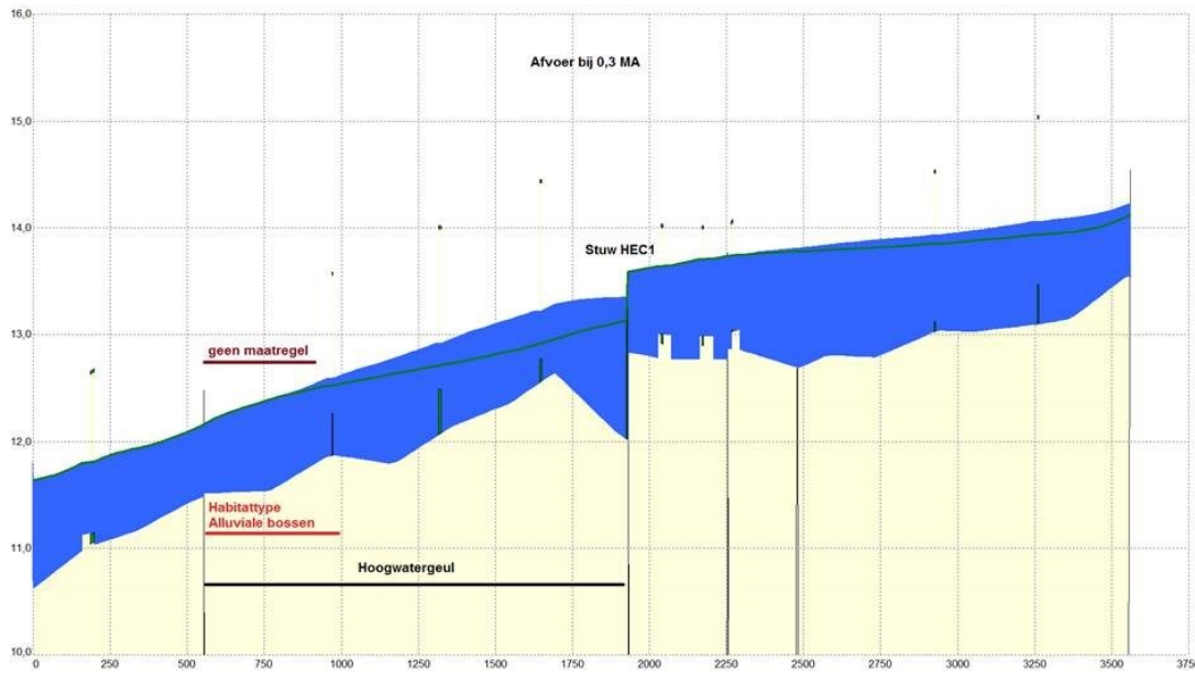
Figuur 2-3. Effect maatregelenpakket op oppervlaktewaterstand, waarbij de laatste 300 m het oude profiel van de hoogwatergeul is laten zitten. In blauw: waterstand huidig, groene lijn: waterstand met gewijzigde maatregel.
