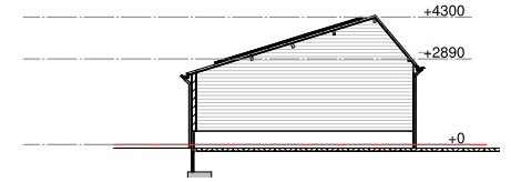
Doorsnede C-C
