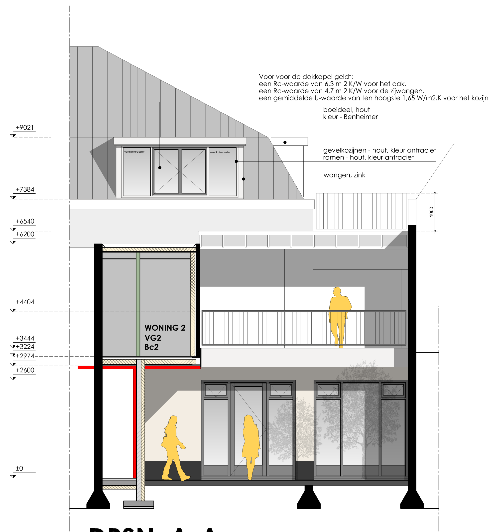
DRSN A-A nieuwe toestand
