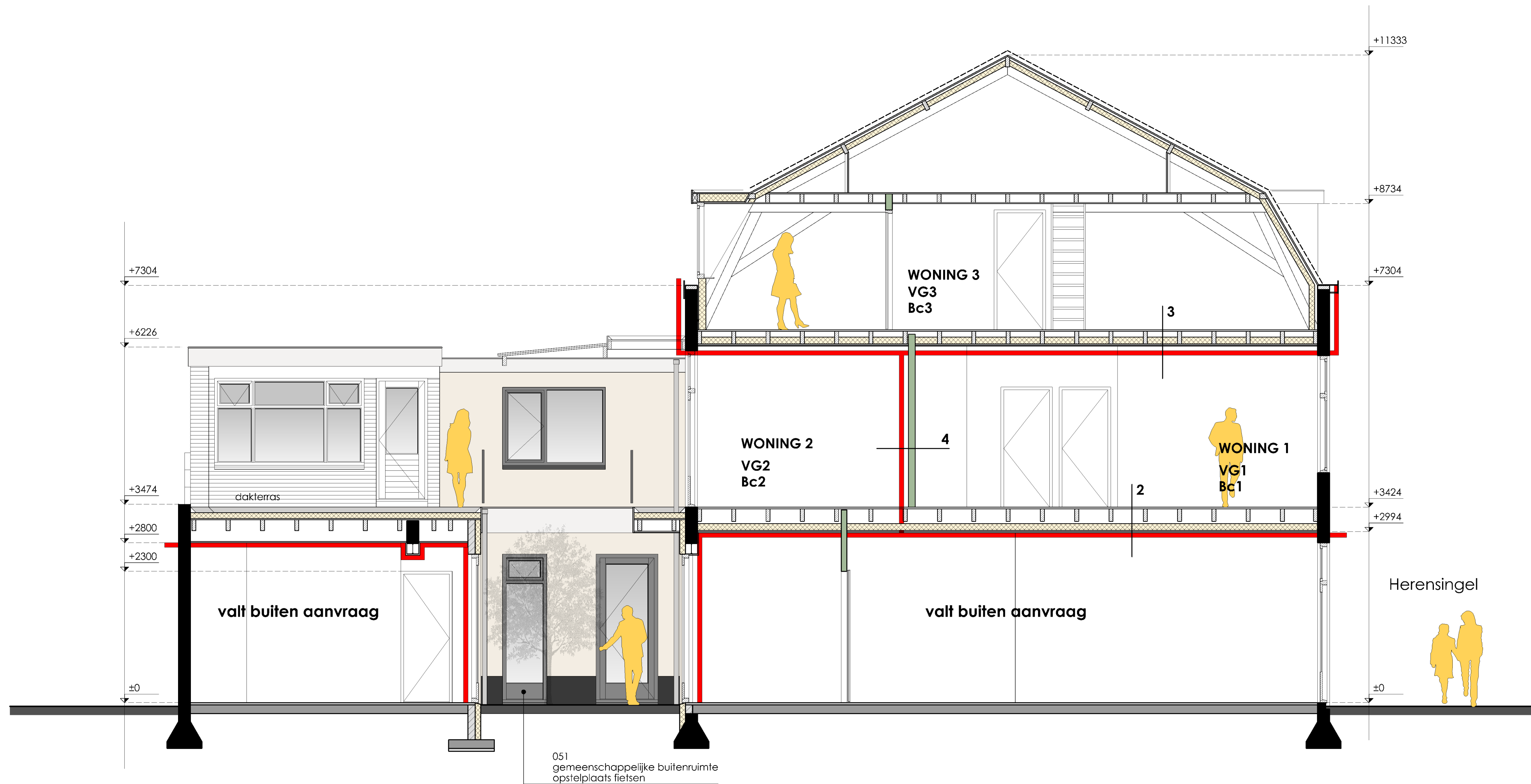
DRSN C-C nieuwe toestand
