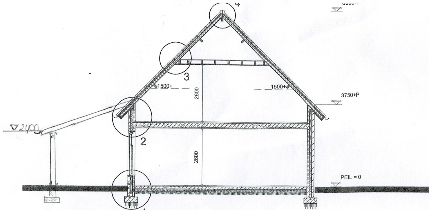
DOORSNEDE A-A
