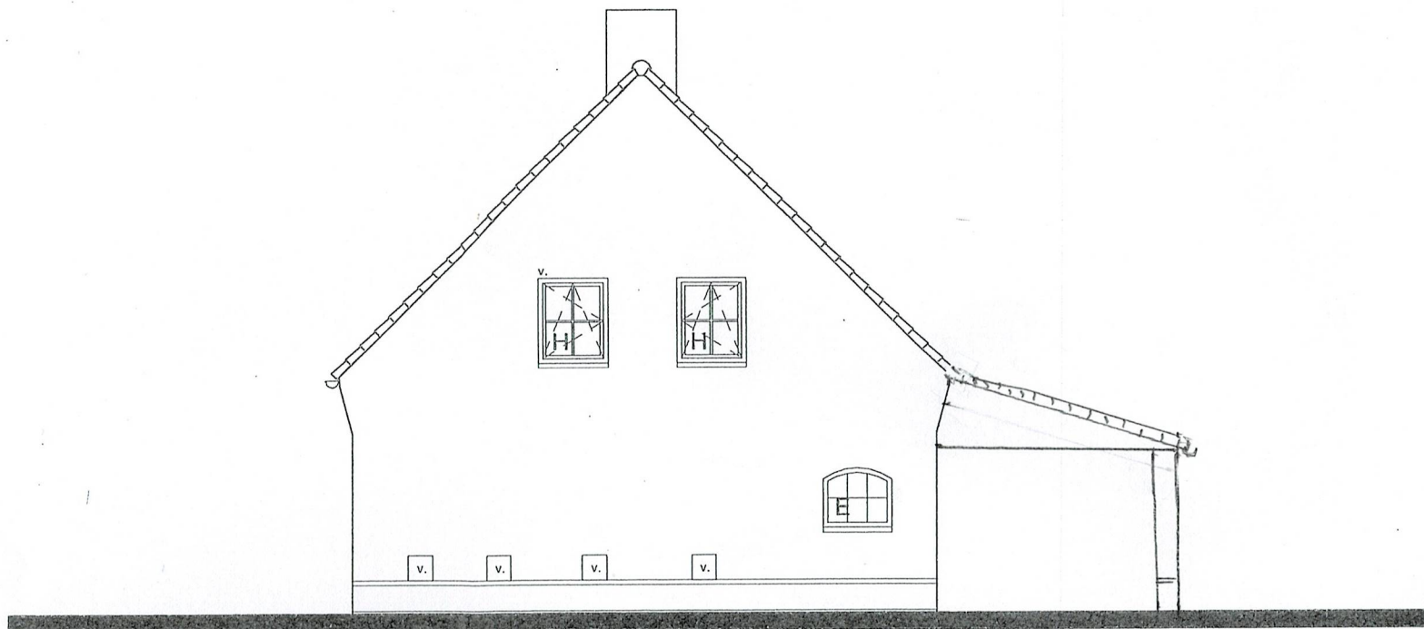
RECHTER ZIJGEVEL
