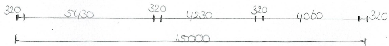
ACHTERGEVEL
