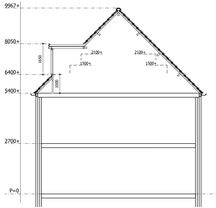
GEWIJZIGDE DOORSNEDE
