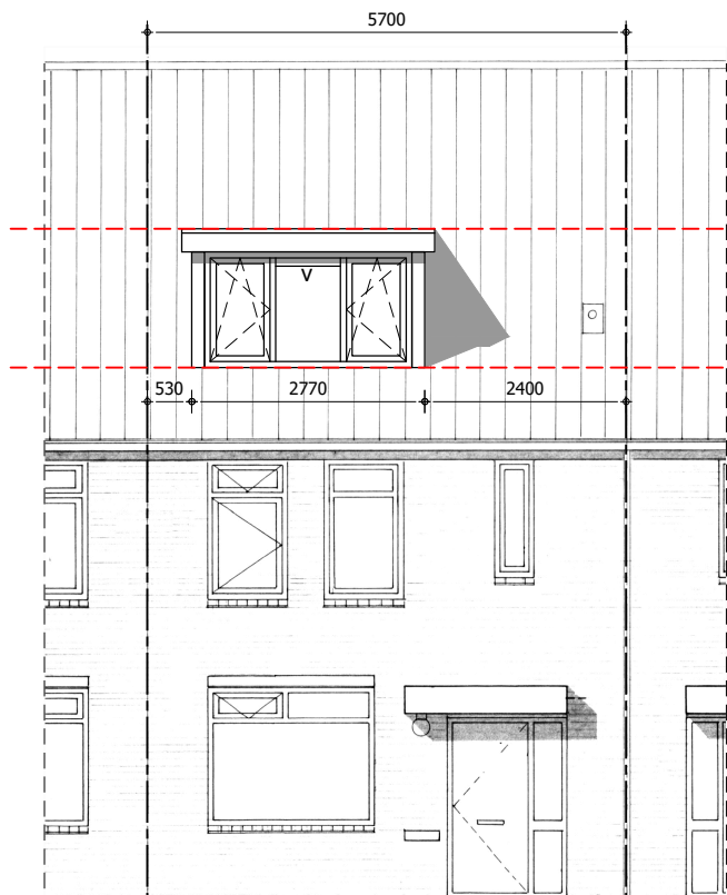
GEWIJZIGDE VOORGEVEL v = ventilatierooster nom. gemiddelde capaciteit bij 1 Pascal van 22,6 l/s.
