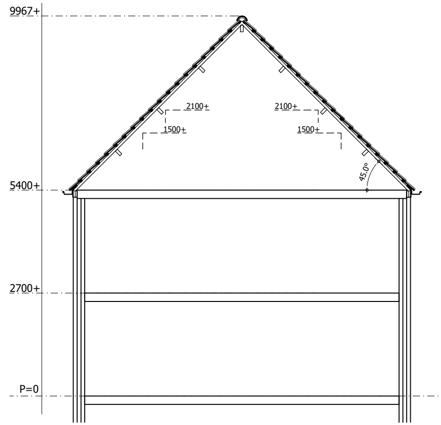
BESTAANDE DOORSNEDE
