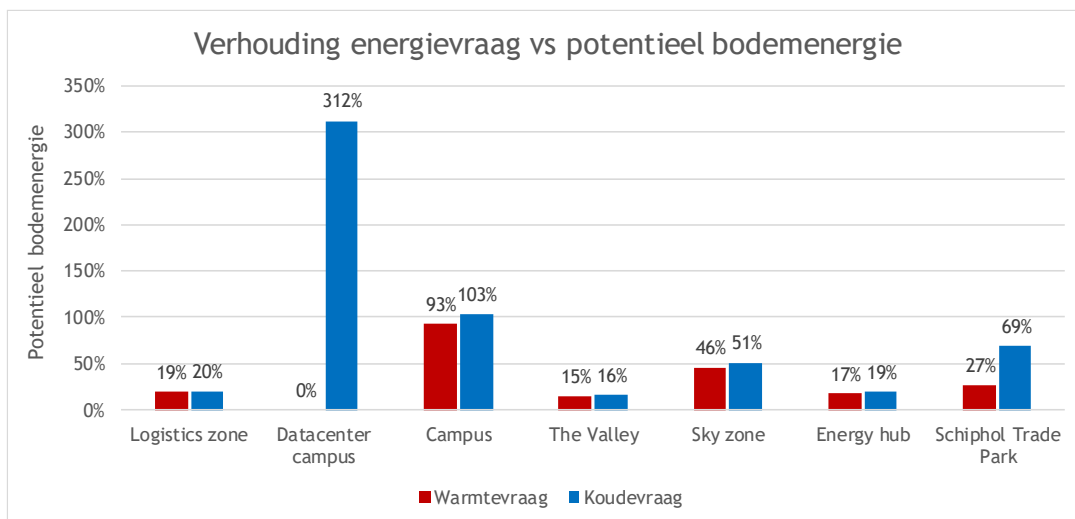
Figuur 4.4 | Energievraag tegenover beschikbaar bodempotentieel
