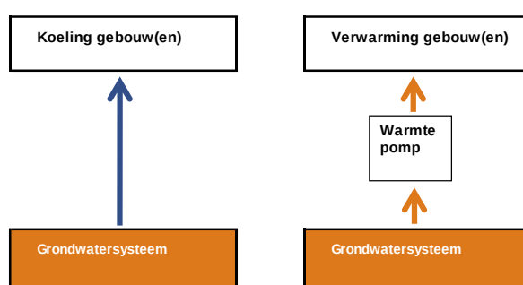
Figuur 4.3 | Principe energieconcept WKO
