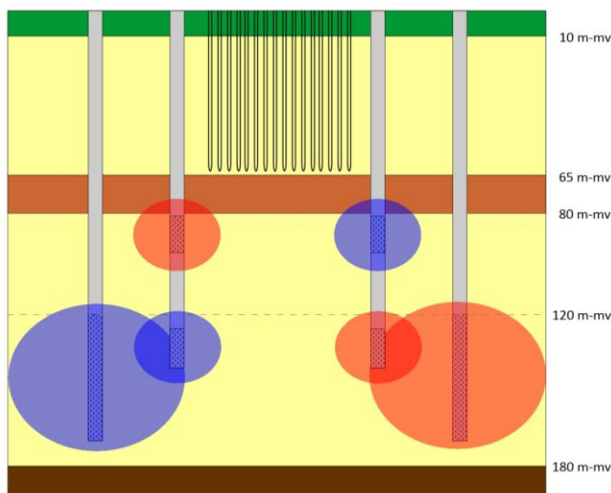
Figuur 4.5 | Schematische weergave diepteligging verschillende type systemen
