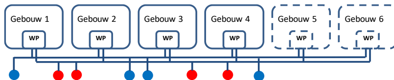
Figuur 1.4 | Collectief WKO systeem
